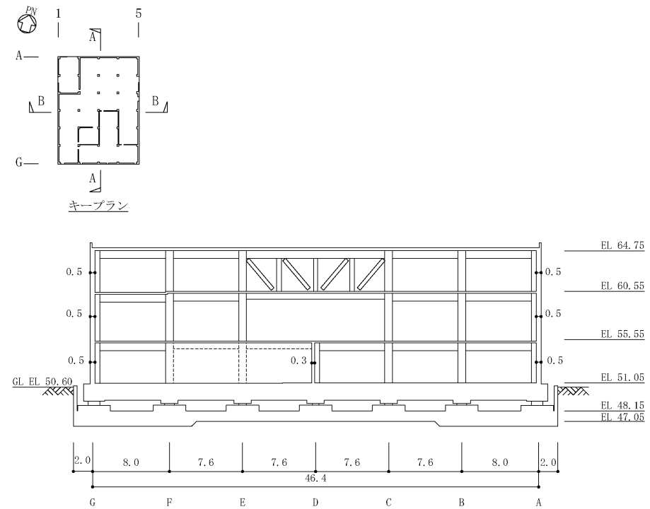
A-A断面 (3通り) 断面図 (Y方向)
