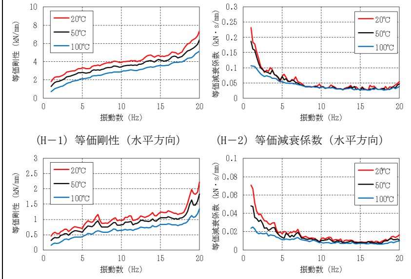
(H-1) 等価剛性 (水平方向) (H-2) 等価減衰係数 (水平方向) (V-1) 等価剛性 (鉛直方向) (V-2) 等価減衰係数 (鉛直方向) 第3-6-5添図 粘性体温度による減衰性能への影響確認結果
