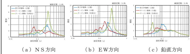
第3-21図 床応答スペクトル
