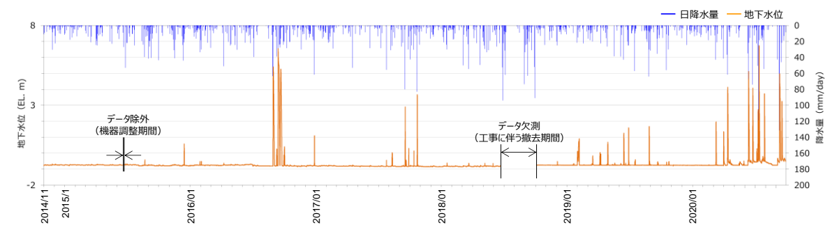
補足 9-2(6)図 地下水位観測記録 (No. 6 孔)
