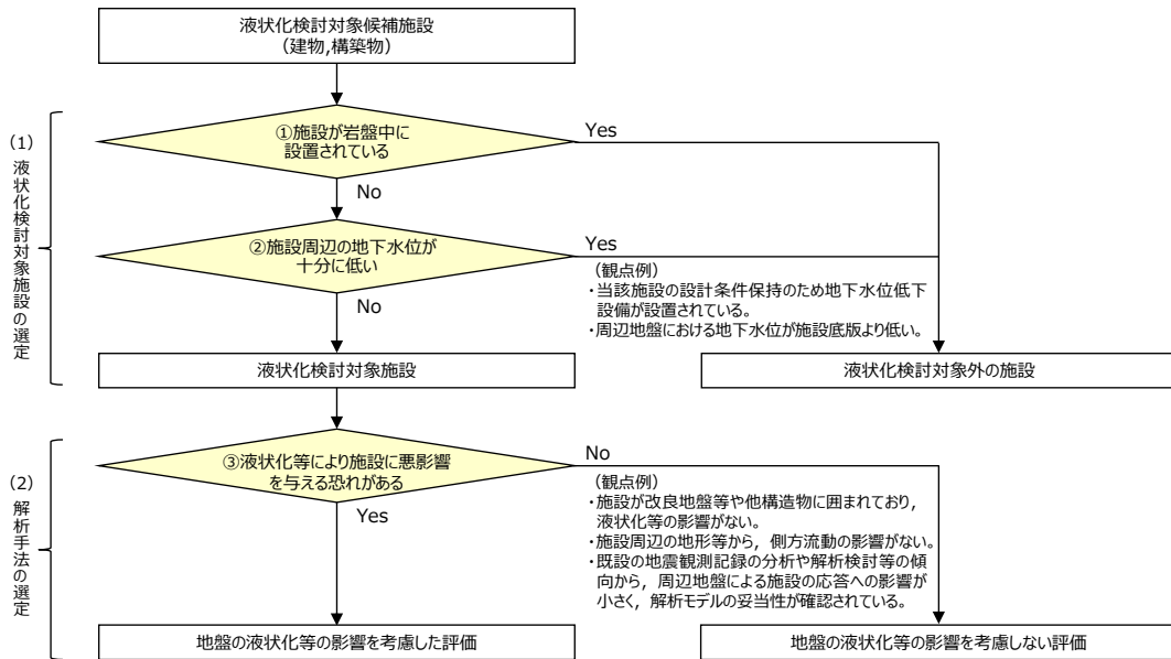
第4-2-2 図(1) 液状化検討対象施設の選定及び解析手法 選定フロー（建物、構築物）
