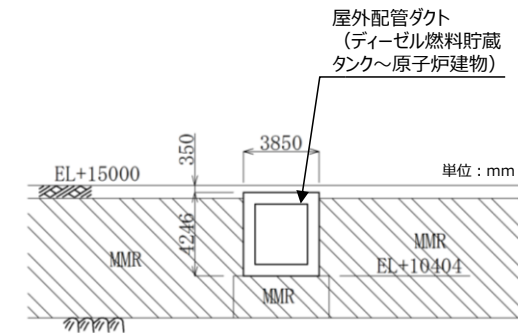
第6-2-79図 屋外配管ダクト (ディーゼル燃料貯蔵タンク~原子炉建物) 断面図 (4-4)断面)
