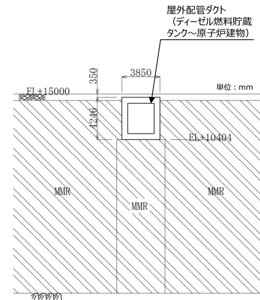
第6-2-80図 屋外配管ダクト (ディーゼル燃料貯蔵タンク~原子炉建物) 断面図 (5-5)断面)
