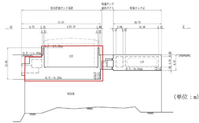
別添6-63図 復水貯蔵タンク基礎断面図 (A-A)
