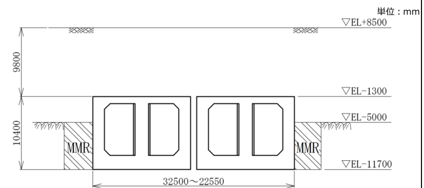
第6-2-10図 取水槽 断面図 (④-④断面)
