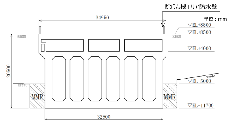
第6-2-9図 取水槽 断面図 (③-③断面)
