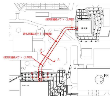
別添6-16図 排気筒連絡ダクト掘削図
