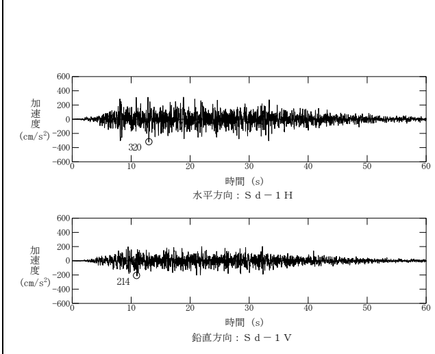
第 1.4-8 図 弾性設計用地震動 S d - 1 の設計用模擬地震波の加速度時刻歴波形
