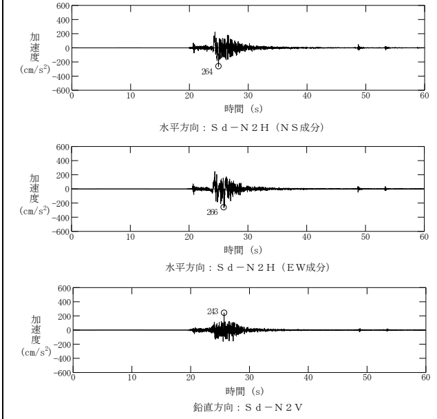
第 1.4-7 図 弾性設計用地震動 S d - N 2 の速度時刻歴波形
