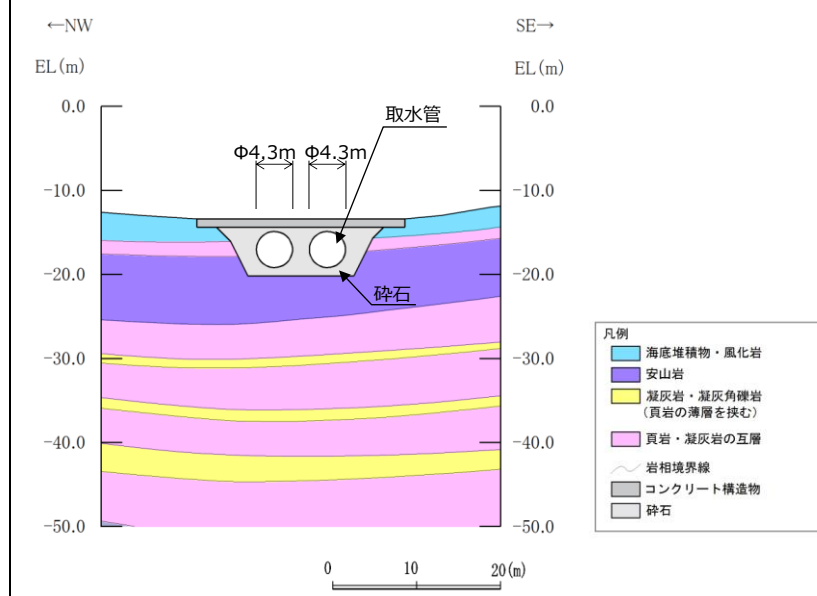
第6-2-122図 取水管 地質断面図 (④-④断面)
