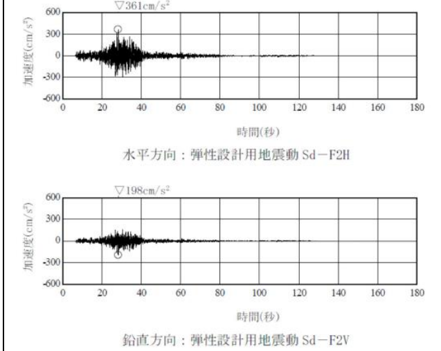
第 1.4.1-6 図 弾性設計用地震動 S d - F 2 の加速度時刻歴波形
