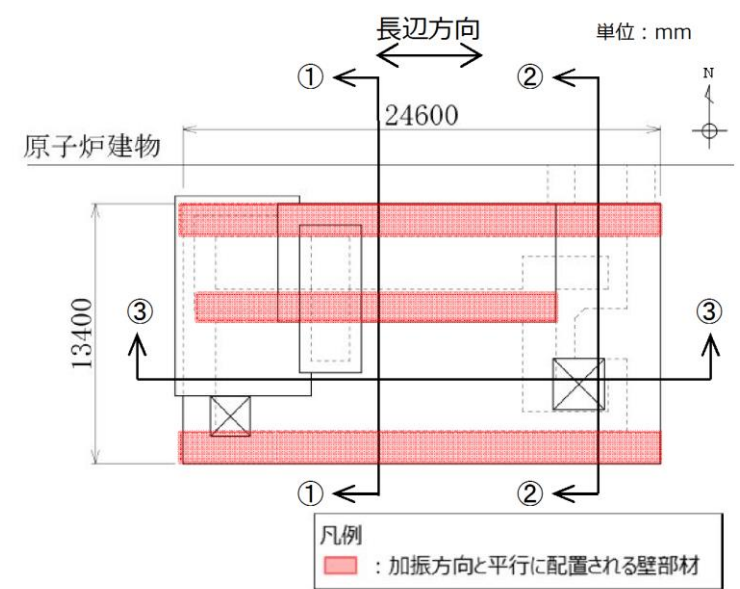
第6-2-37図 第1ベントフィルタ格納槽 平面図
