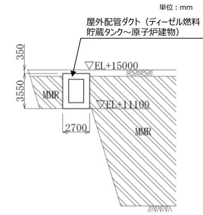
第6-2-78図 屋外配管ダクト (ディーゼル燃料貯蔵タンク~原子炉建物) 断面図 (2-2)断面)
