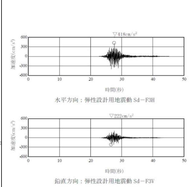
第 1.4.1-7 図 弾性設計用地震動 S d - F 3 の加速度時刻歴波形
