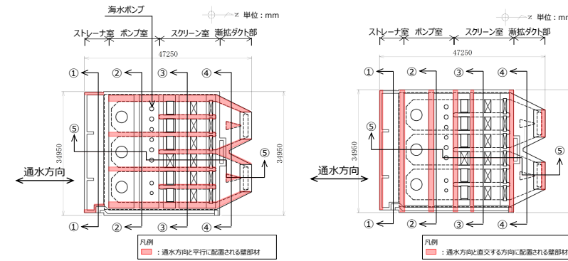
第6-2-5図 取水槽 平面図
