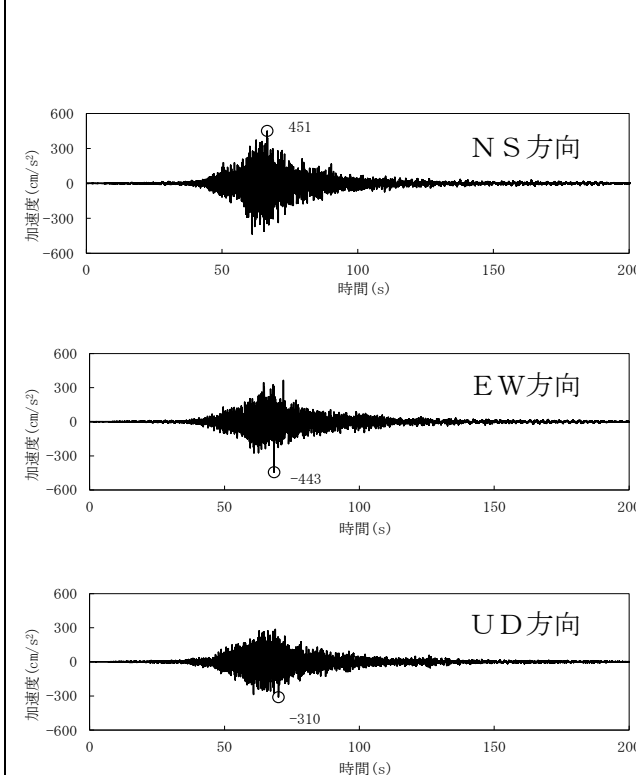
第 1.3-9 図 弾性設計用地震動 S d - 2 1 の時刻歴波形
