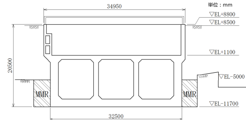
第6-2-8図 取水槽 断面図 (②-②断面)
