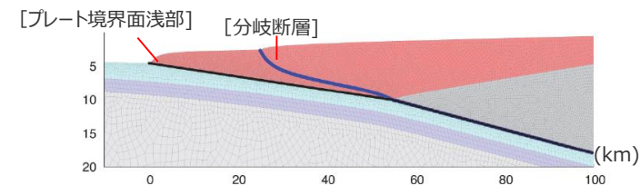
プレート境界モデルおよび分岐断層モデル (奥村・後藤(2013)を基に作成)
