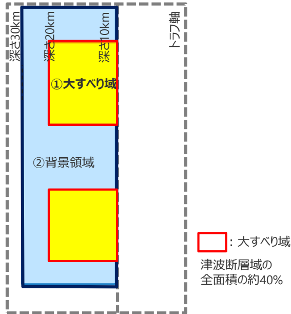
プレート沈み込み速度を考慮したモデルの すべり分布概念図
