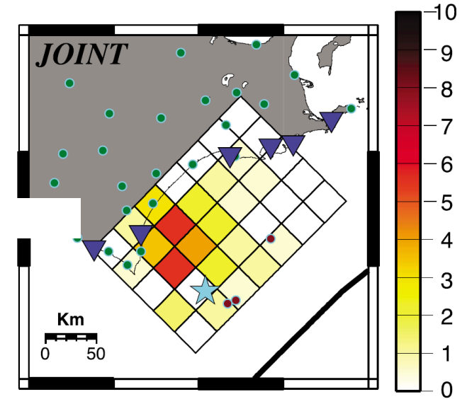
Romano et al.(2010)による波源モデル
