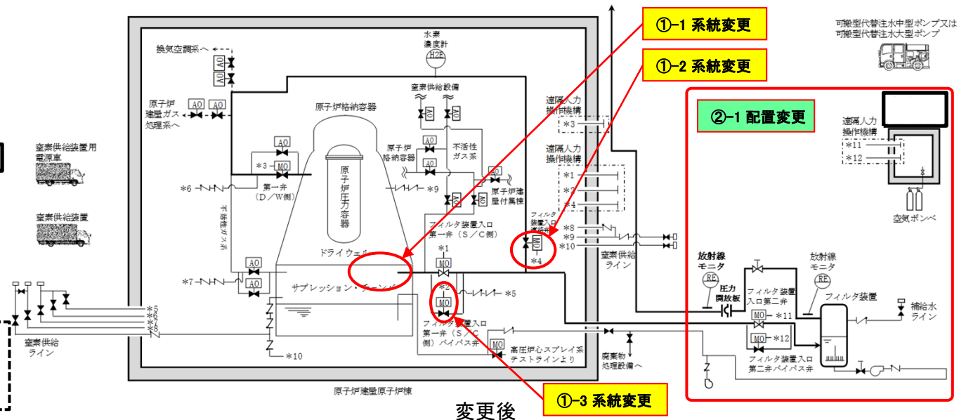
第5図 FV系統概要図
