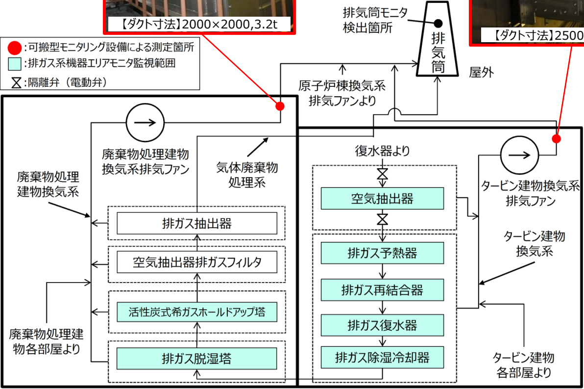
系統概要及び可搬型モニタリング設備測定箇所例
