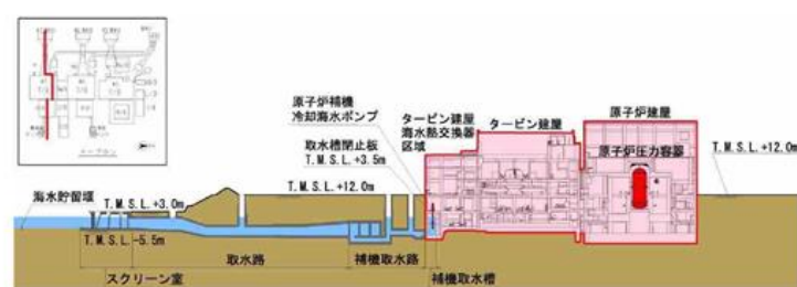
補機取水路断面
