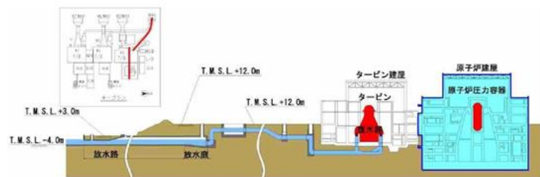
放水路断面
