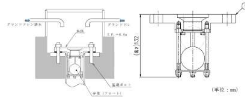
第 2.2-30 図 緊急用海水ポンプグランド dren 排出口逆止弁構造図
