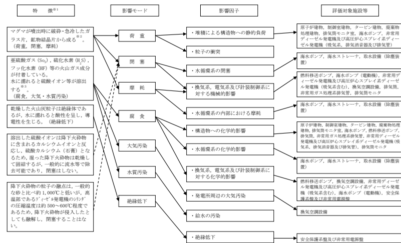
第2-1図 降下火砕物の特徴と影響因子
