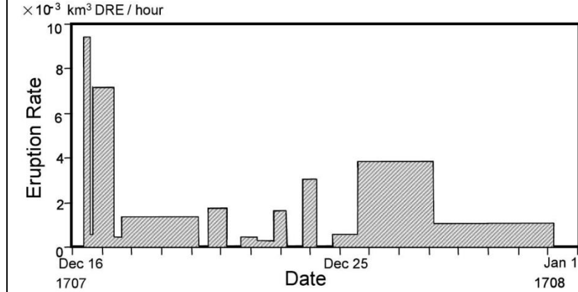
第15-1図 富士山（宝永噴火1707年）の噴出率の推移（宮地・小山（2007））
