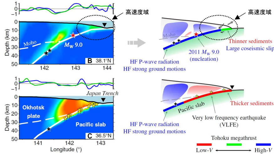
プレート境界におけるP波速度分布とそのイメージ(p159再掲) (Liu and Zhao(2018)に一部加筆)
