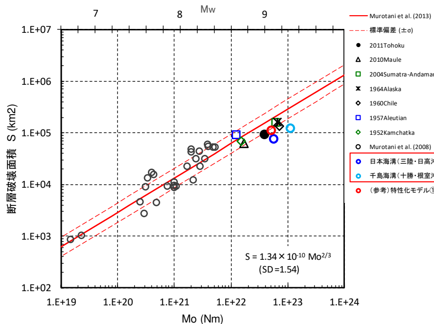
破壊領域(S)とM 0 の関係※ (Murotani et al.(2013)一部修正・加筆)
