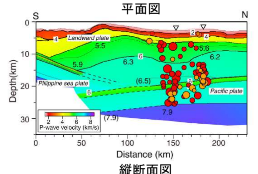
3.11地震の余震分布(3月12日-19日)とプレート境界面の位置関係 (Shinohara et al.(2011))
