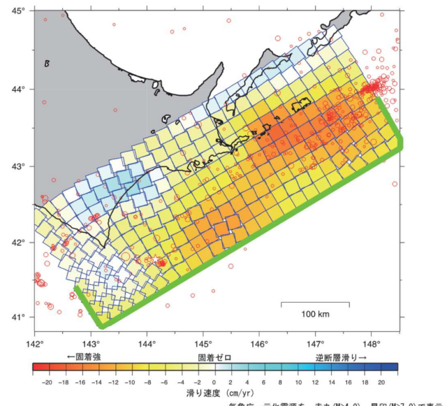
気象庁一元化震源を, 赤丸(M s 4.0), 黒印(M s 7.0)で表示.
