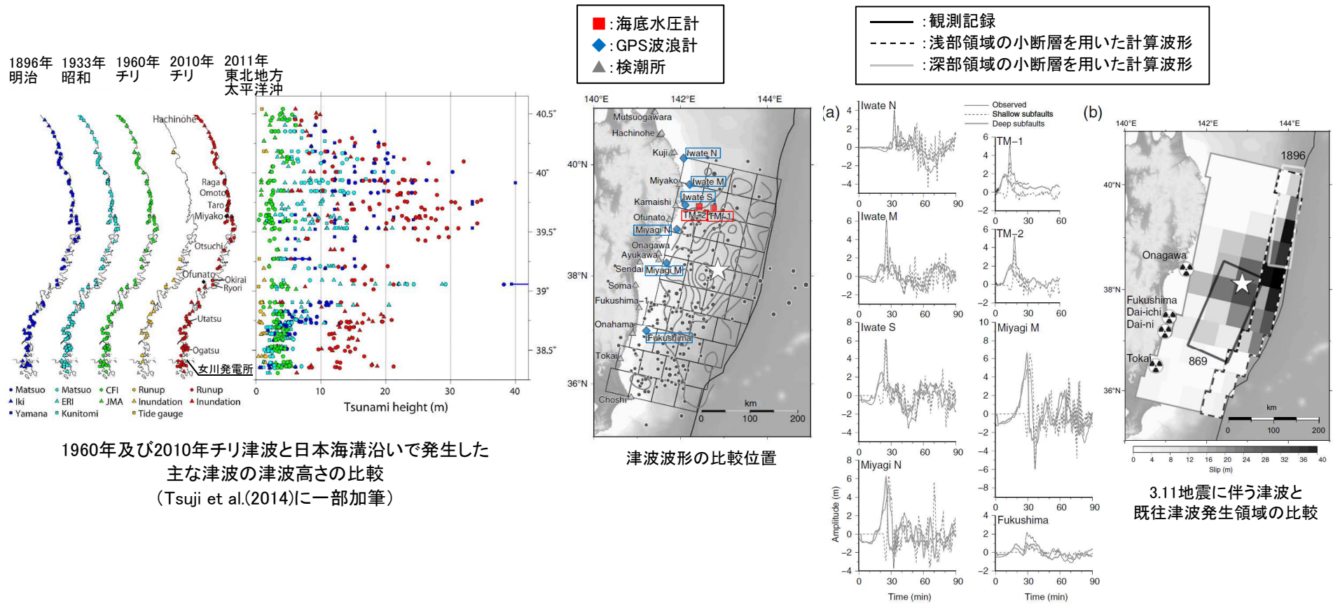
観測波形と計算波形の比較
