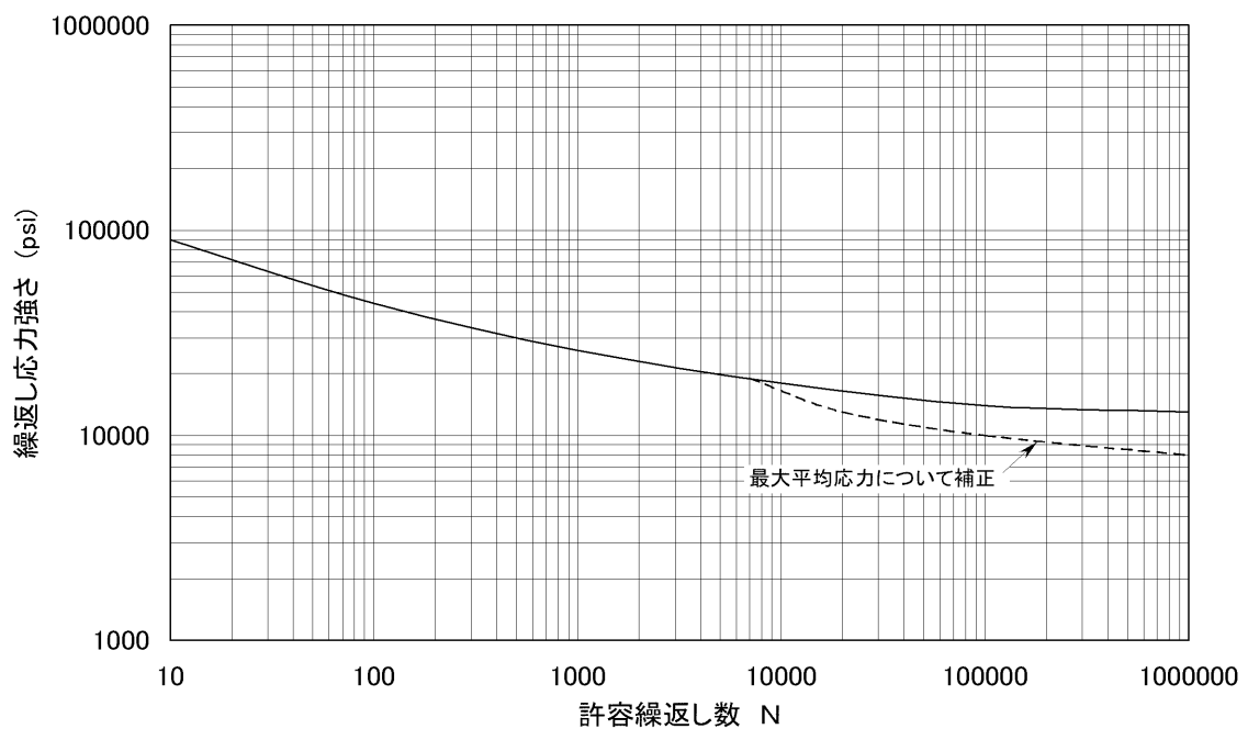
第3-10図 NDA 被覆管の設計疲労曲線 (注2)
