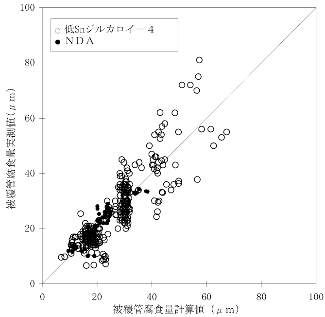
第 3-14 図 被覆管腐食量（最大酸化膜厚）の実測値と予測値の比較
