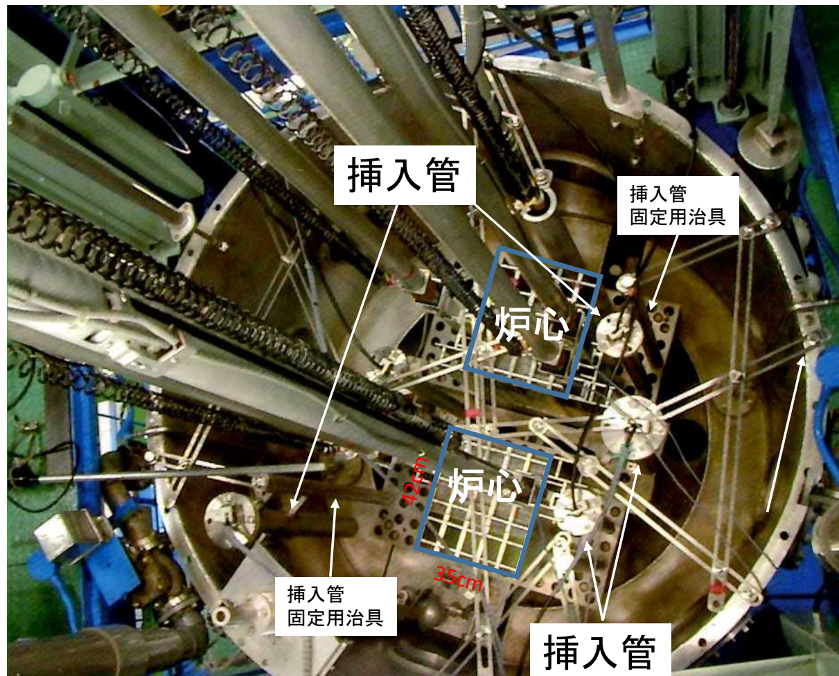
軽水減速炉心(2分割炉心)における挿入管の使用方法
