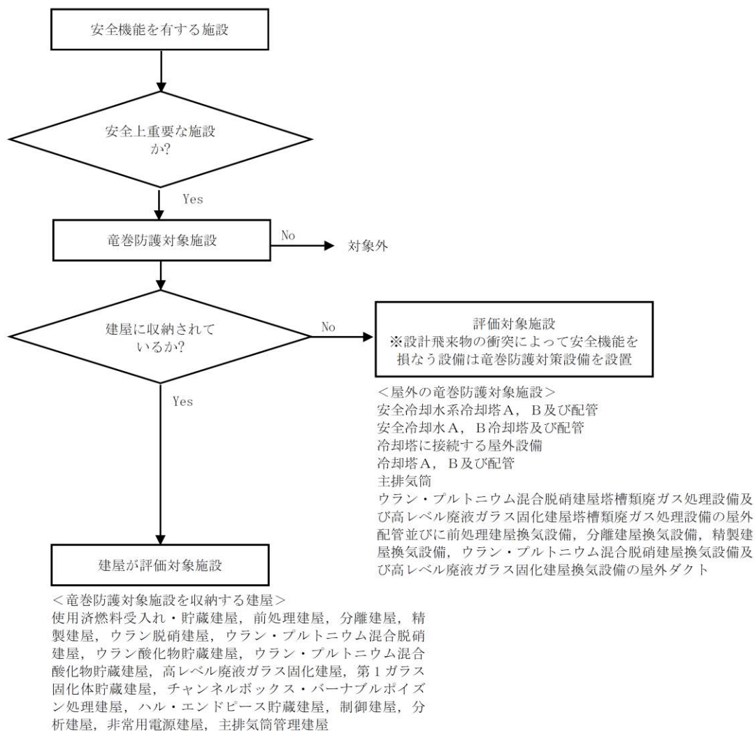
第 3 図 飛来物に対する評価対象施設の選定フロー
