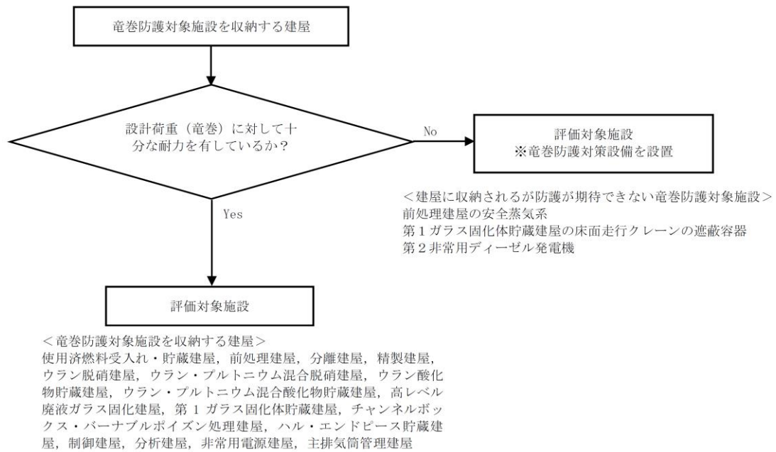
第4図 建屋の耐力に関する評価対象施設の選定フロー
