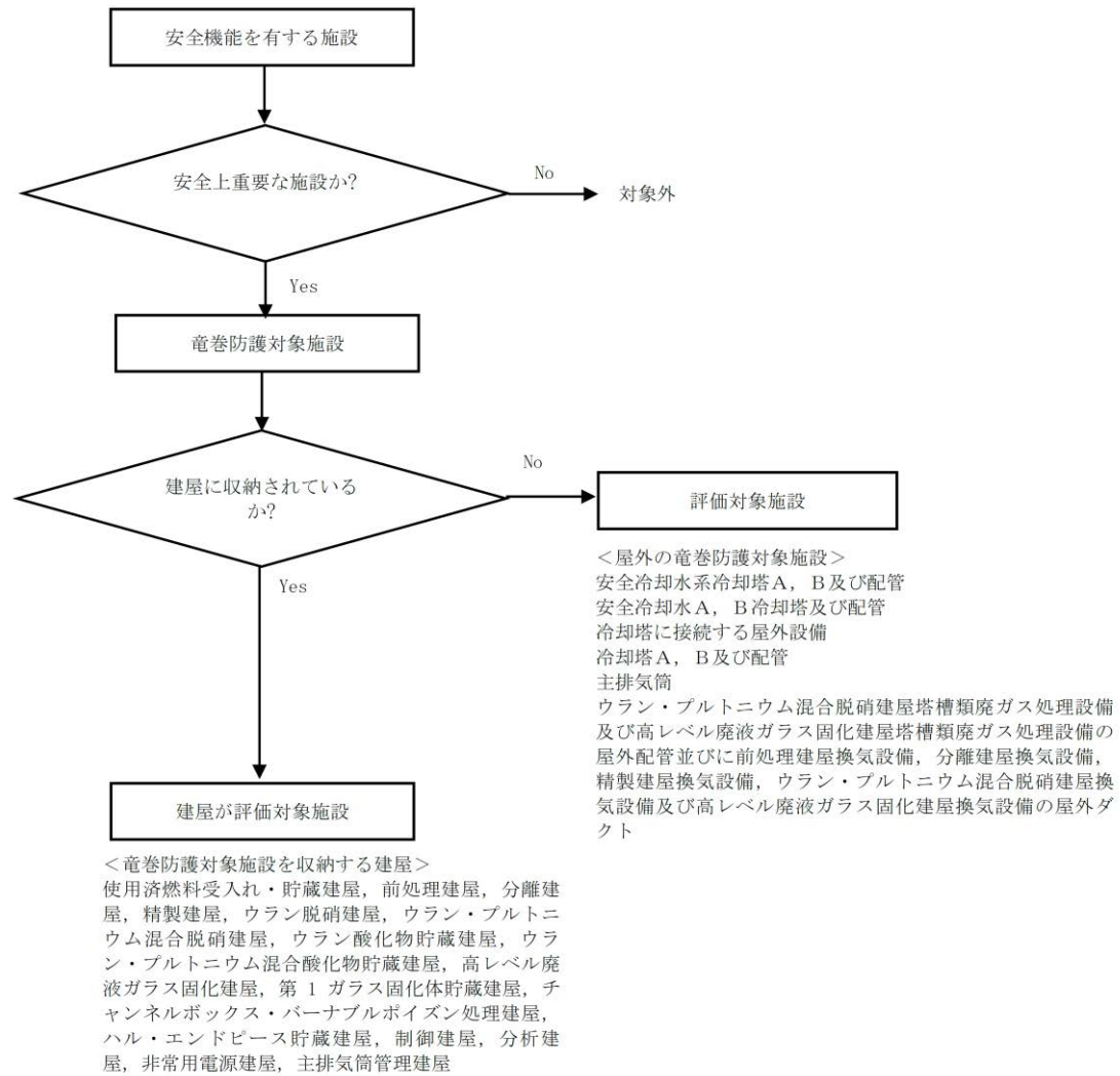
第 1 図 風圧力に対する評価対象施設の選定フロー
