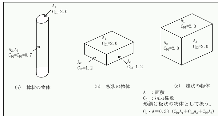
第1図 抗力係数
