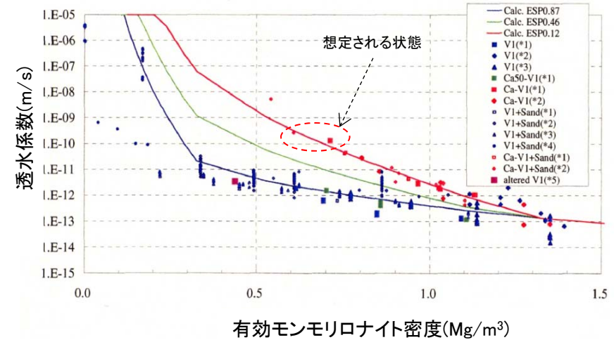
有効モンモリロナイト密度とベントナイト系材料の透水性の関係
