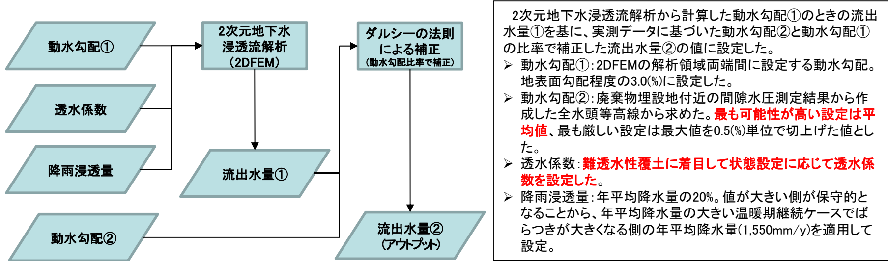
埋設設備からの流出水量に係るパラメータの関係
