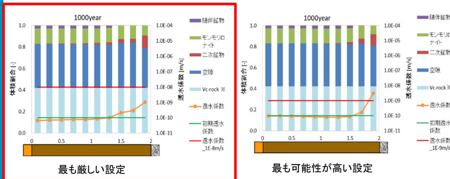
3号廃棄物埋設地の難透水性覆土における鉱物組成と透水性の分布図(1,000年後)
