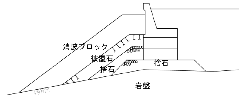
第5図 護岸の構造概要
