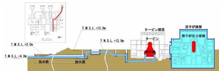
放水路断面
