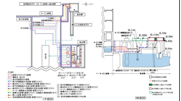
第1.5-13図 バウンダリ機能を保持するポンプ、配管及び隔離弁（電動弁、逆止弁）の設置箇所の概要
