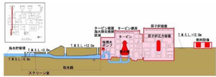
取水路断面
