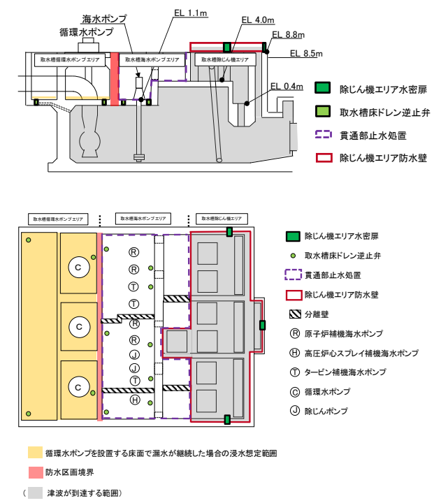
第1.5-12図 防水区画化範囲
