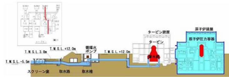
取水路断面
