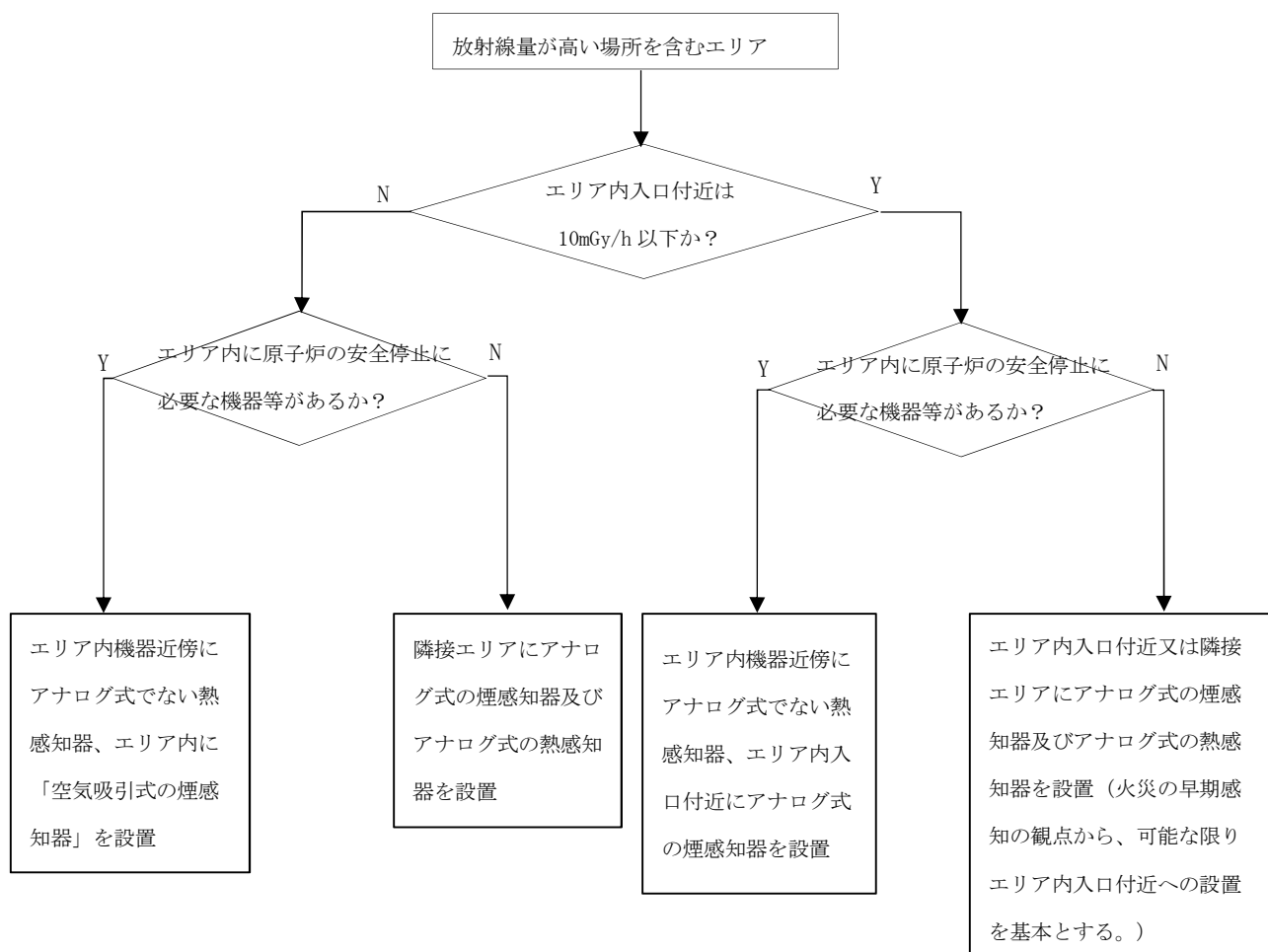
第 3-6-4 図 放射線量が高い場所を含むエリアにおける火災感知器の設置場所の条件を整理したフロー
