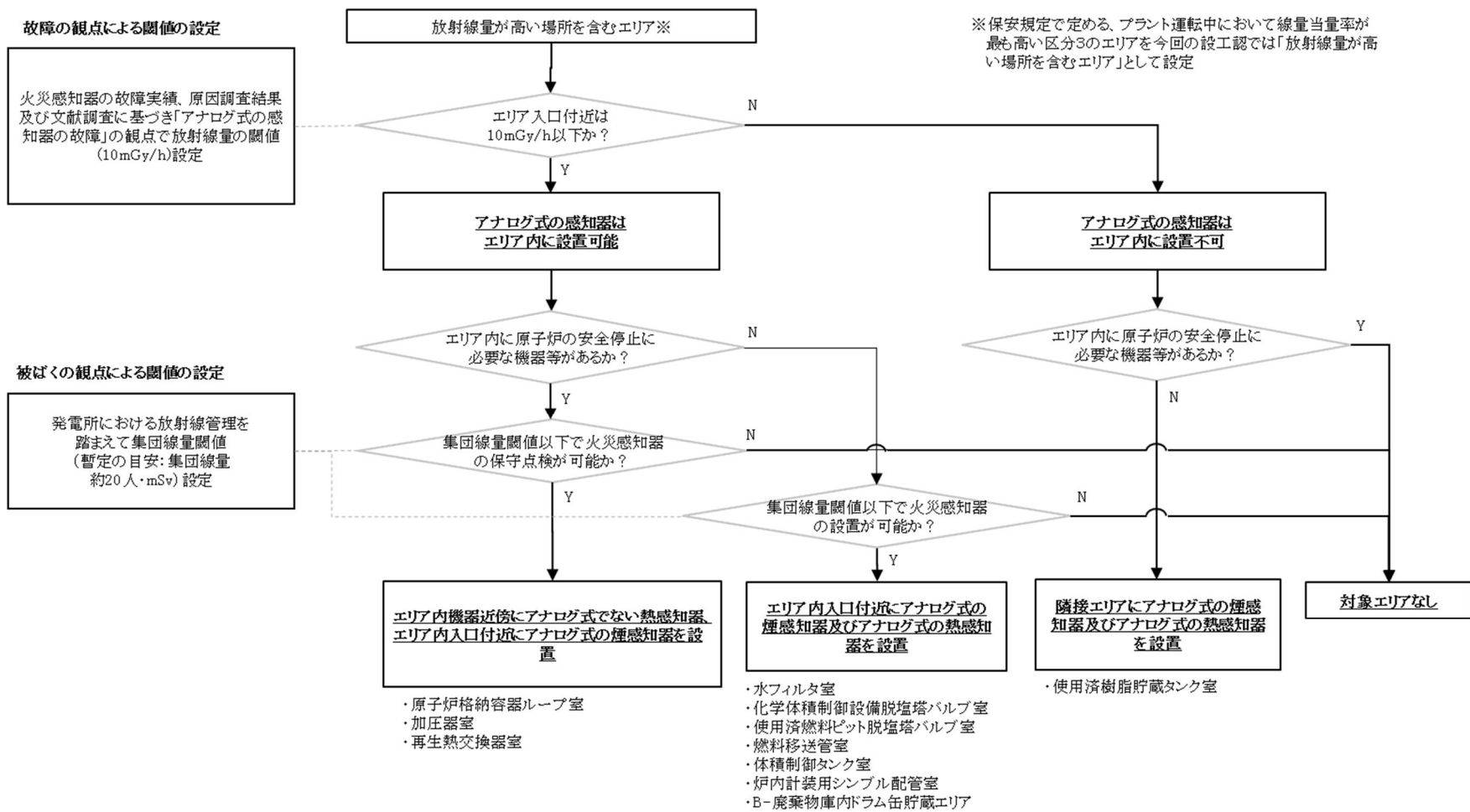
第 3-6-5 図 放射線量が高い場所を含むエリアの火災感知器設計フロー
