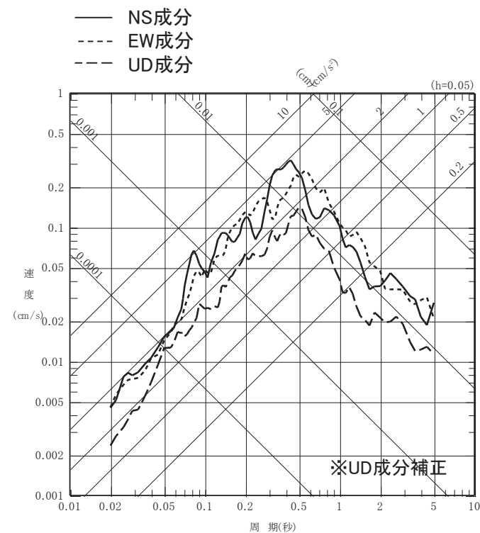
応答スペクトル
