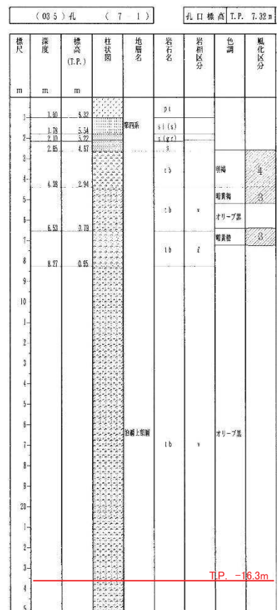
地質柱状図及びピコア写真
