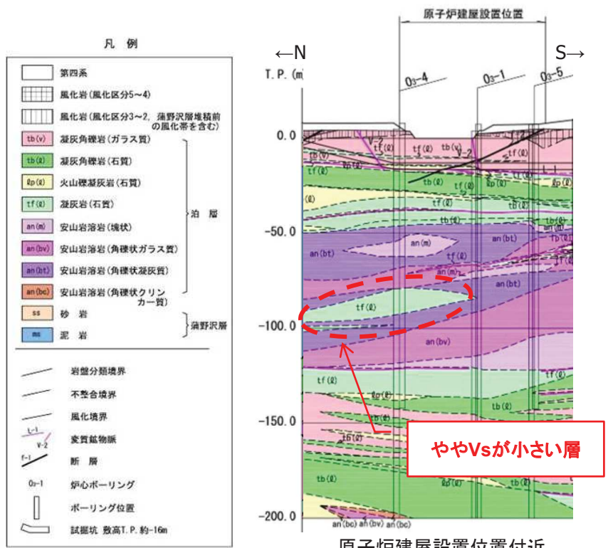
原子炉建屋設置位置 における地質鉛直断面図
