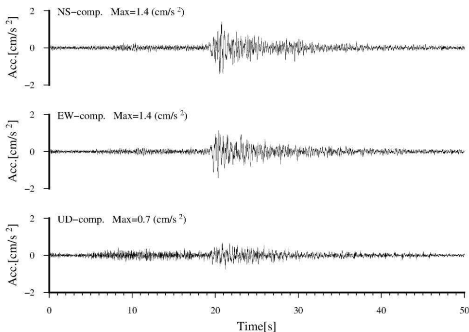
加速度波形
