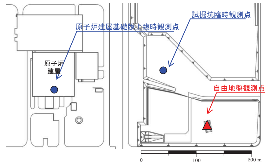
検討に用いた地震観測点
