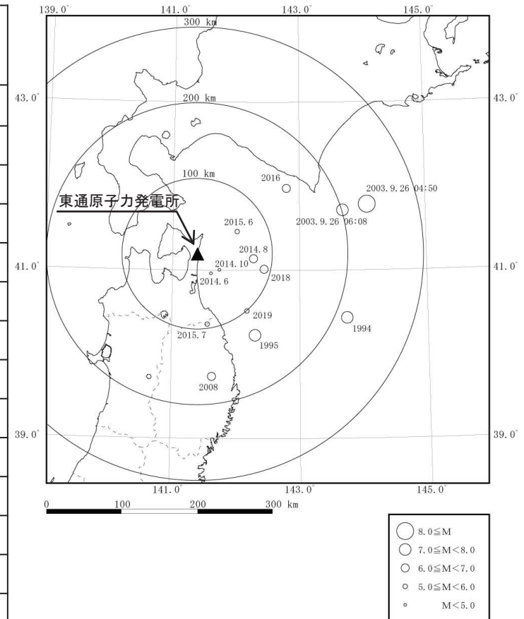
震央分布図
