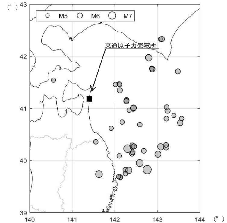
震央分布
