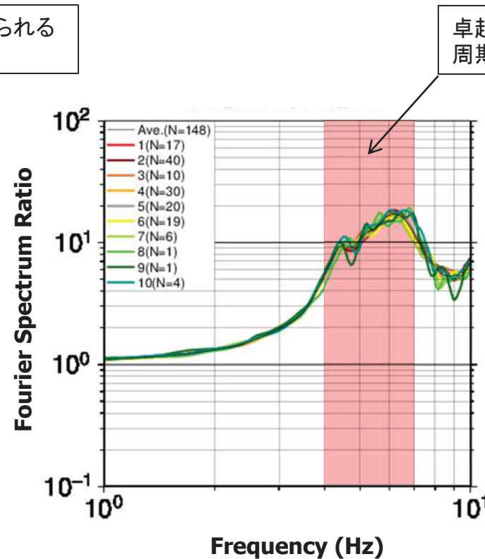
基準化スペクトルB No.13観測点*/試掘坑の岩盤上観測点
