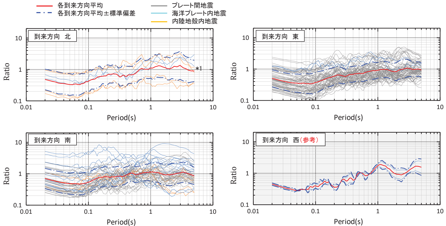
観測記録とNoda et al.(2002)との比較 地震波到来方向別 水平成分 自由地盤の岩盤上部地震観測点 (T.P.+2.0m) / Noda et al.(2002)
