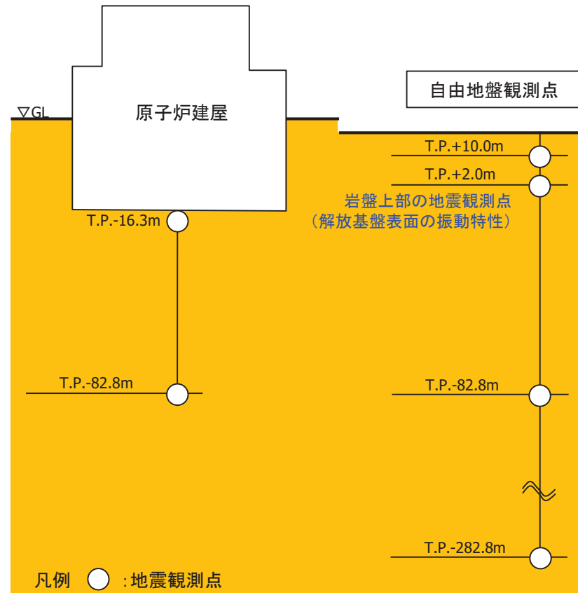
敷地内地盤系の地震観測点
