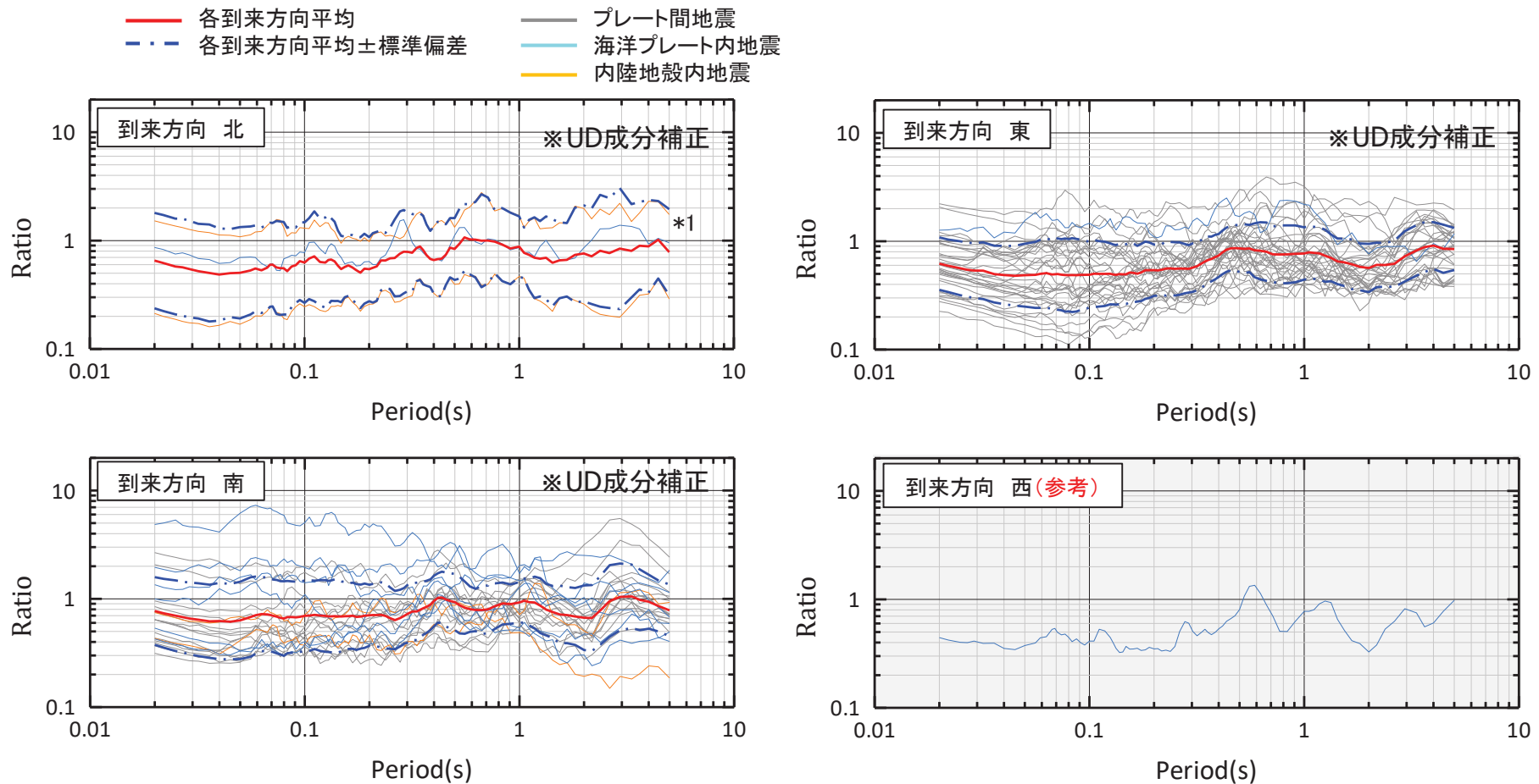
観測記録とNoda et al.(2002)との比較 地震波到来方向別 鉛直成分 自由地盤の岩盤上部地震観測点 (T.P.+2.0m) / Noda et al.(2002)
