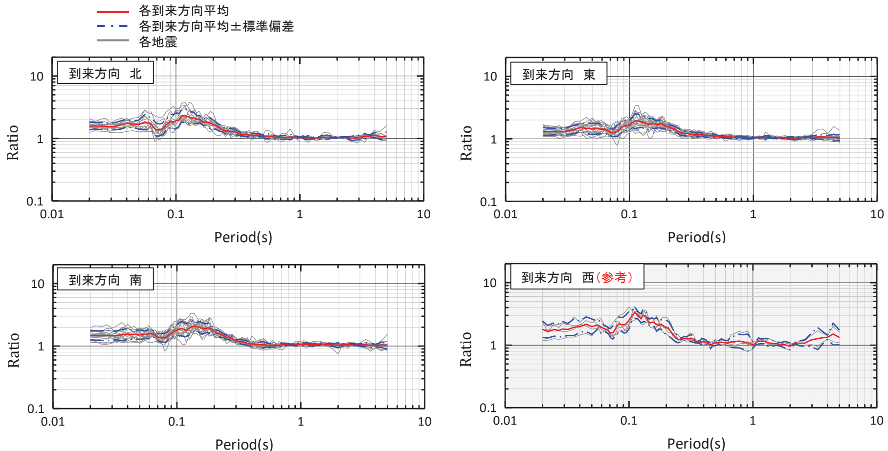
地震波到来方向別の応答スペクトル比 原子炉建屋直下 鉛直成分
