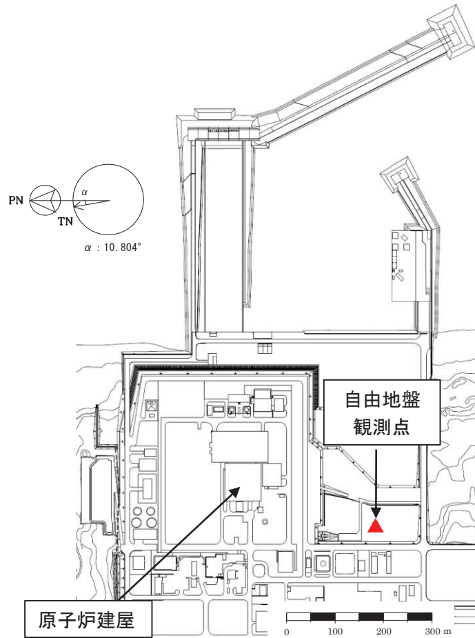
平面配置図
