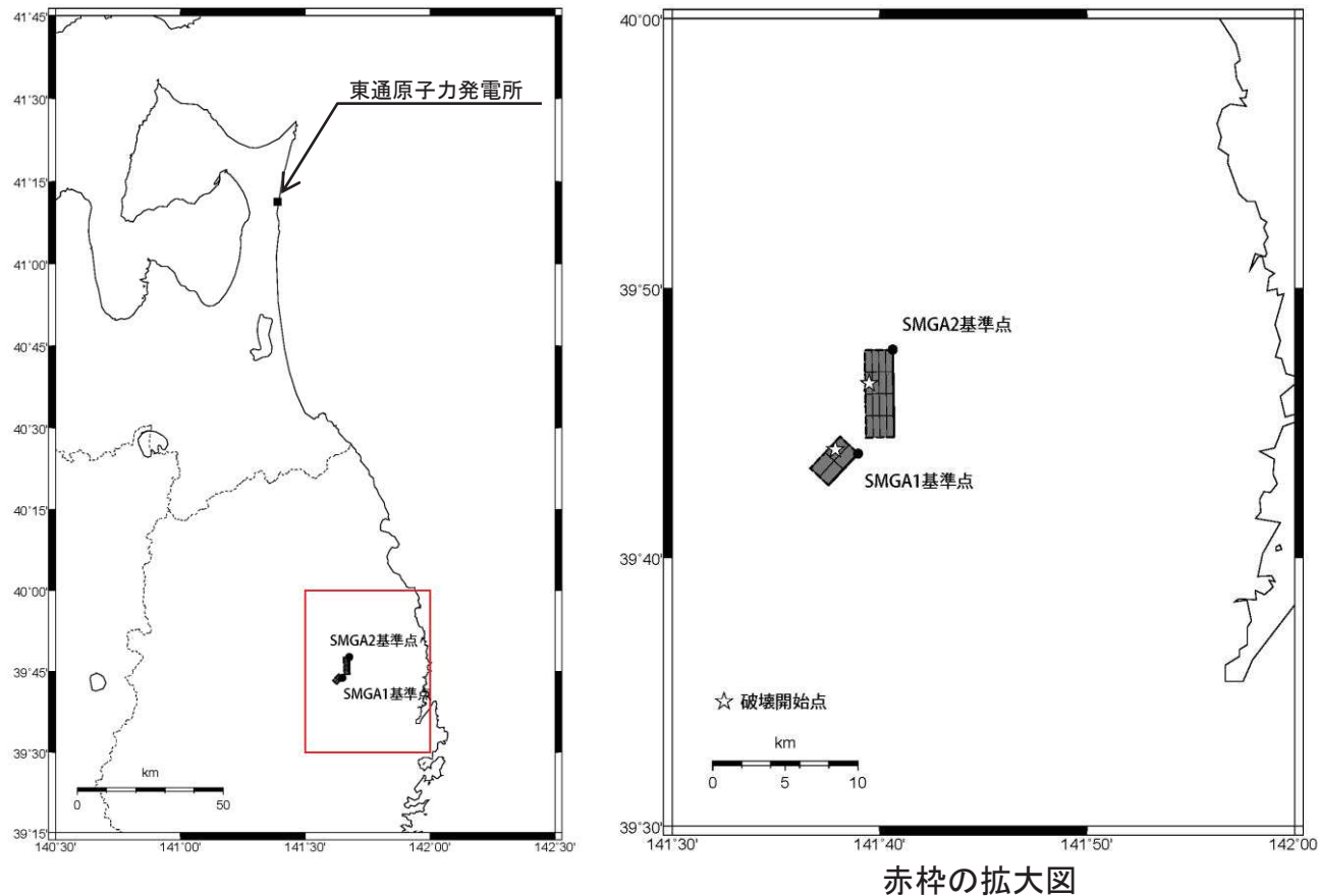
2008年岩手県沿岸北部の地震のシミュレーション解析に用いる震源断層モデル
