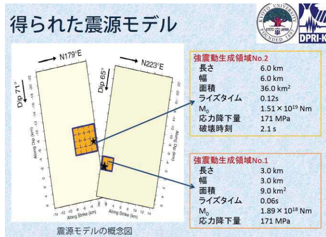
震源モデル
