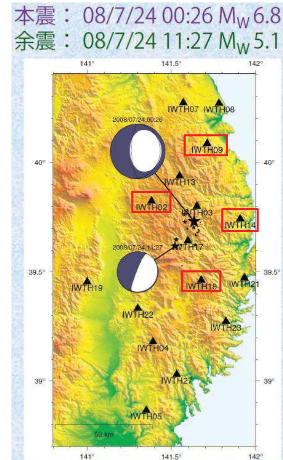
本震・余震の震央位置と観測点
