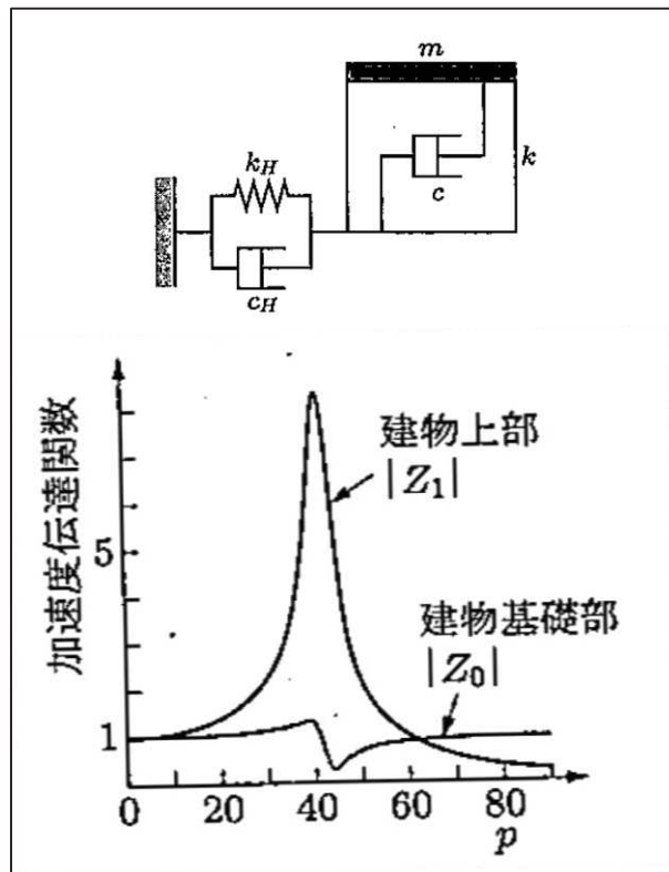
建物と地盤の相互作用を持つ1質点系 建物基礎部の応答 〔柴田(2014)より抜粋〕
