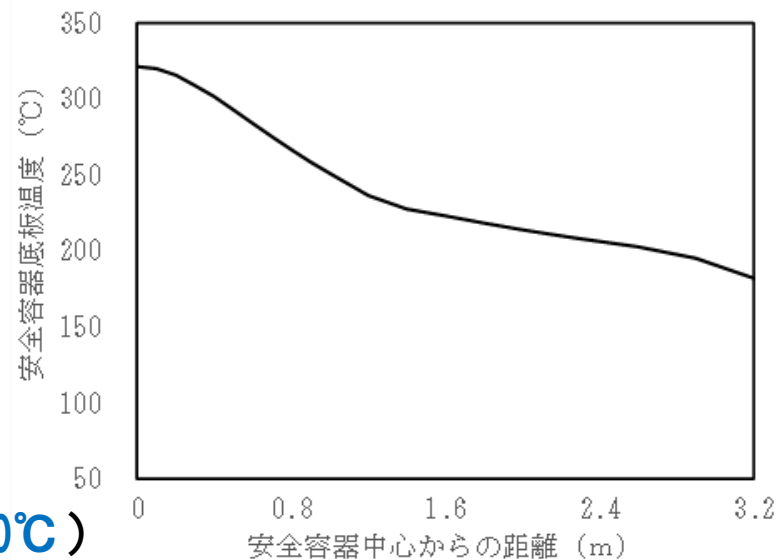
安全容器底板の径方向温度分布 (基本ケース、初期定常解析)
