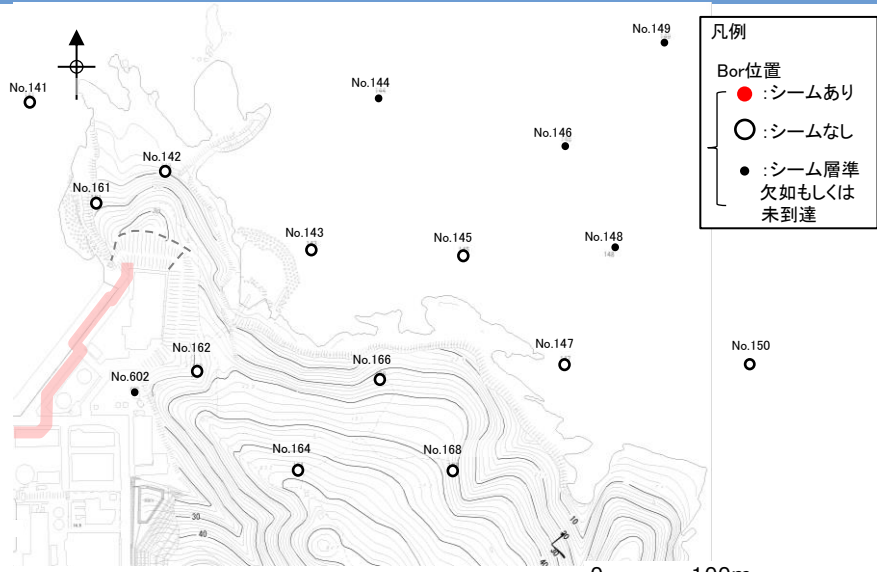
B29シームの有無の確認結果
