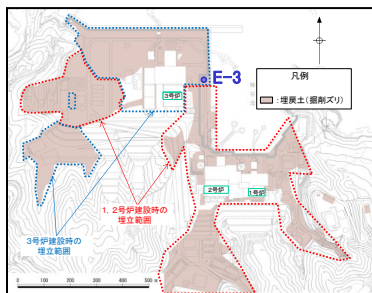
3号炉建設時の埋戻土 ボーリングNo. E-3 1.5m~17.4m
