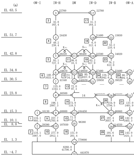
水平モデル(EW方向)
