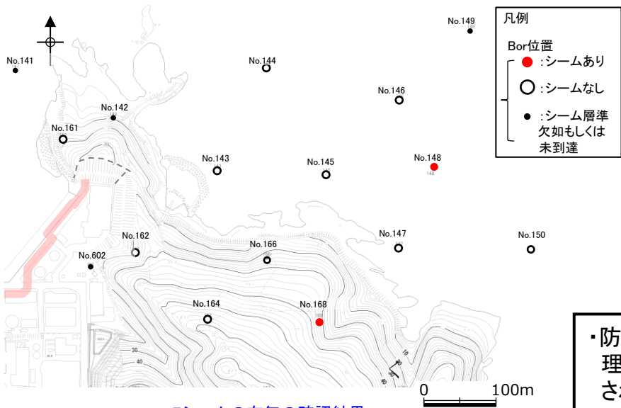
Eシームの有無の確認結果
