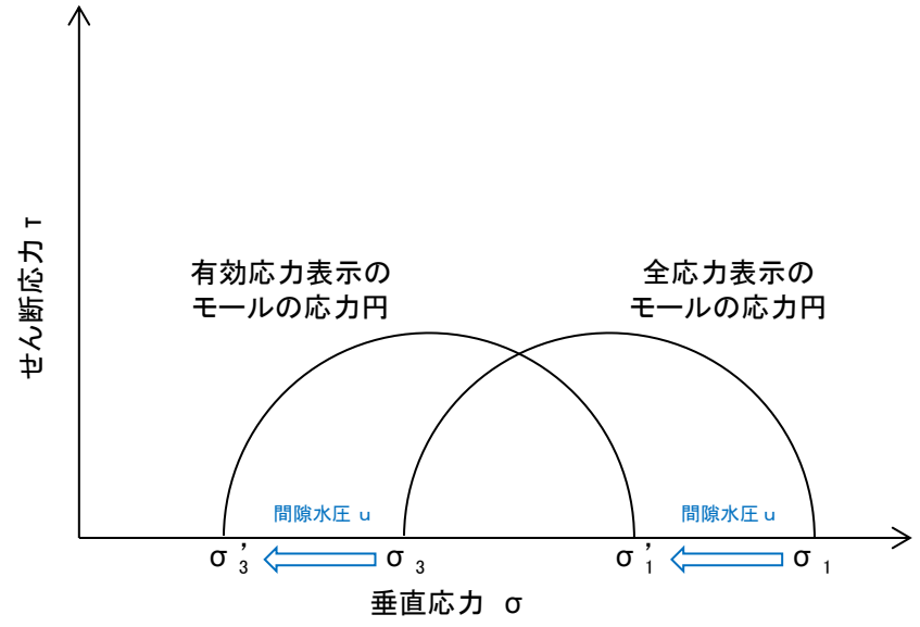
有効応力算定のイメージ図
