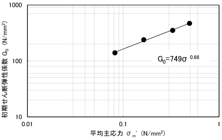
動的変形特性 (初期せん断弾性係数)
