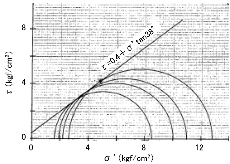
大型三軸圧縮試験(CU試験)の結果
