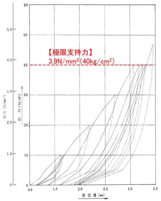
(a) 凝灰岩
