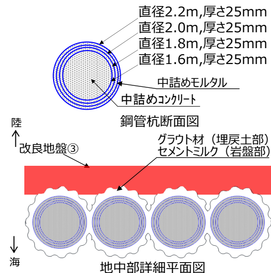
地中部詳細平面図
