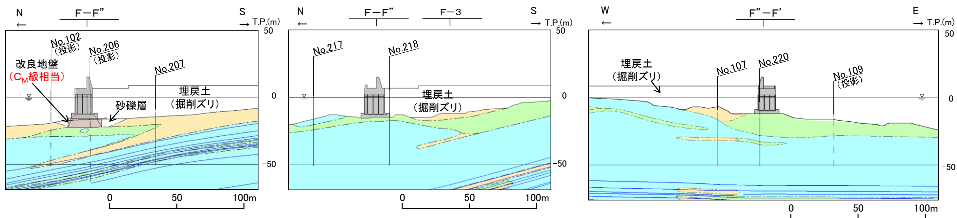
防波壁(波返重力擁壁) F-1 断面横断面図(岩級・シーム)
