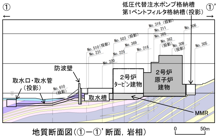
地質断面図(①-①'断面, 岩相)
