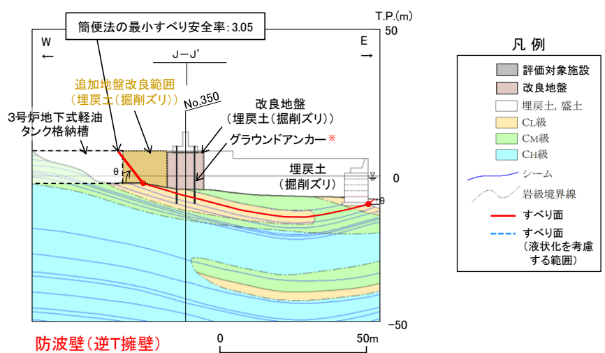
J-3断面 簡便法の結果
