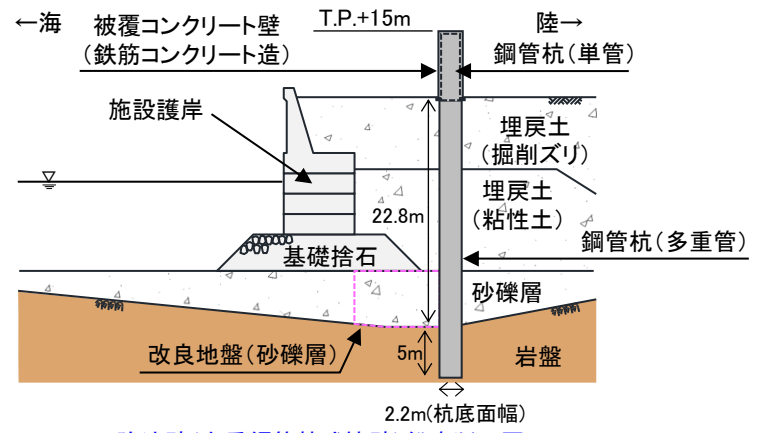
防波壁(多重鋼管杭式擁壁)鉛直断面図
