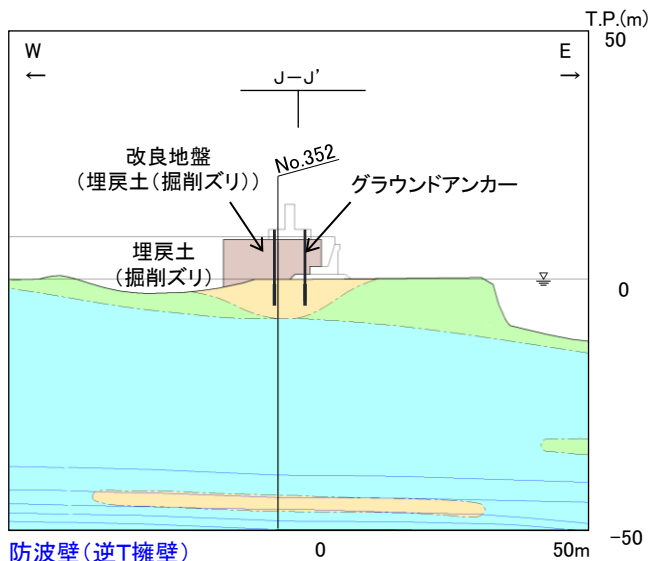
防波壁(逆T擁壁) J-1断面 横断面図(岩級・シーム)
