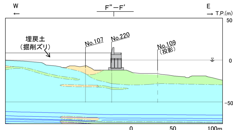
防波壁(波返重力擁壁)
