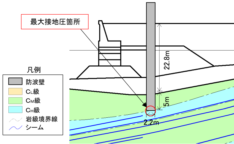
防波壁(多重鋼管杭式擁壁)
