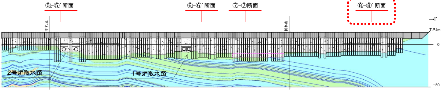
検討断面位置図
