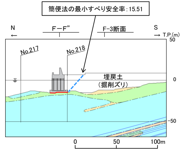
防波壁(波返重力擁壁) F-2断面横断面図(岩級・シーム)
