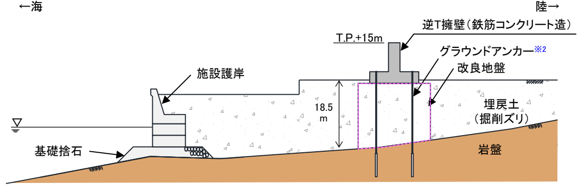
防波壁(逆T擁壁)鉛直断面図※1
