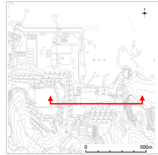
断面位置図
