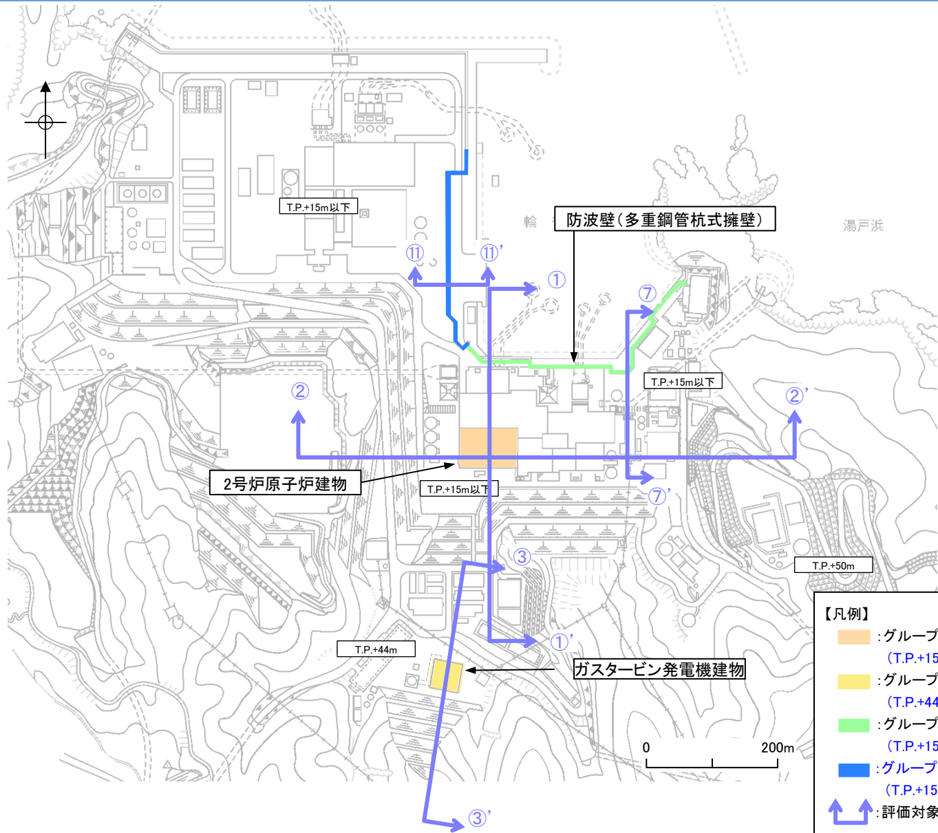
評価対象断面の選定結果
