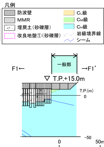
防波壁縦断面図(波返重力擁壁)
