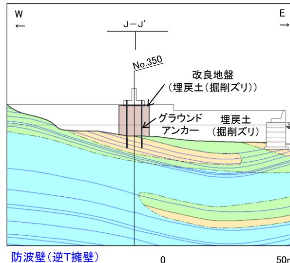
防波壁(逆T擁壁) J-3断面 横断面図(岩級・シーム)
