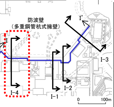
断面位置図
