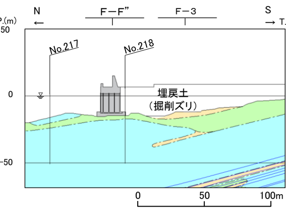
防波壁(波返重力擁壁)
