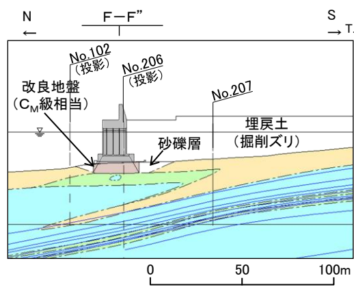
防波壁(波返重力擁壁)
