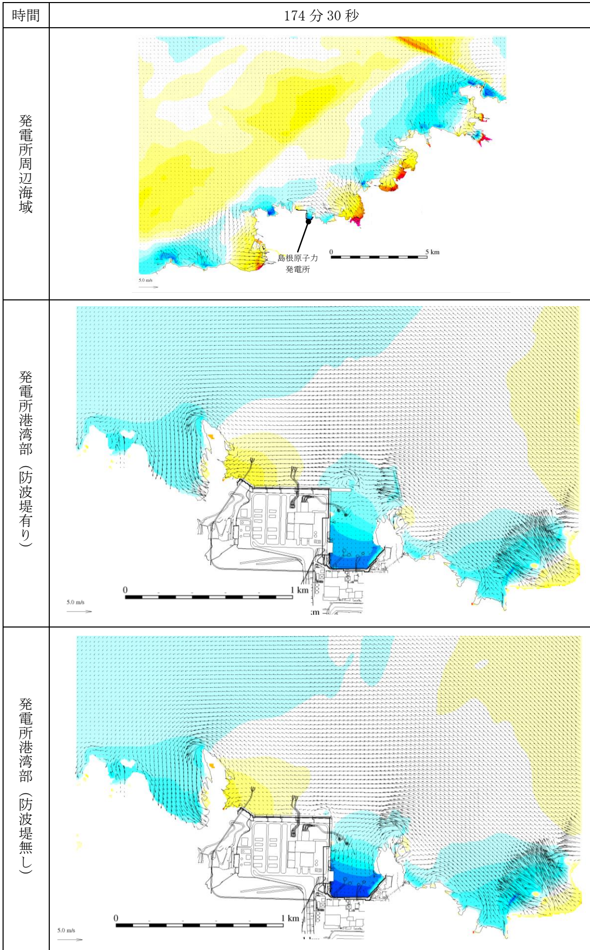
第 1 図 (150) 基準津波 1 の水位変動・流向ベクトル
