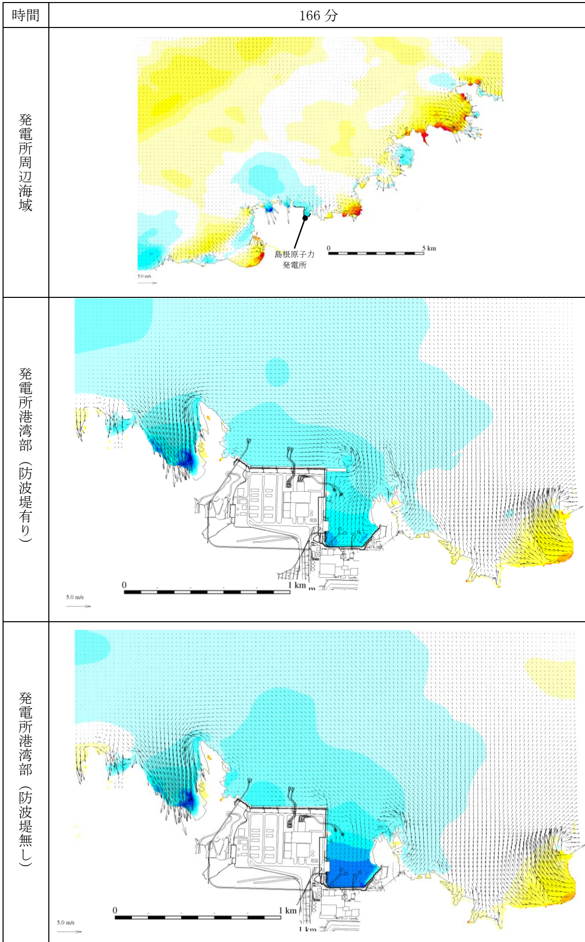
第 1 図(133) 基準津波 1 の水位変動・流向ベクトル
