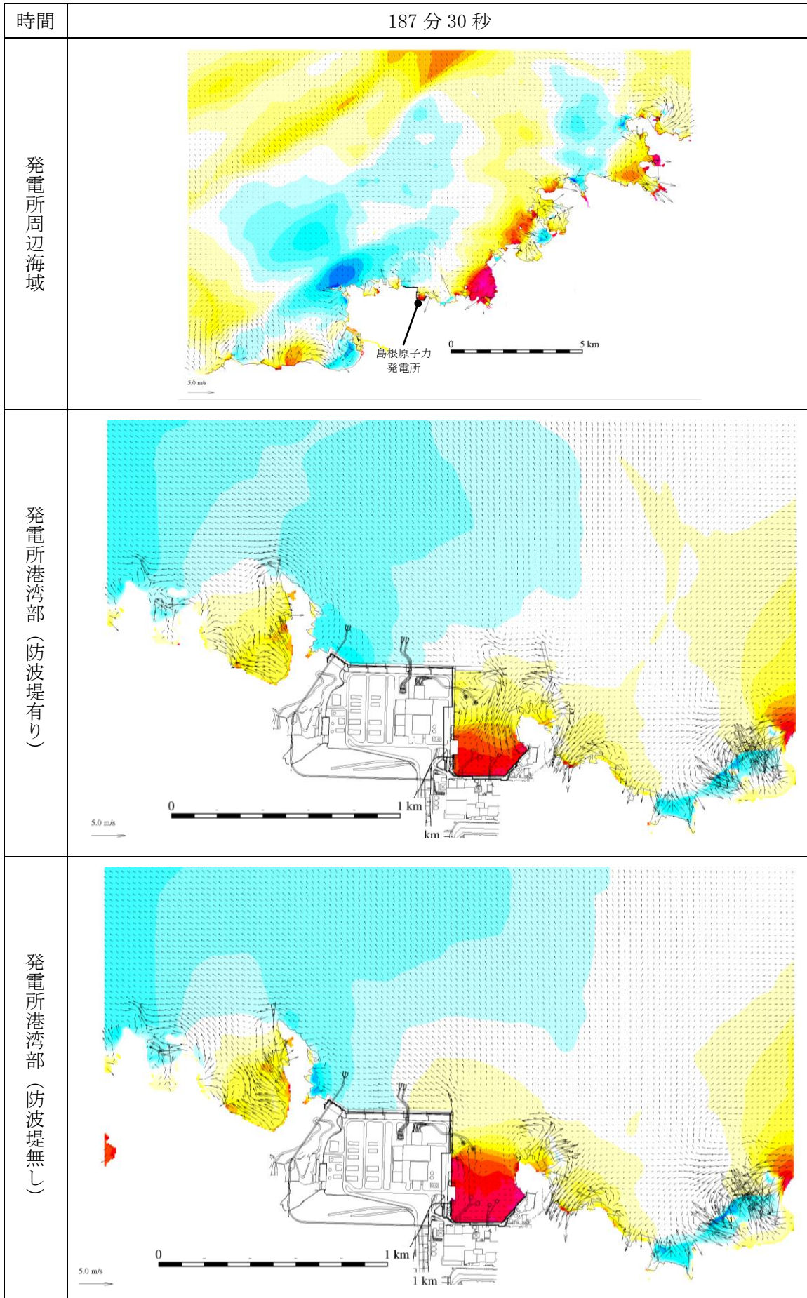
第 1 図 (176) 基準津波 1 の水位変動・流向ベクトル
