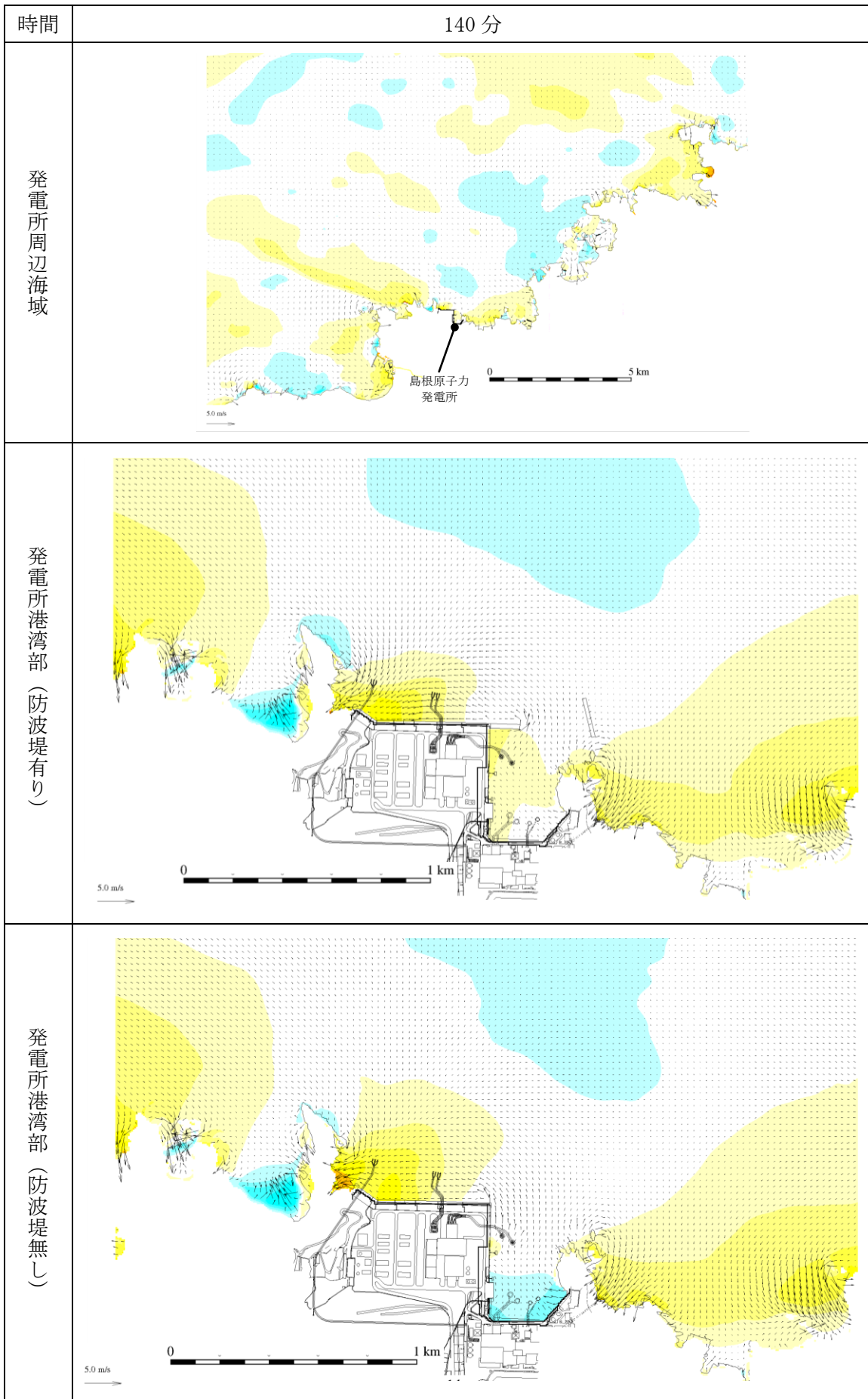
第 1 図(81) 基準津波 1 の水位変動・流向ベクトル
