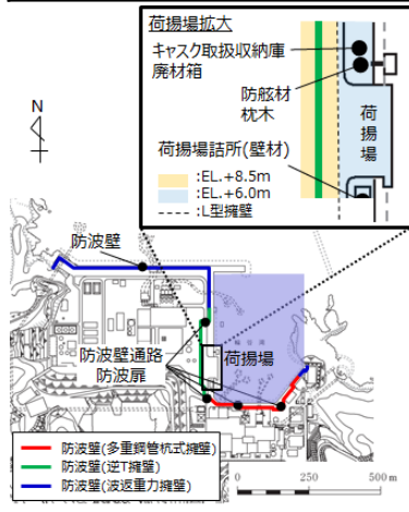
港湾内に面する津波防護施設に考慮する漂流物の配置
