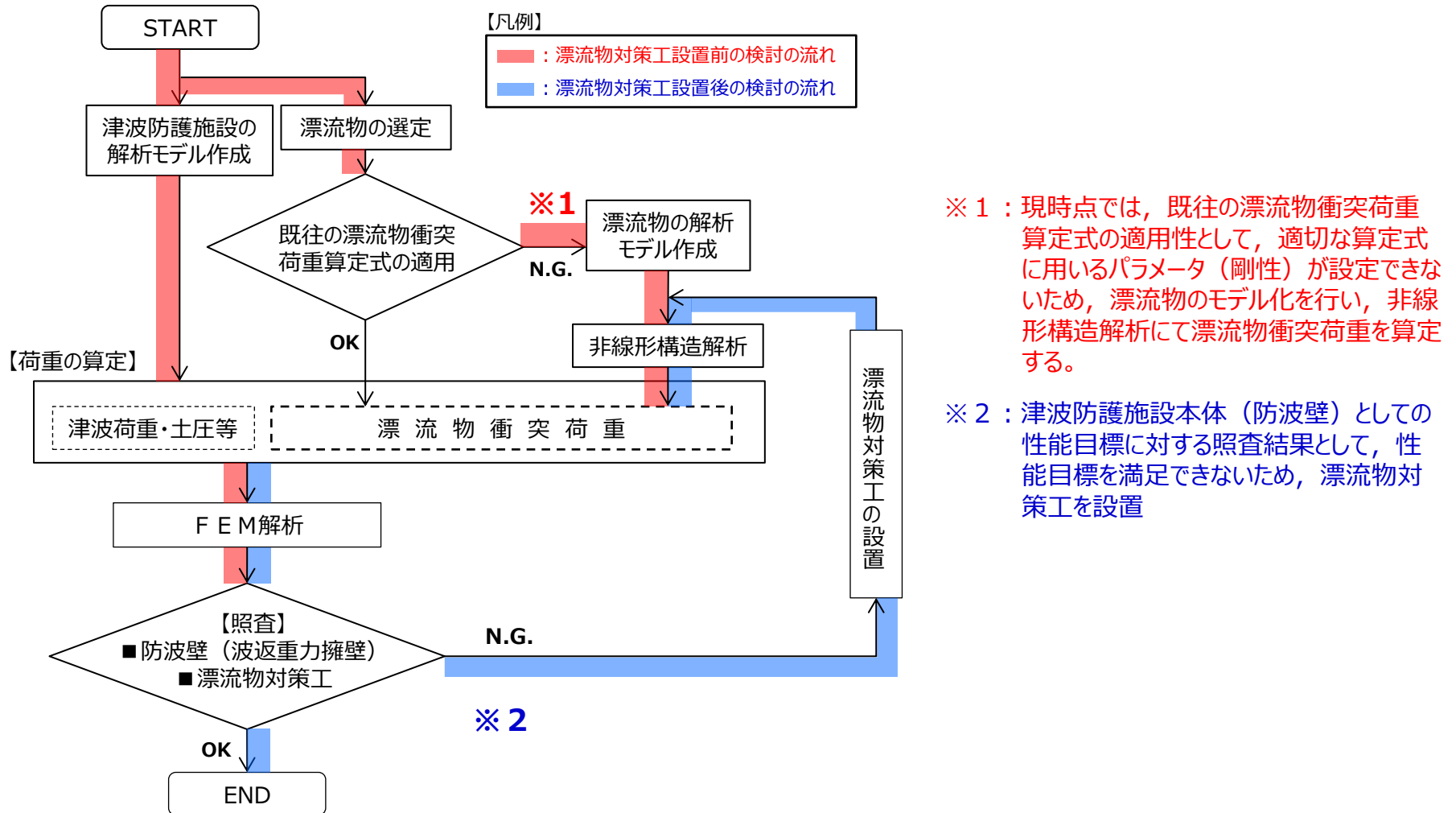
（例）津波防護施設（防波壁:波返重力擁壁）における漂流物対策工に係る検討の流れ
