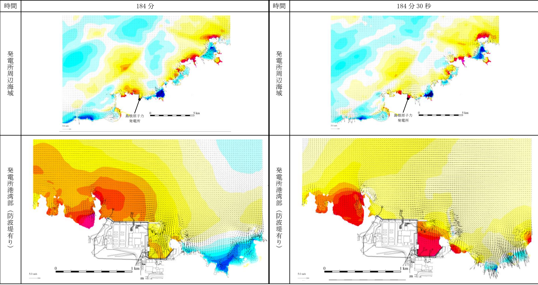
水位変動・流向ベクトル（基準津波 1（防波堤有り） 184分， 184分30秒）
