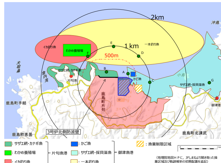
防波壁 (多重鋼管杭式擁壁)
