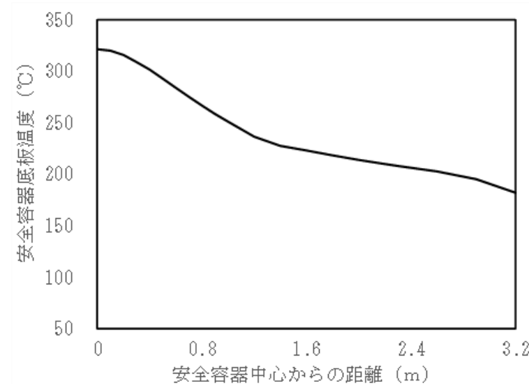
安全容器底板の径方向温度分布
