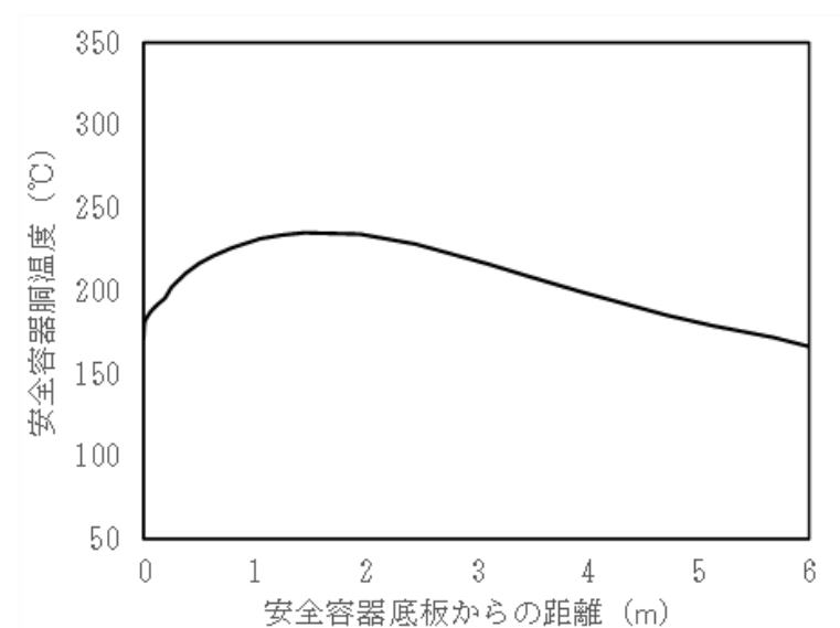
安全容器胴部の軸方向温度分布
