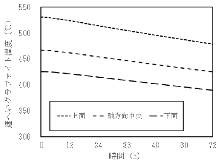
遮へいグラファイト温度の時間変化
