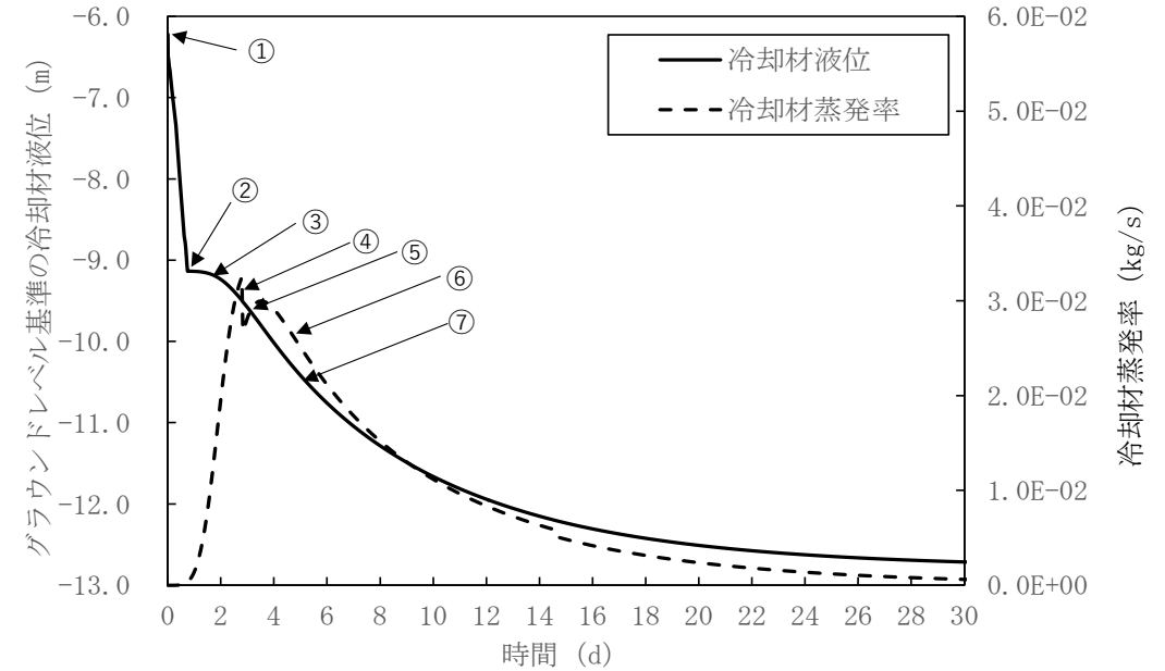
冷却材液位及び冷却材蒸発率の推移
