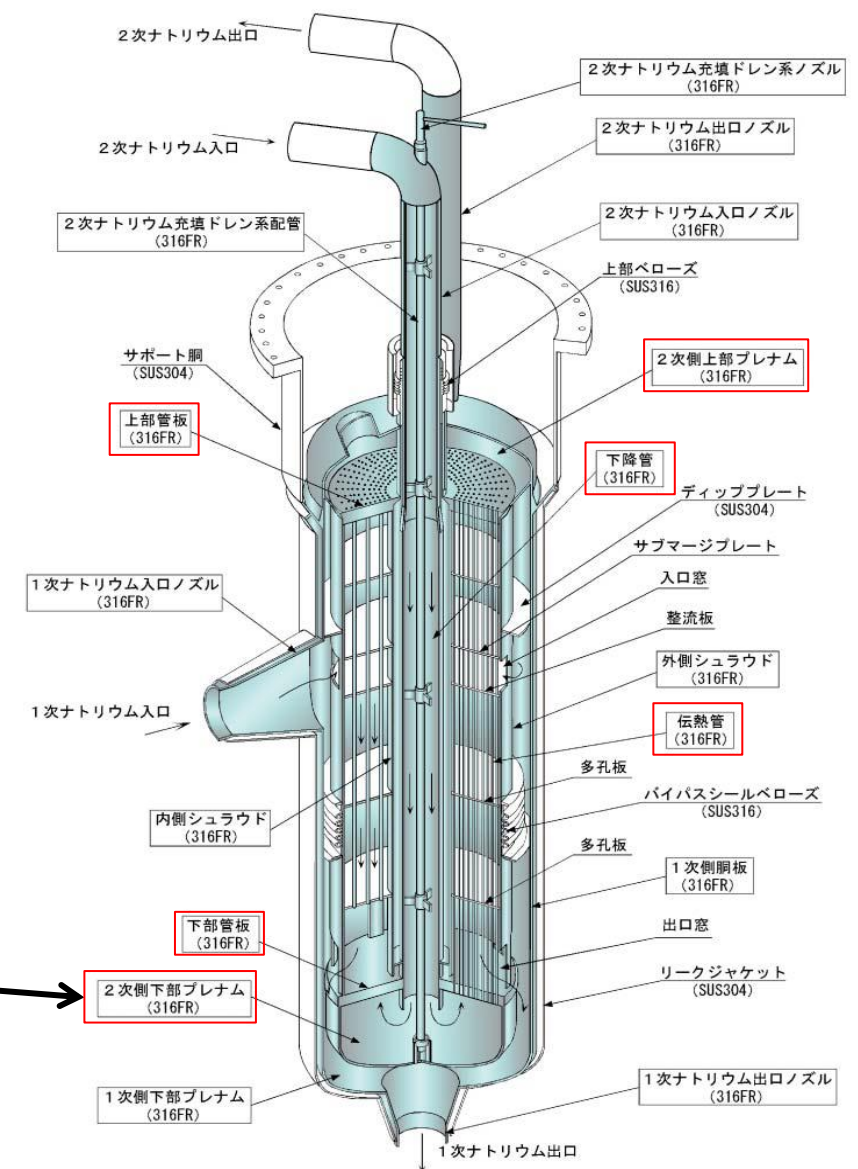
主中間熱交換器の構造
