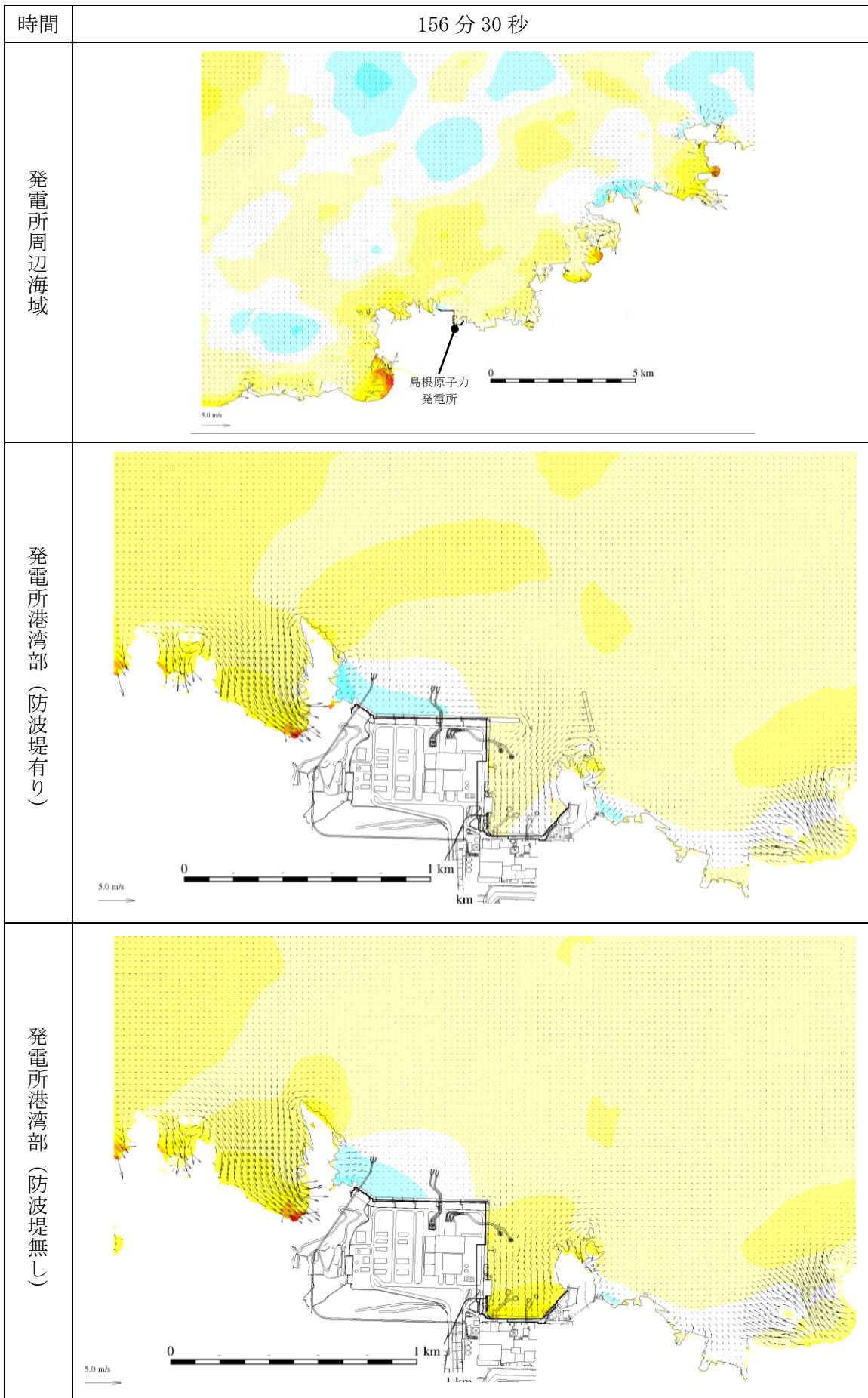
第 1 図(114) 基準津波 1 の水位変動・流向ベクトル
