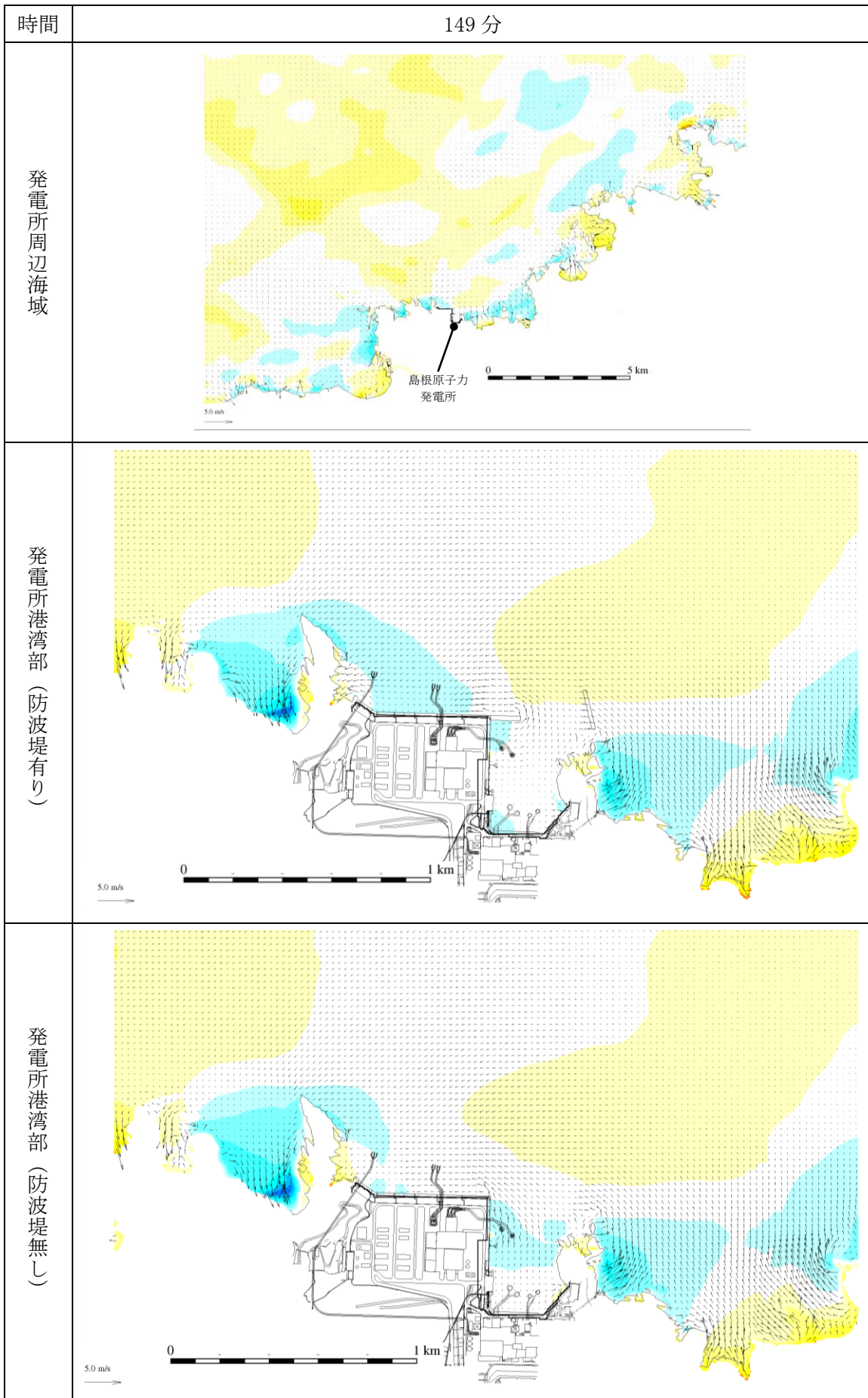
第 1 図(99) 基準津波 1 の水位変動・流向ベクトル
