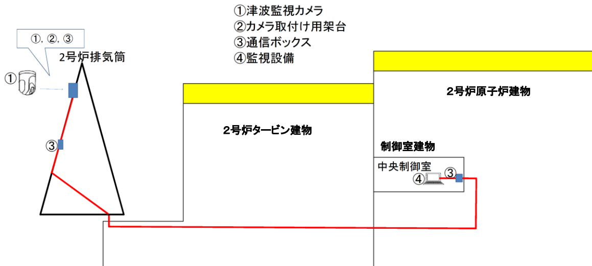
第4.3-5図 津波監視カメラ設備構成
