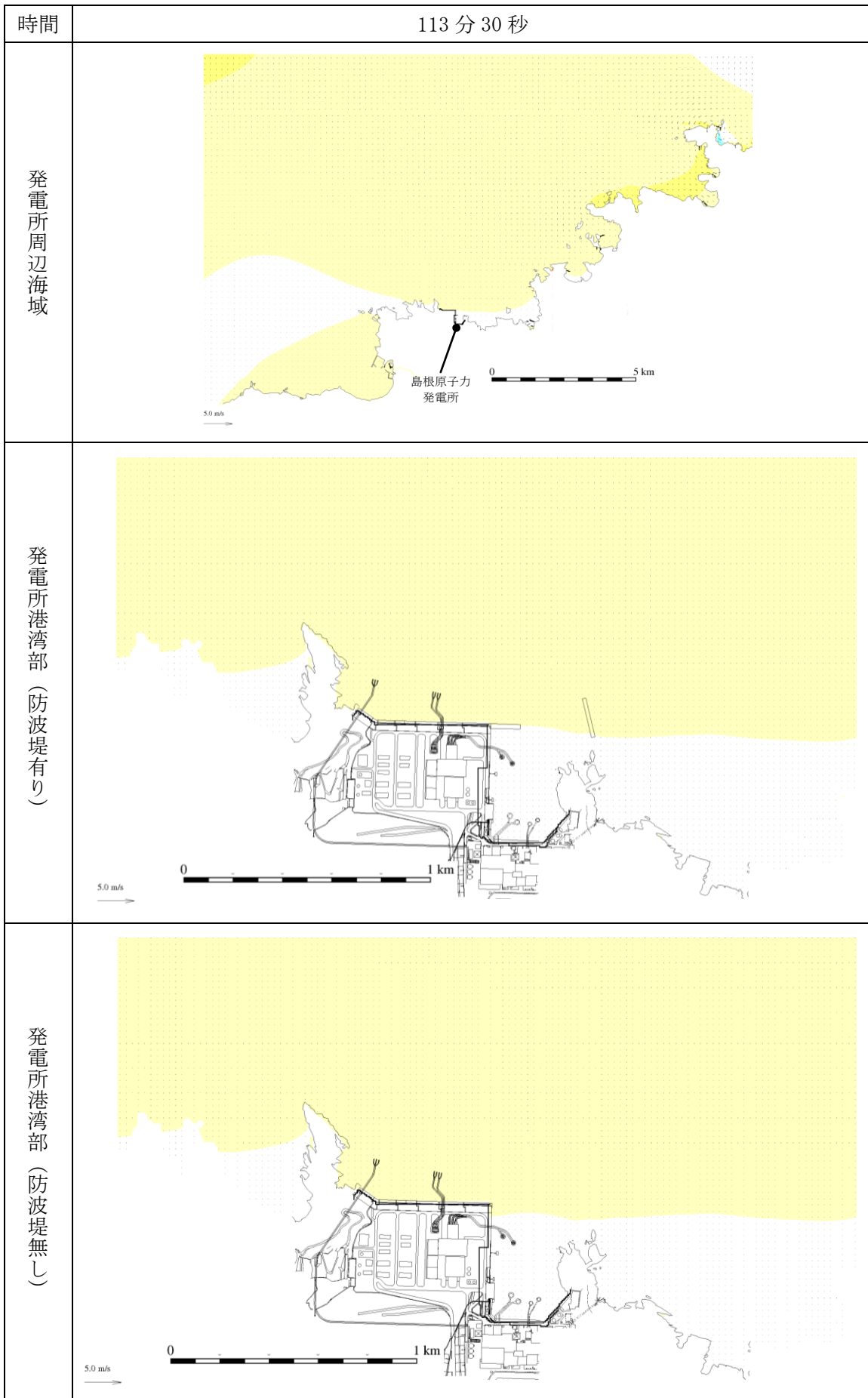
第 1 図(28) 基準津波 1 の水位変動・流向ベクトル
