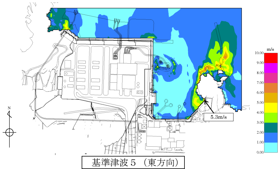
図8 基準津波 5 最大流速分布 (2 / 2)
