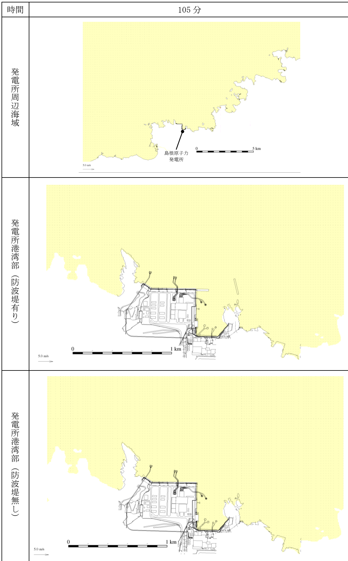
第 1 図(11) 基準津波 1 の水位変動・流向ベクトル
