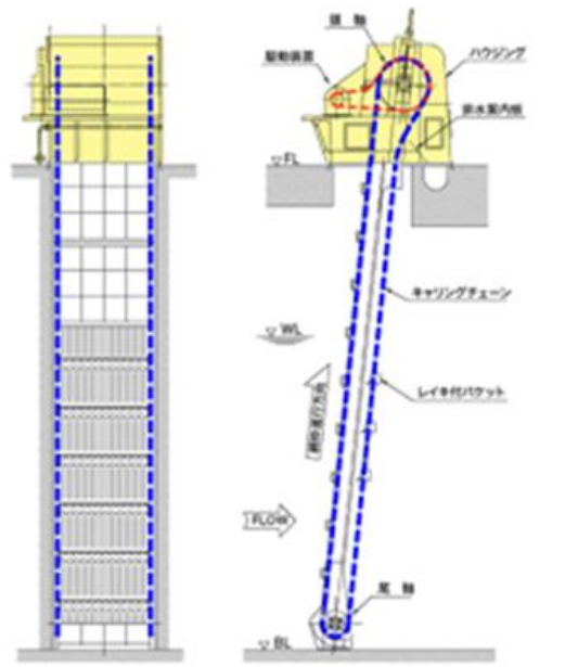
第 2.5-30 図 除塵装置の概要
