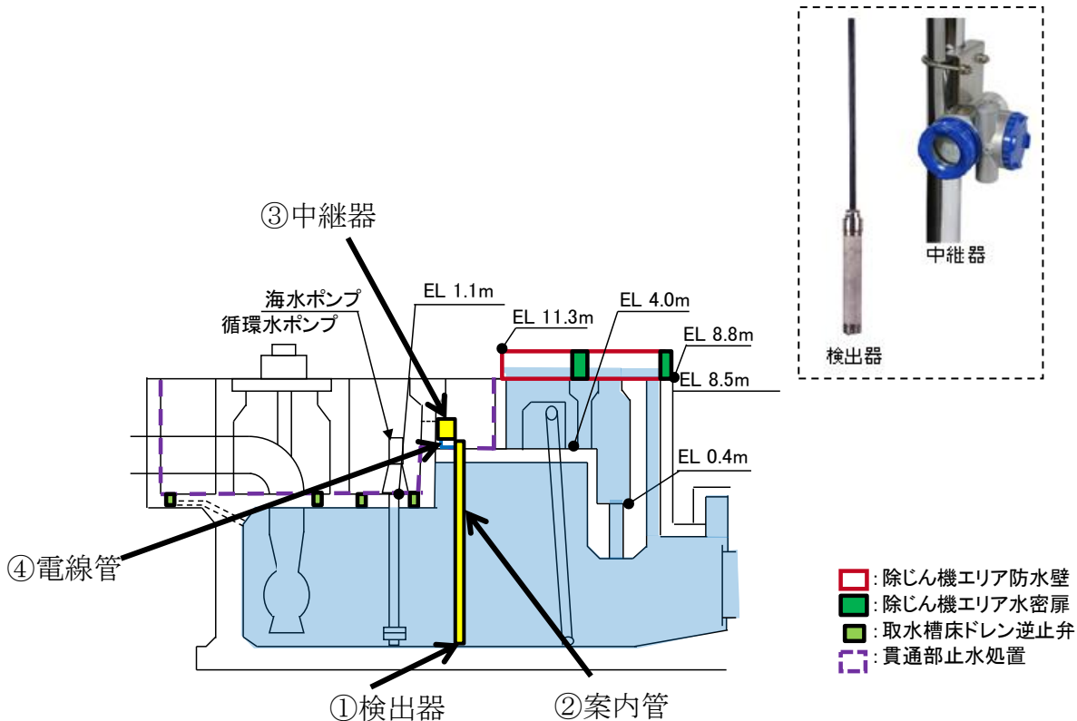
第4.3-7図 取水槽水位計の設置位置及び設備構成
