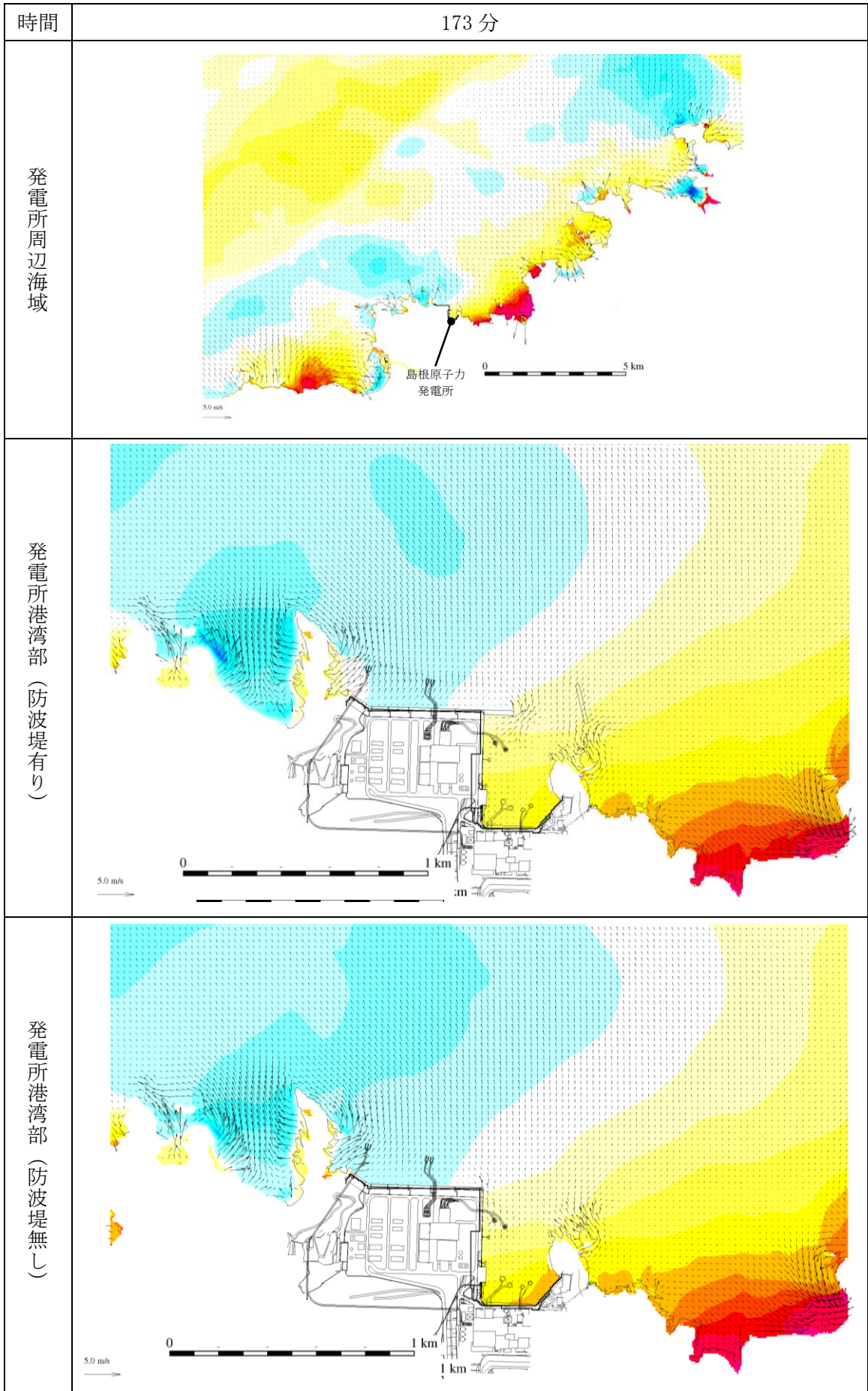
第 1 図(147) 基準津波 1 の水位変動・流向ベクトル
