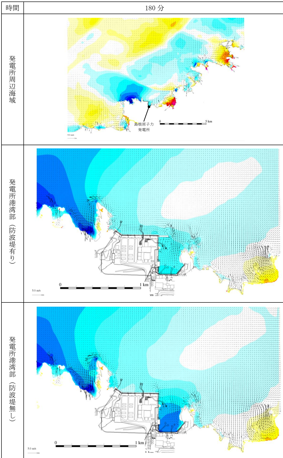
第 1 図(161) 基準津波 1 の水位変動・流向ベクトル
