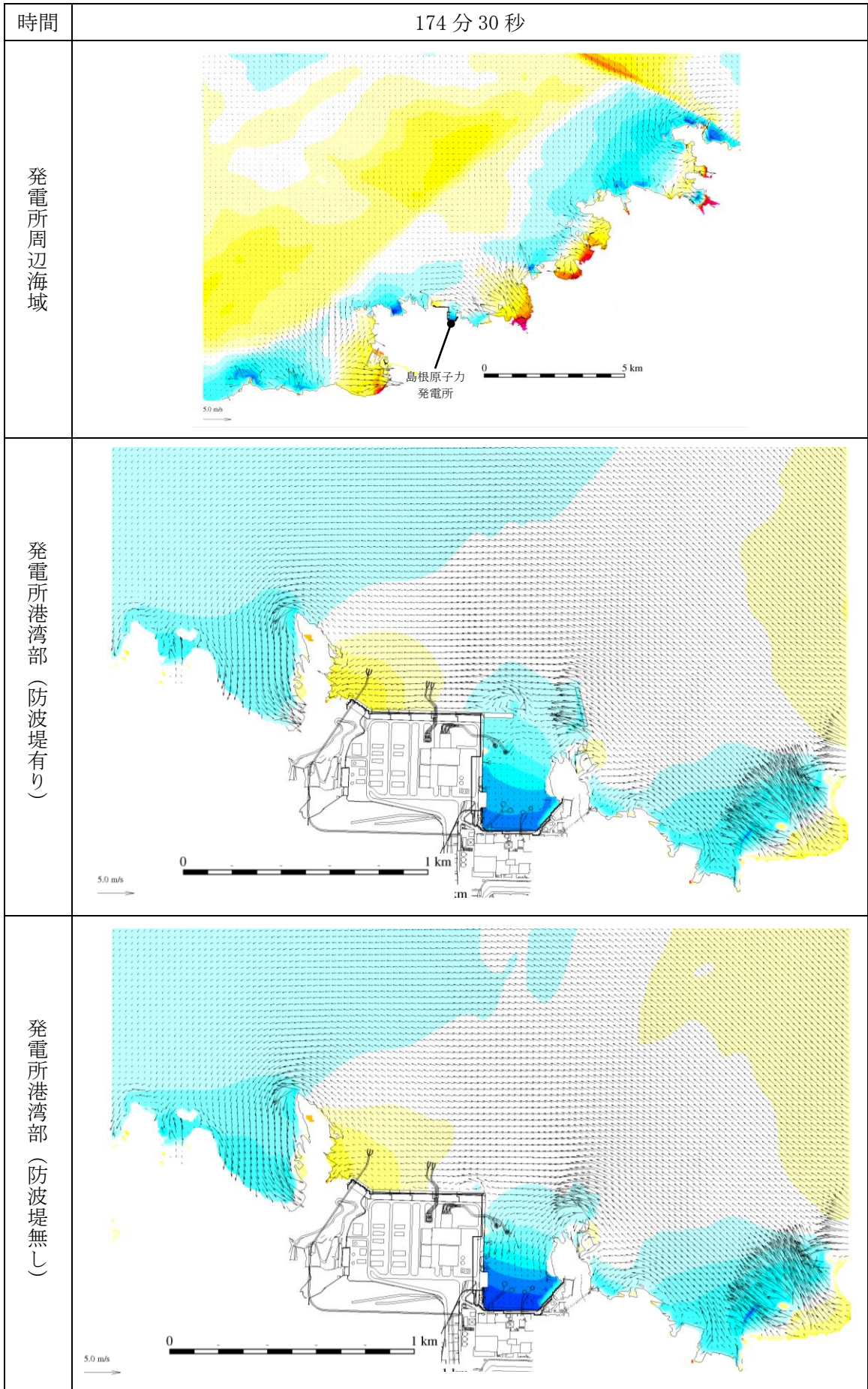
第 1 図 (150) 基準津波 1 の水位変動・流向ベクトル
