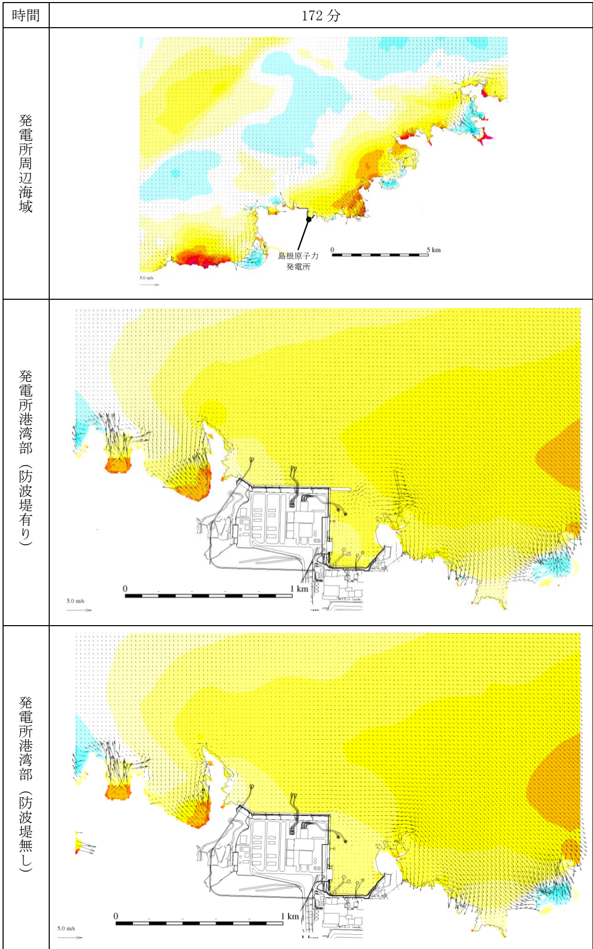
第 1 図(145) 基準津波 1 の水位変動・流向ベクトル
