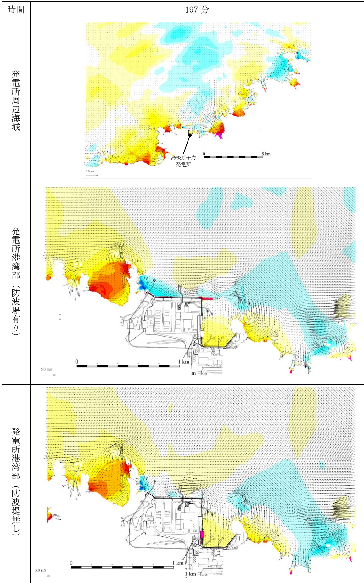
第 1 図(195) 基準津波 1 の水位変動・流向ベクトル
