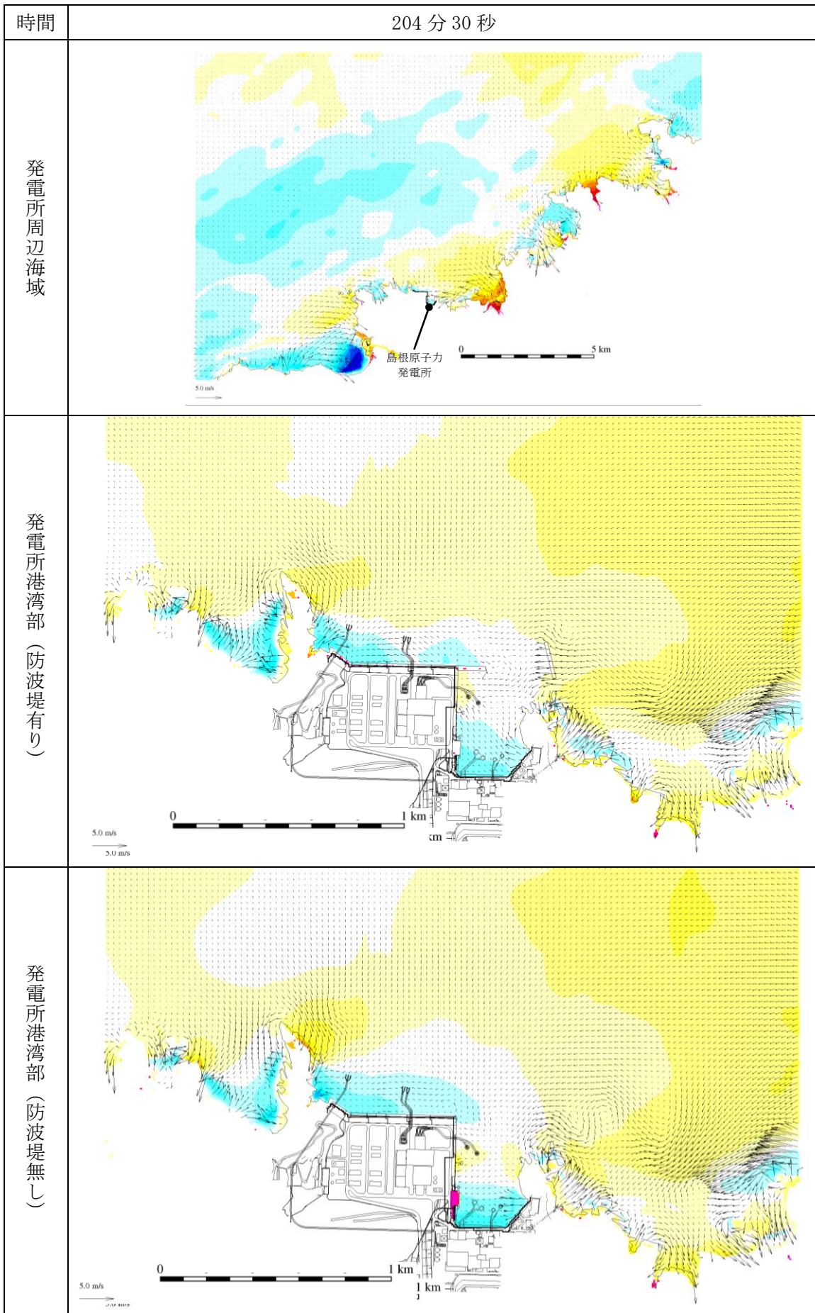
第 1 図 (210) 基準津波 1 の水位変動・流向ベクトル
