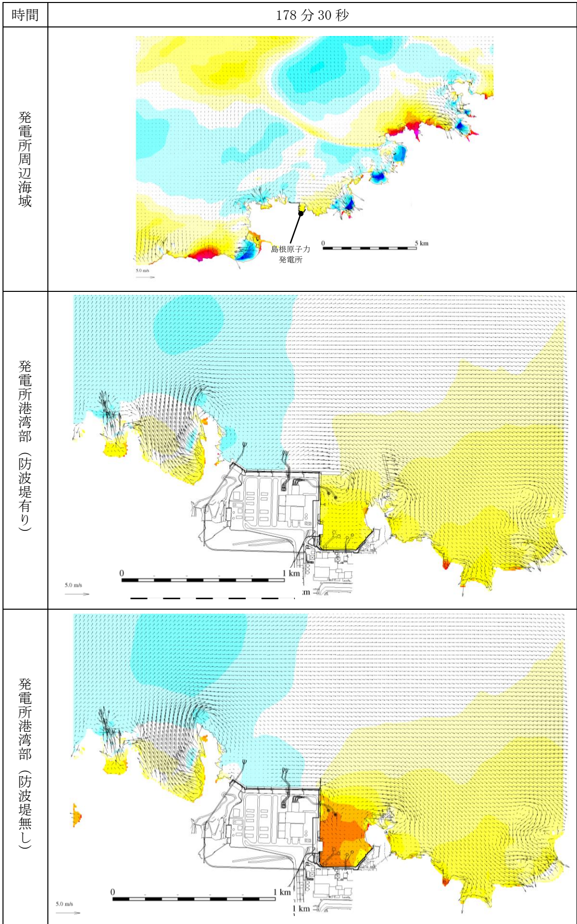
第 1 図(158) 基準津波 1 の水位変動・流向ベクトル
