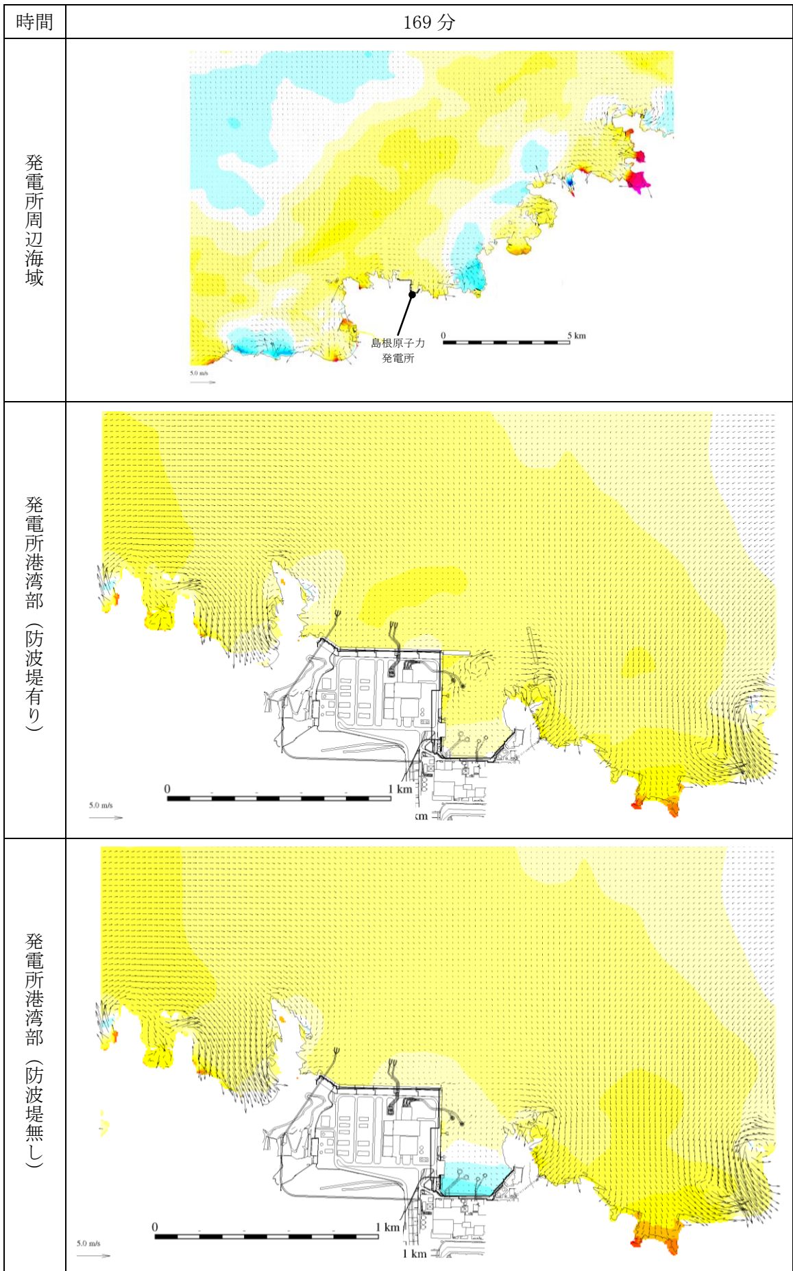
第 1 図 (139) 基準津波 1 の水位変動・流向ベクトル
