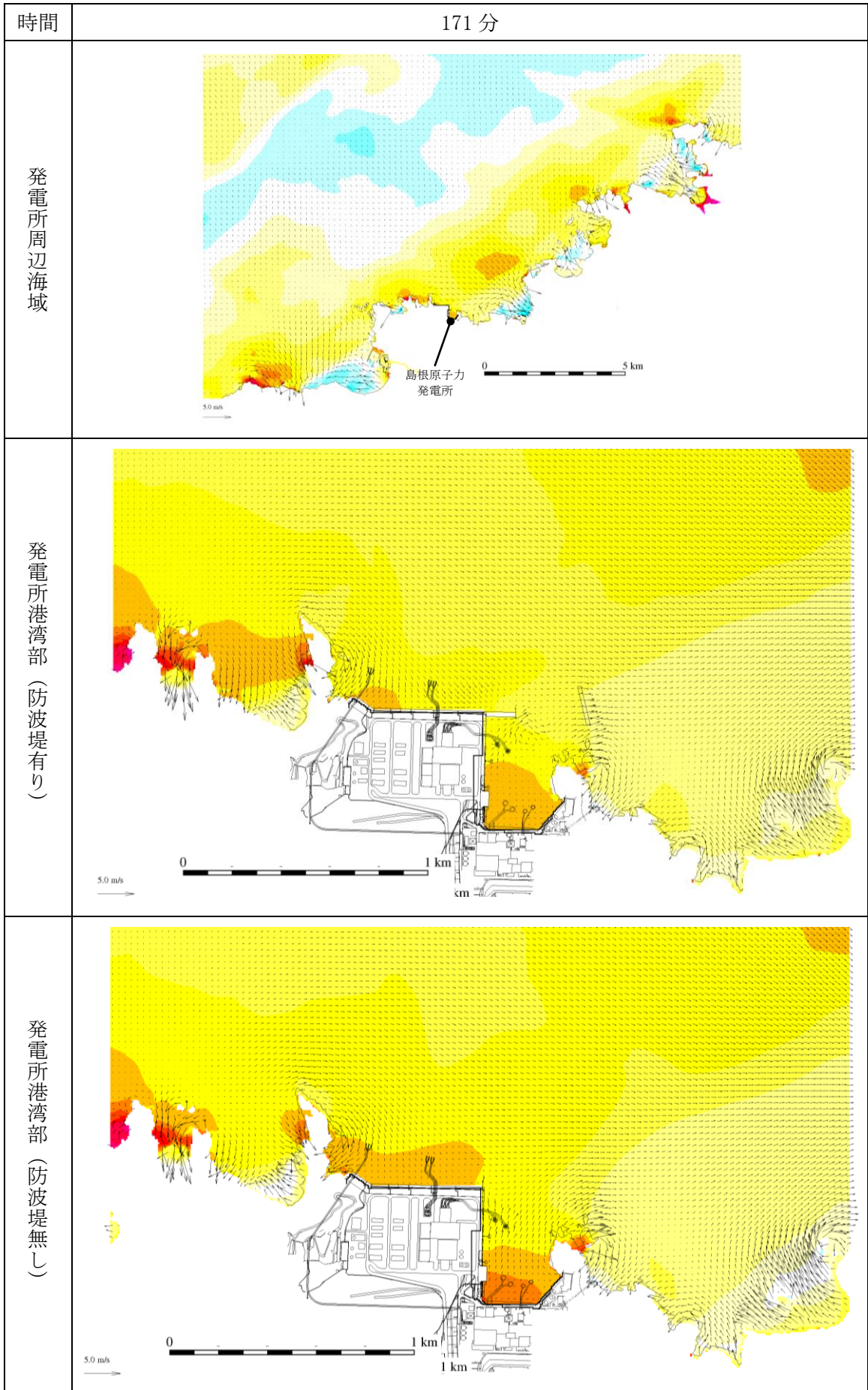
第 1 図(143) 基準津波 1 の水位変動・流向ベクトル
