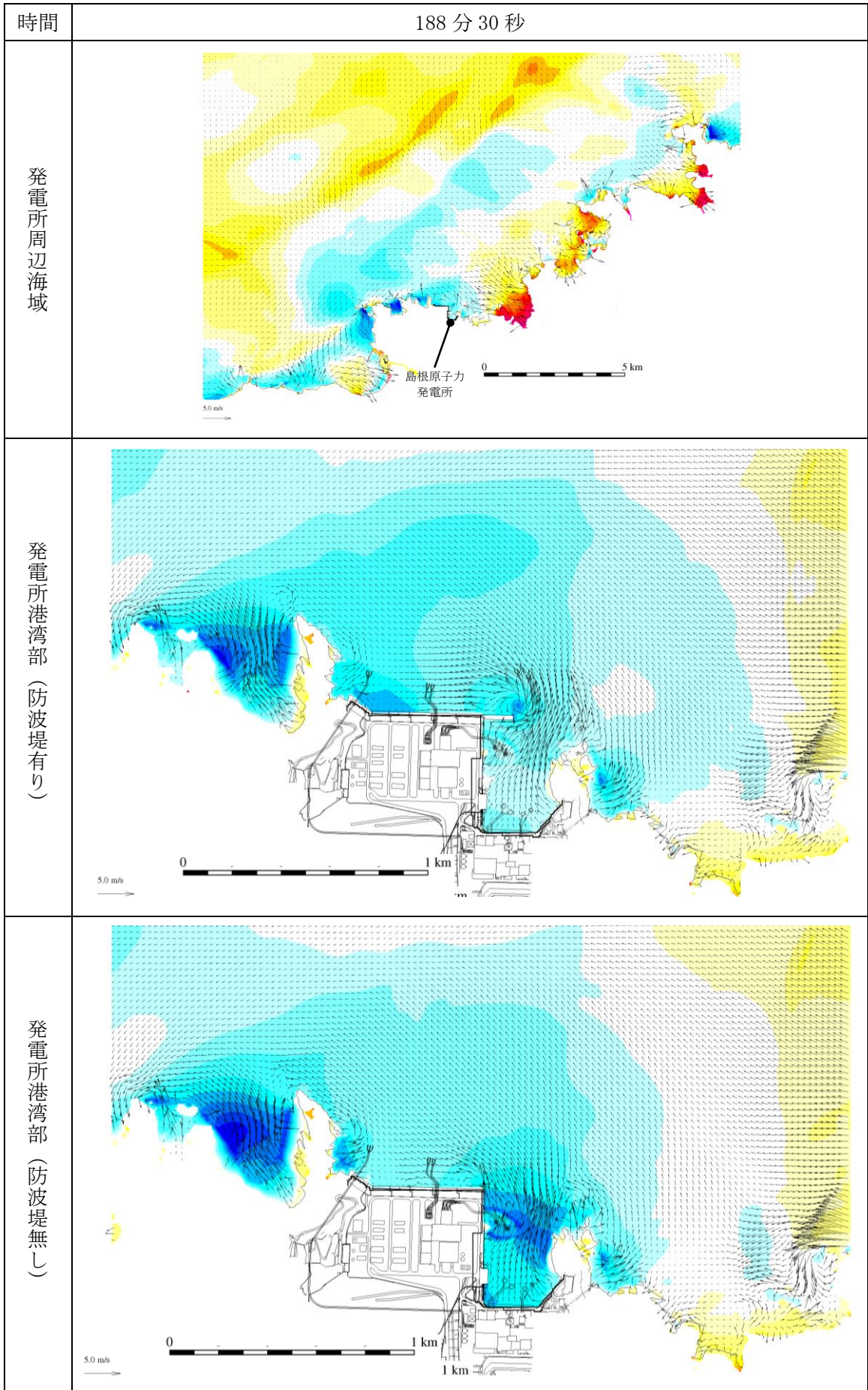
第 1 図(178) 基準津波 1 の水位変動・流向ベクトル
