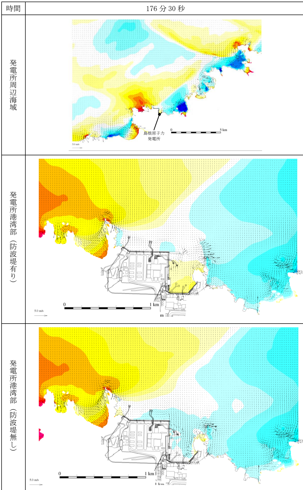
第 1 図 (154) 基準津波 1 の水位変動・流向ベクトル
