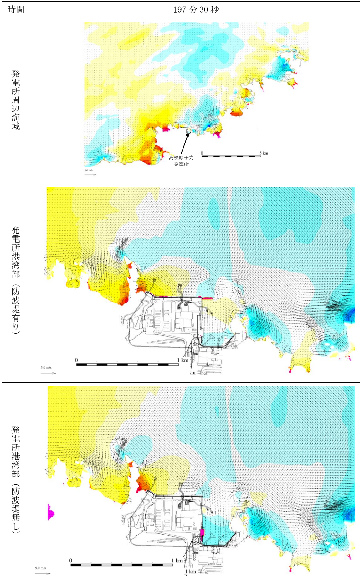
第 1 図(196) 基準津波 1 の水位変動・流向ベクトル
