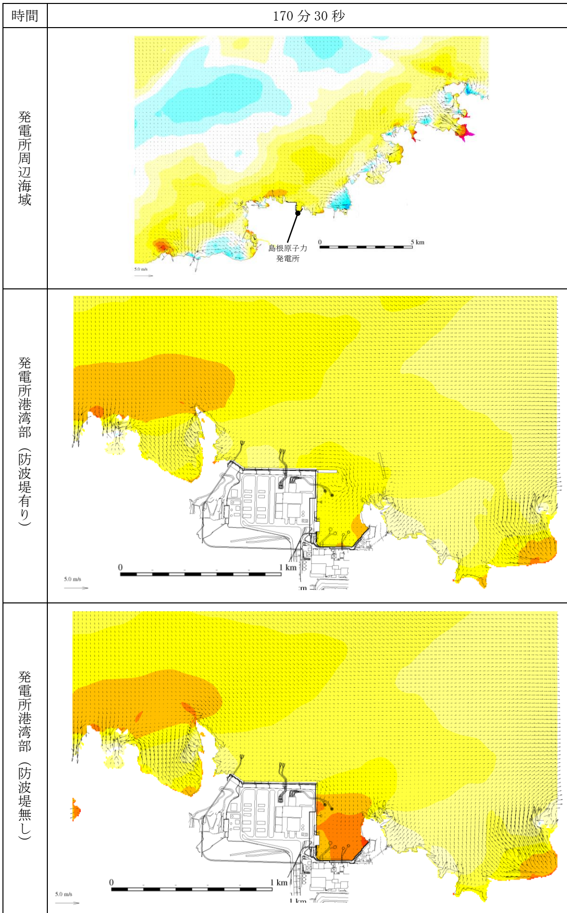
第 1 図(142) 基準津波 1 の水位変動・流向ベクトル
