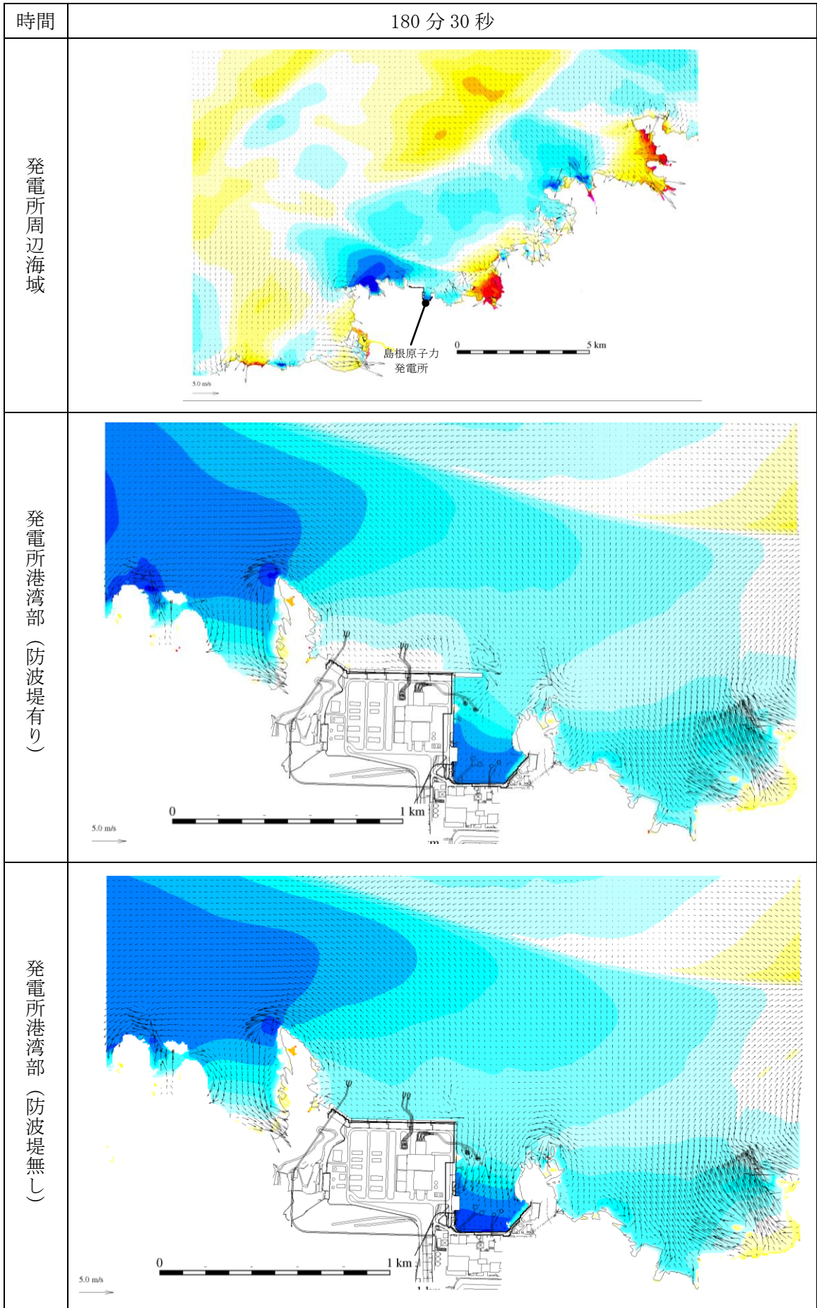
第 1 図(162) 基準津波 1 の水位変動・流向ベクトル
