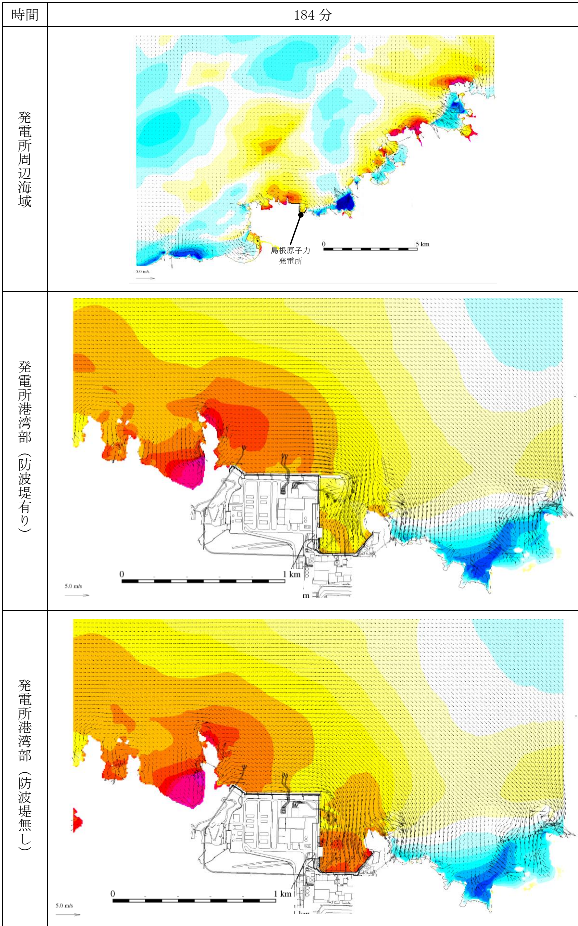
第 1 図(169) 基準津波 1 の水位変動・流向ベクトル
