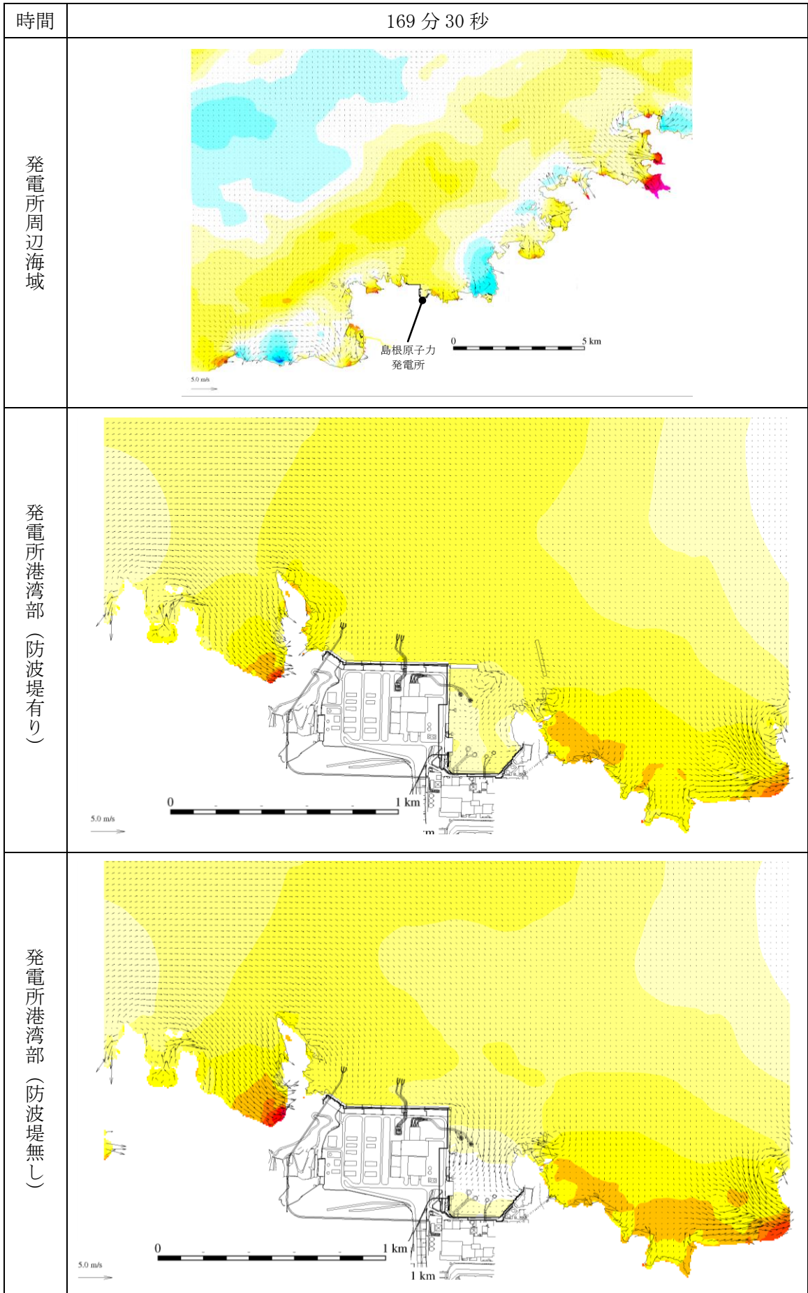
第 1 図(140) 基準津波 1 の水位変動・流向ベクトル
