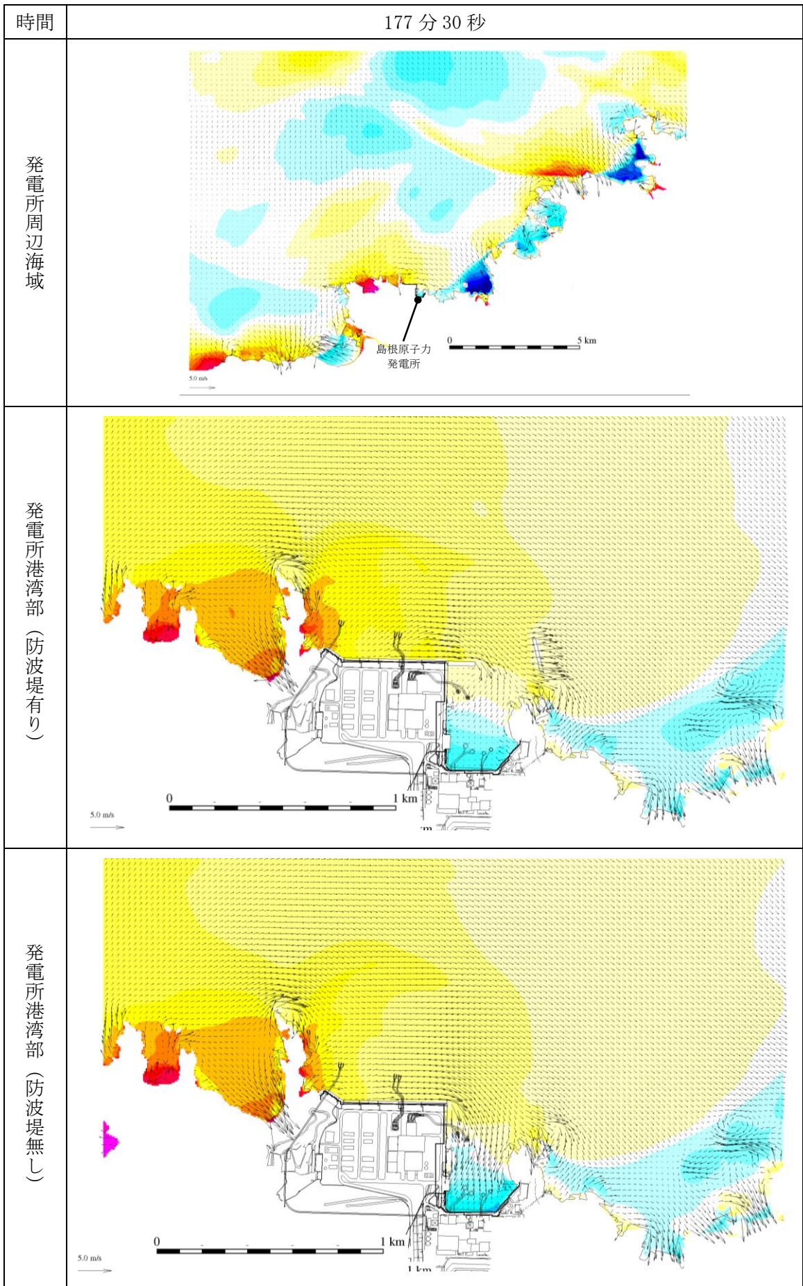
第 1 図 (156) 基準津波 1 の水位変動・流向ベクトル
