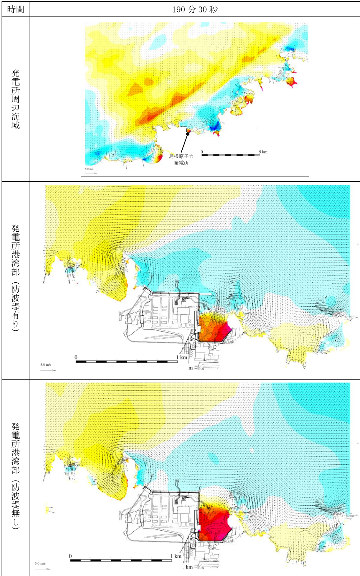
第 1 図(182) 基準津波 1 の水位変動・流向ベクトル
