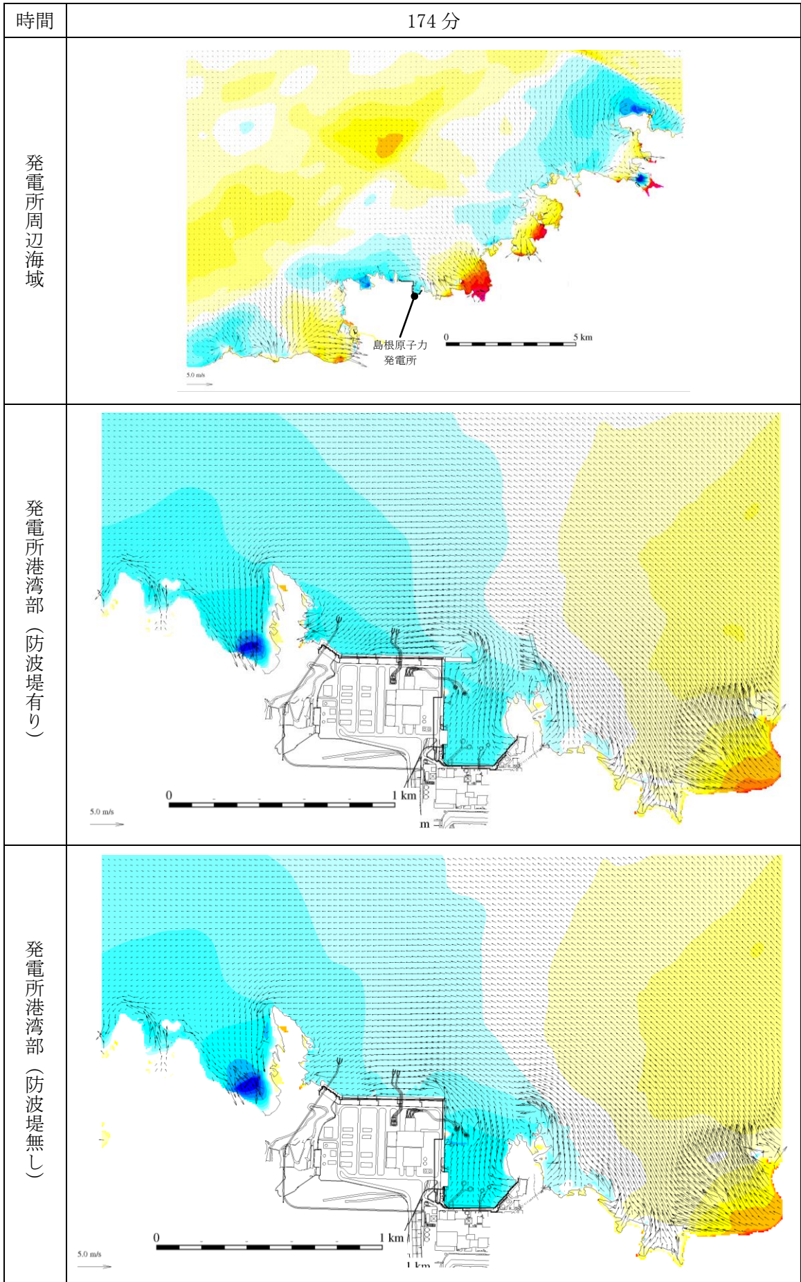
第 1 図(149) 基準津波 1 の水位変動・流向ベクトル
