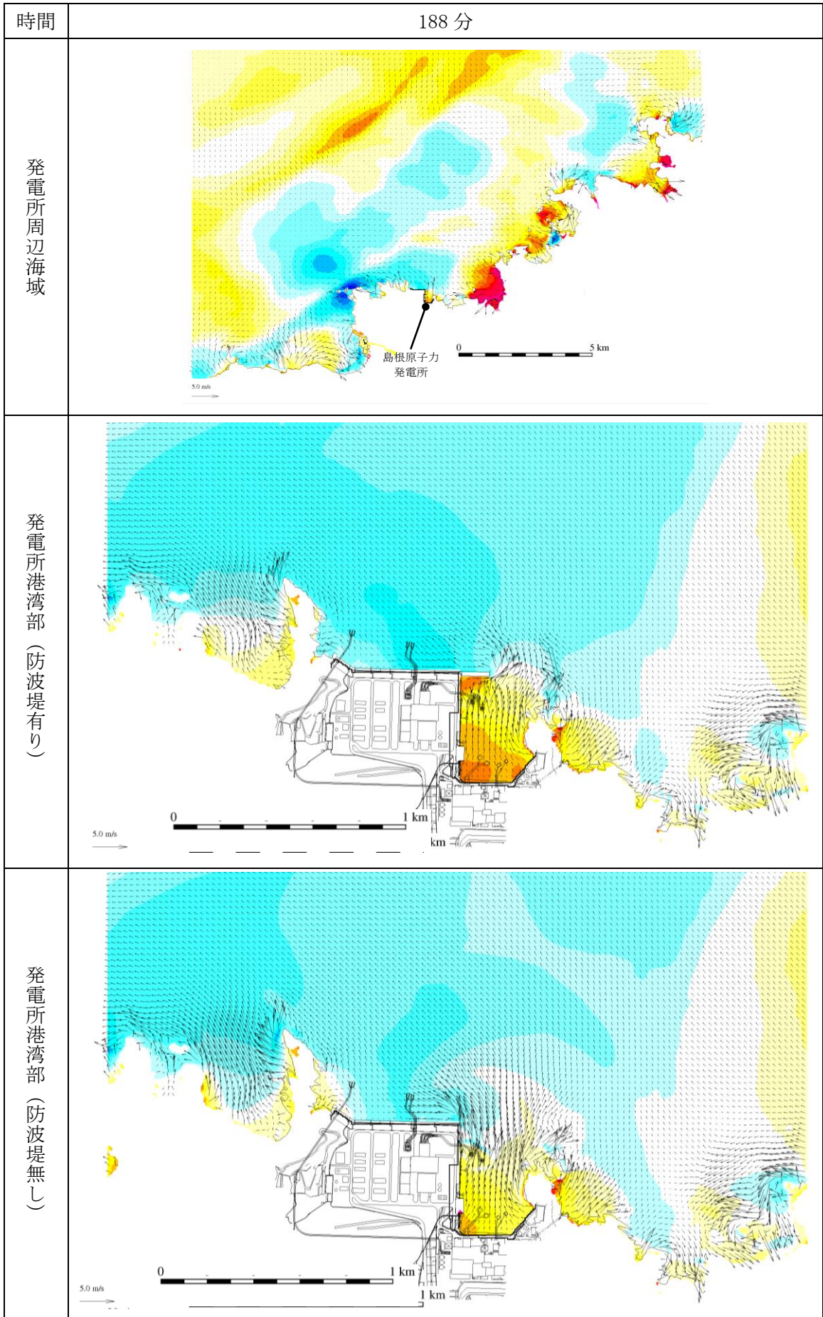
第 1 図 (177) 基準津波 1 の水位変動・流向ベクトル
