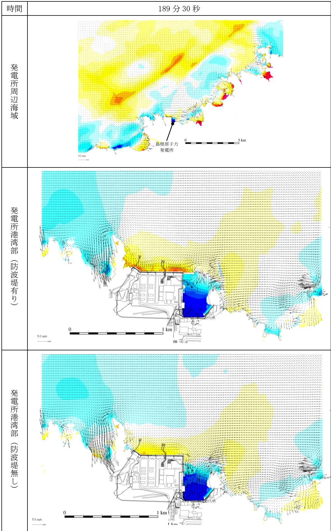
第 1 図(180) 基準津波 1 の水位変動・流向ベクトル
