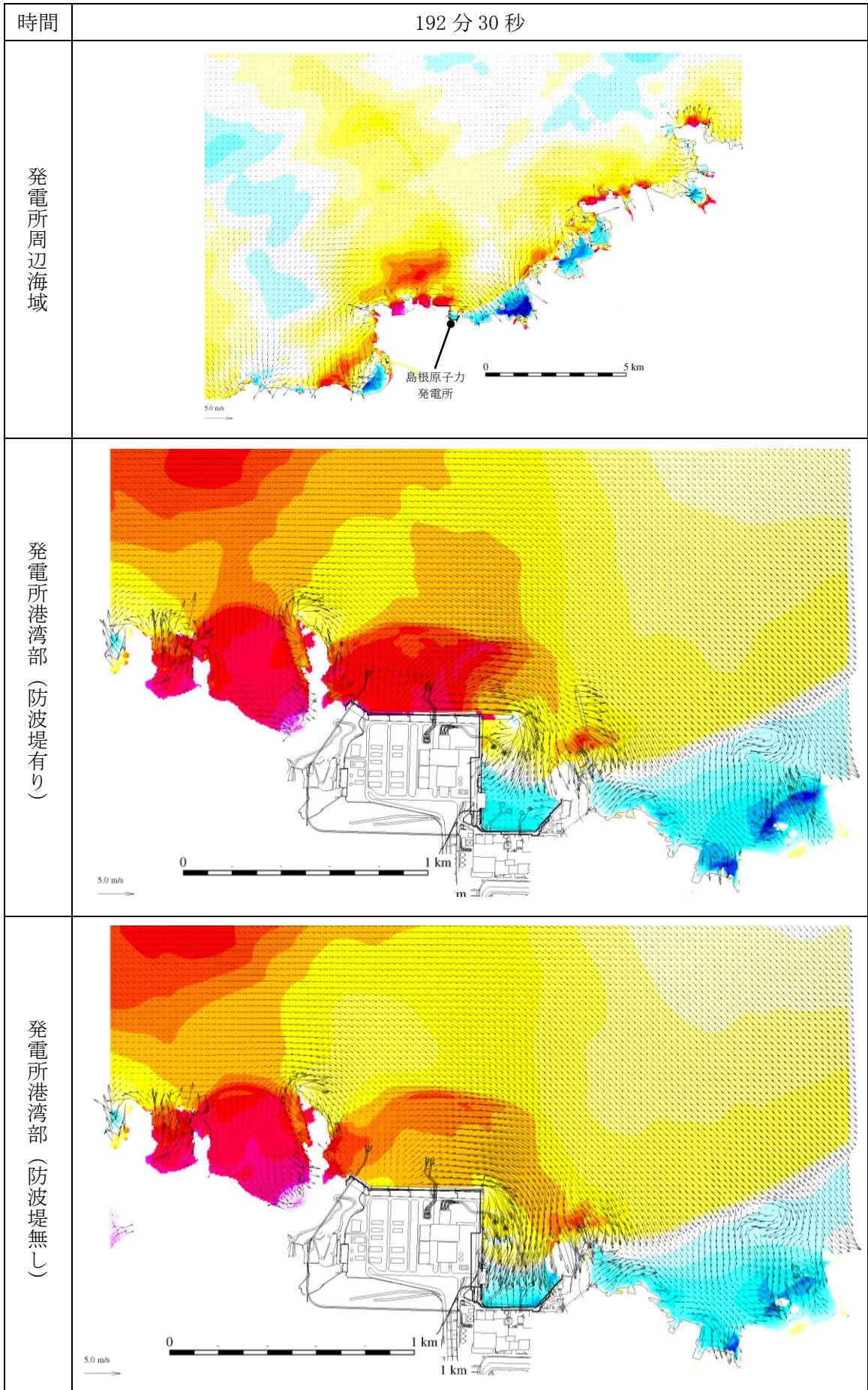
第 1 図(186) 基準津波 1 の水位変動・流向ベクトル
