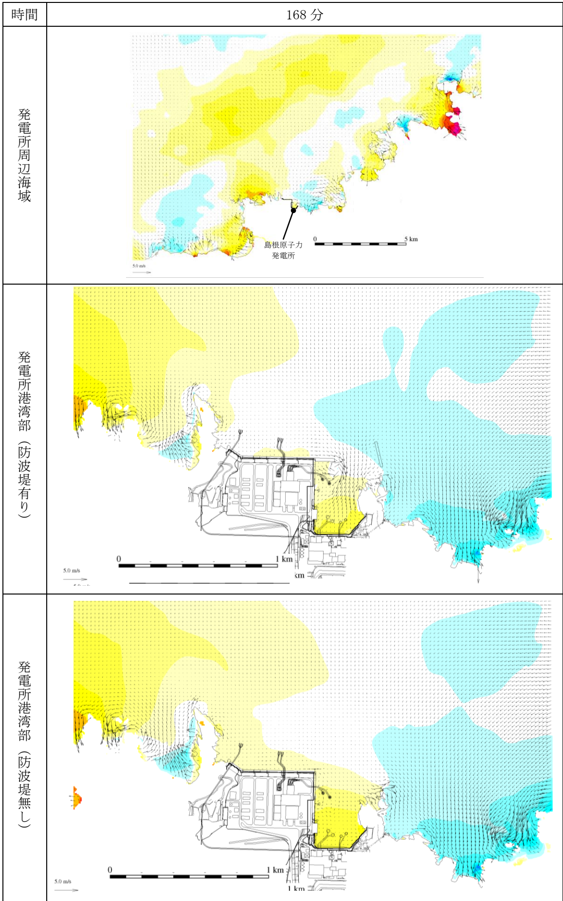
第 1 図(137) 基準津波 1 の水位変動・流向ベクトル
