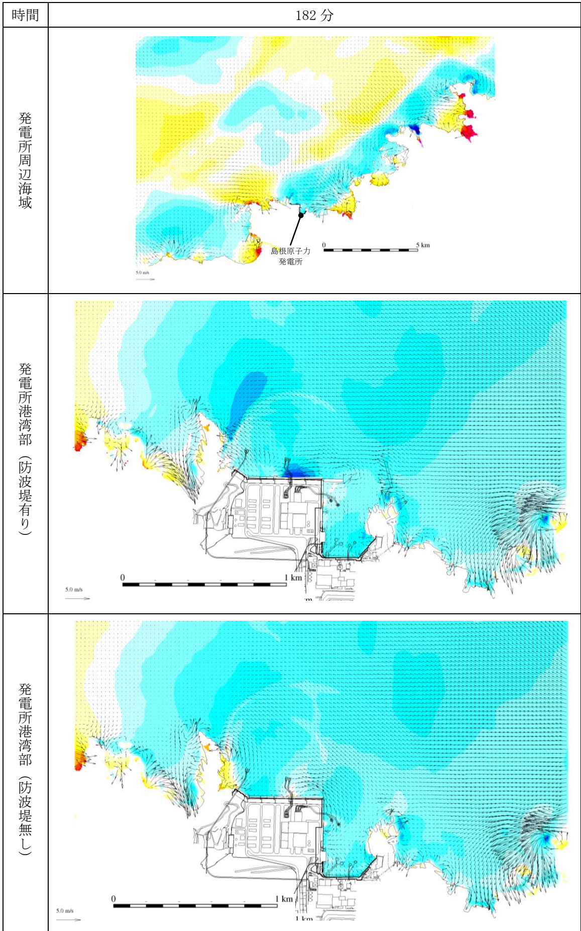
第 1 図(165) 基準津波 1 の水位変動・流向ベクトル
