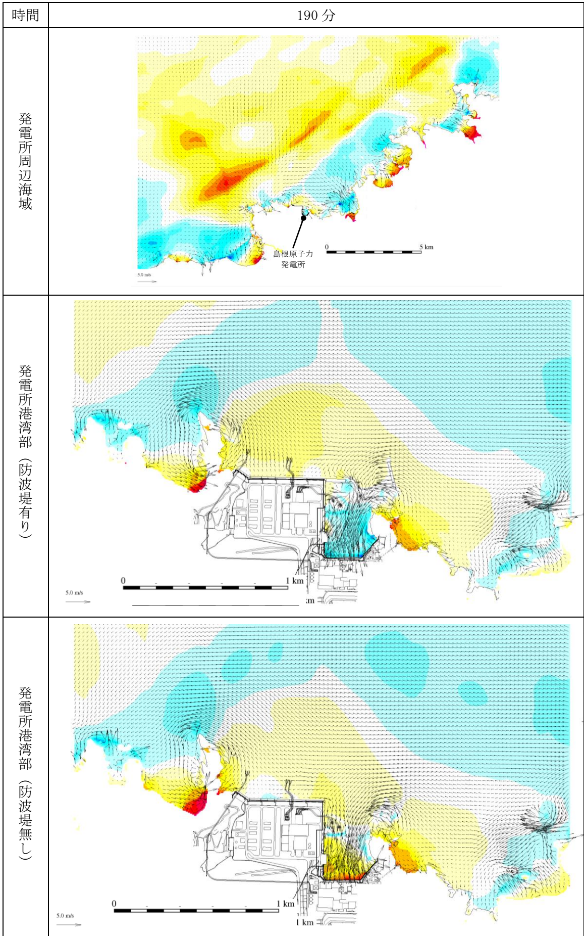
第 1 図(181) 基準津波 1 の水位変動・流向ベクトル
