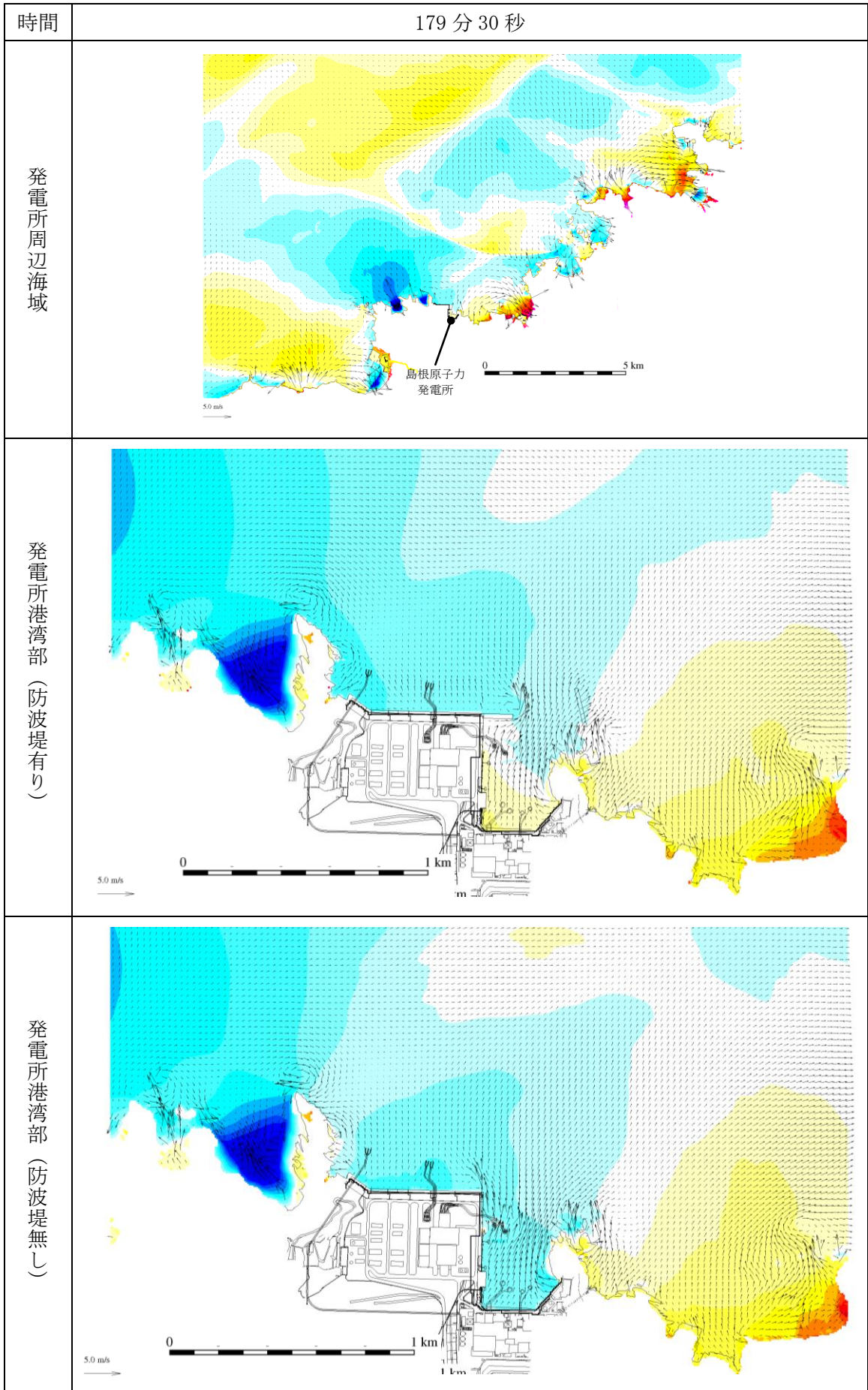
第 1 図(160) 基準津波 1 の水位変動・流向ベクトル
