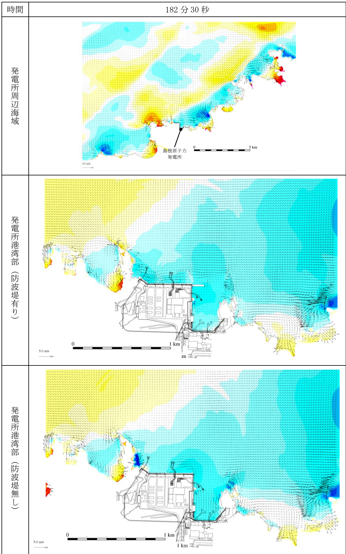
第 1 図(166) 基準津波 1 の水位変動・流向ベクトル
