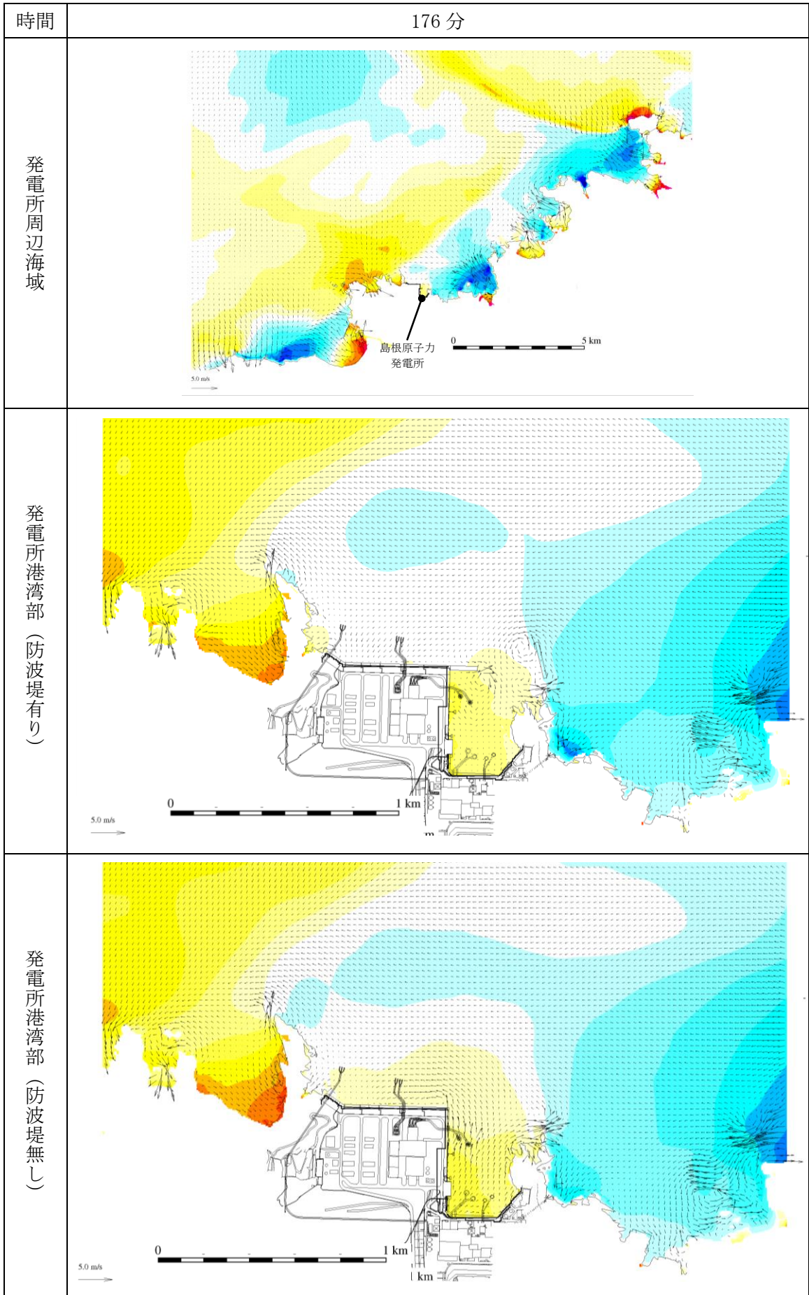
第 1 図(153) 基準津波 1 の水位変動・流向ベクトル
