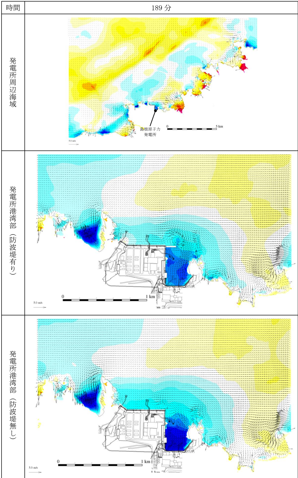
第 1 図 (179) 基準津波 1 の水位変動・流向ベクトル
