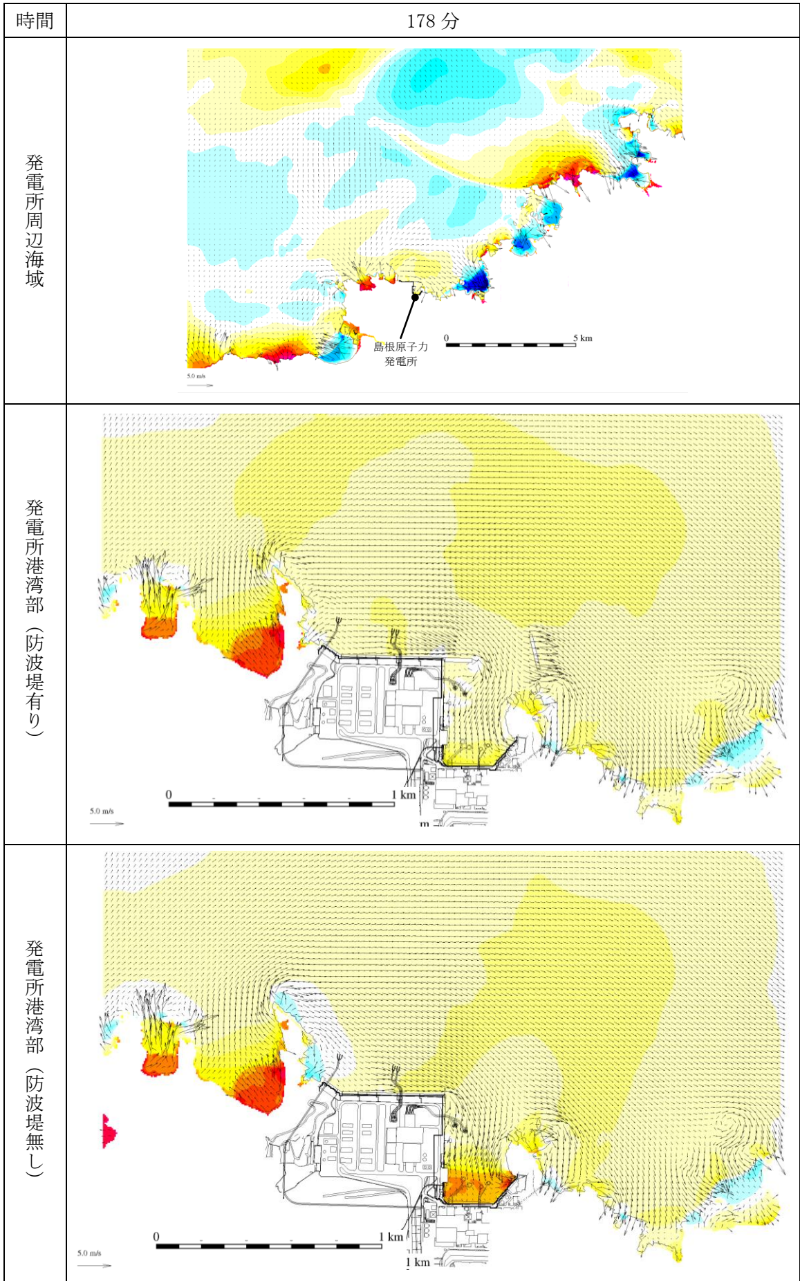
第 1 図 (157) 基準津波 1 の水位変動・流向ベクトル
