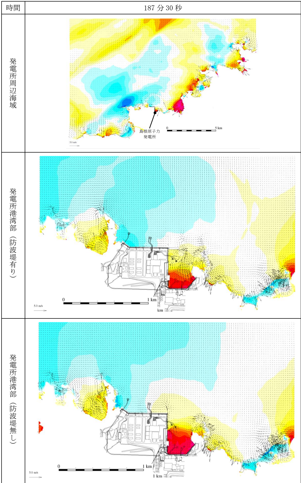
第 1 図 (176) 基準津波 1 の水位変動・流向ベクトル
