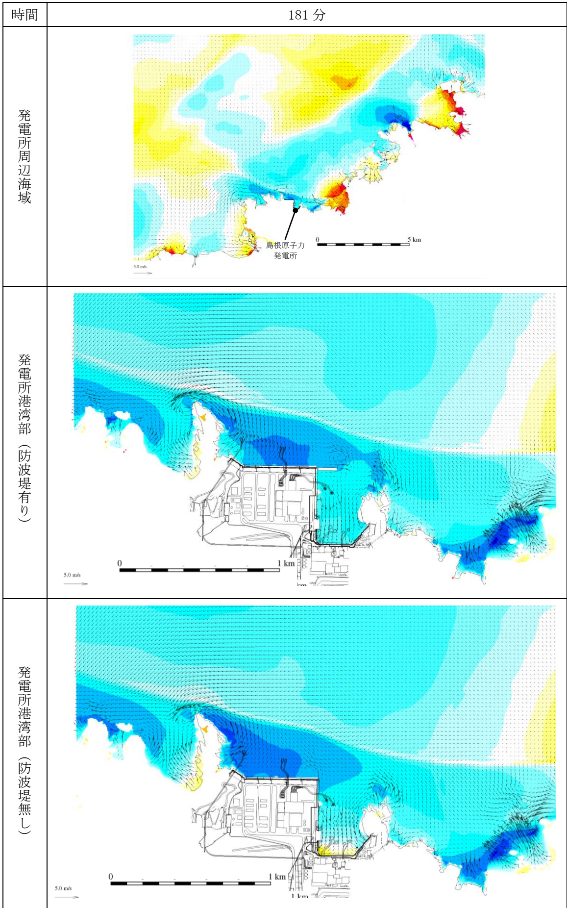
第 1 図(163) 基準津波 1 の水位変動・流向ベクトル
