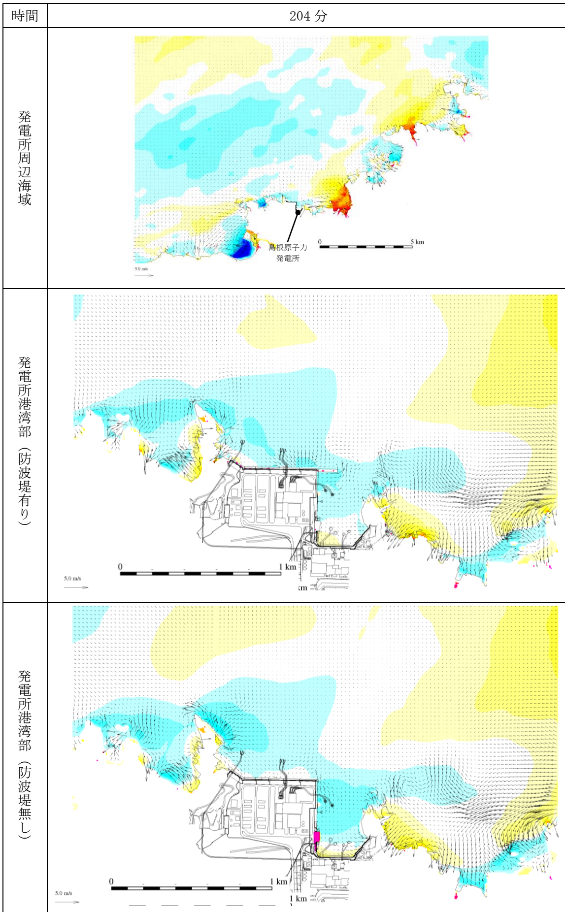
第 1 図 (209) 基準津波 1 の水位変動・流向ベクトル
