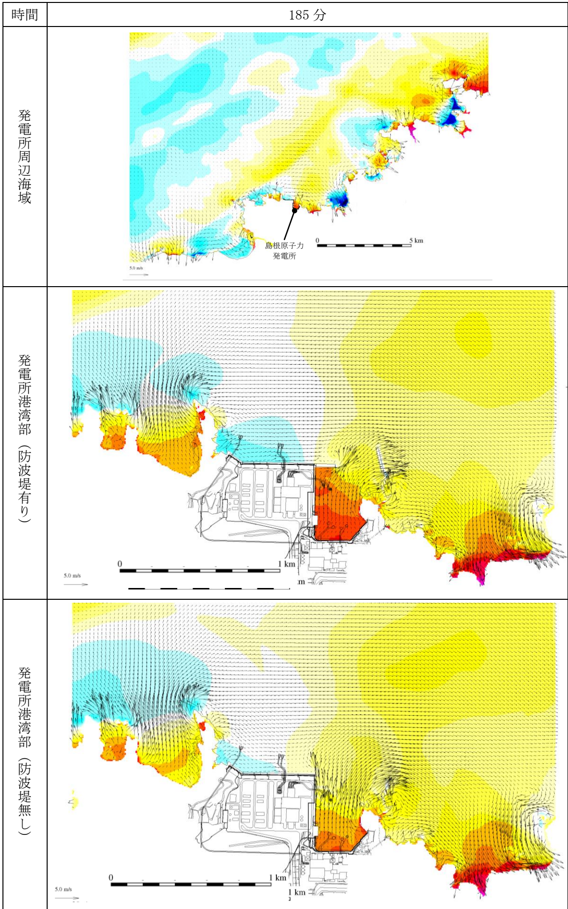
第 1 図(171) 基準津波 1 の水位変動・流向ベクトル
