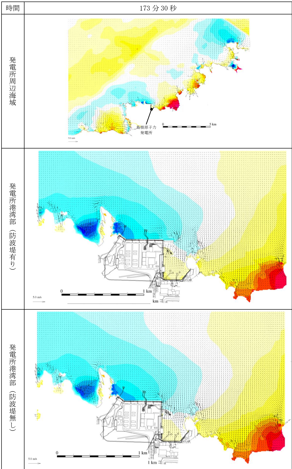
第 1 図(148) 基準津波 1 の水位変動・流向ベクトル
