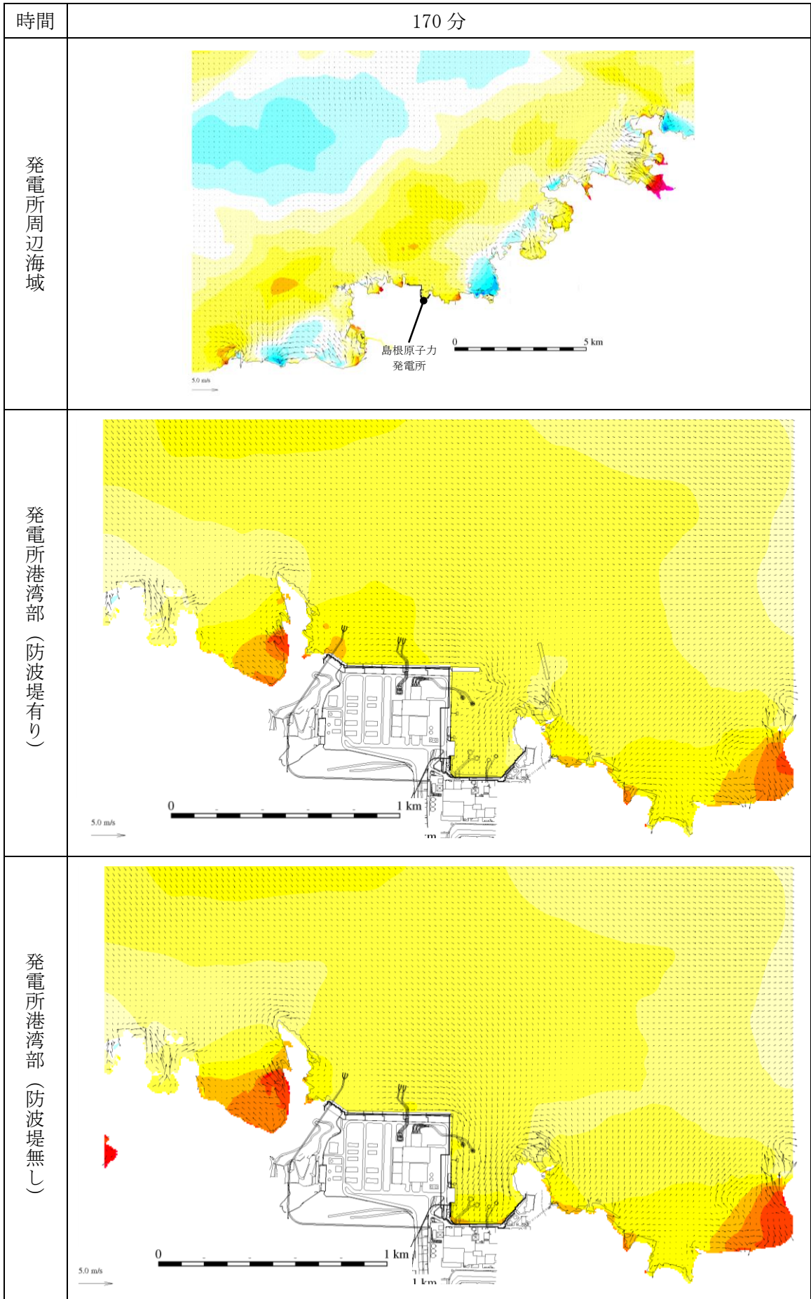
第 1 図(141) 基準津波 1 の水位変動・流向ベクトル
