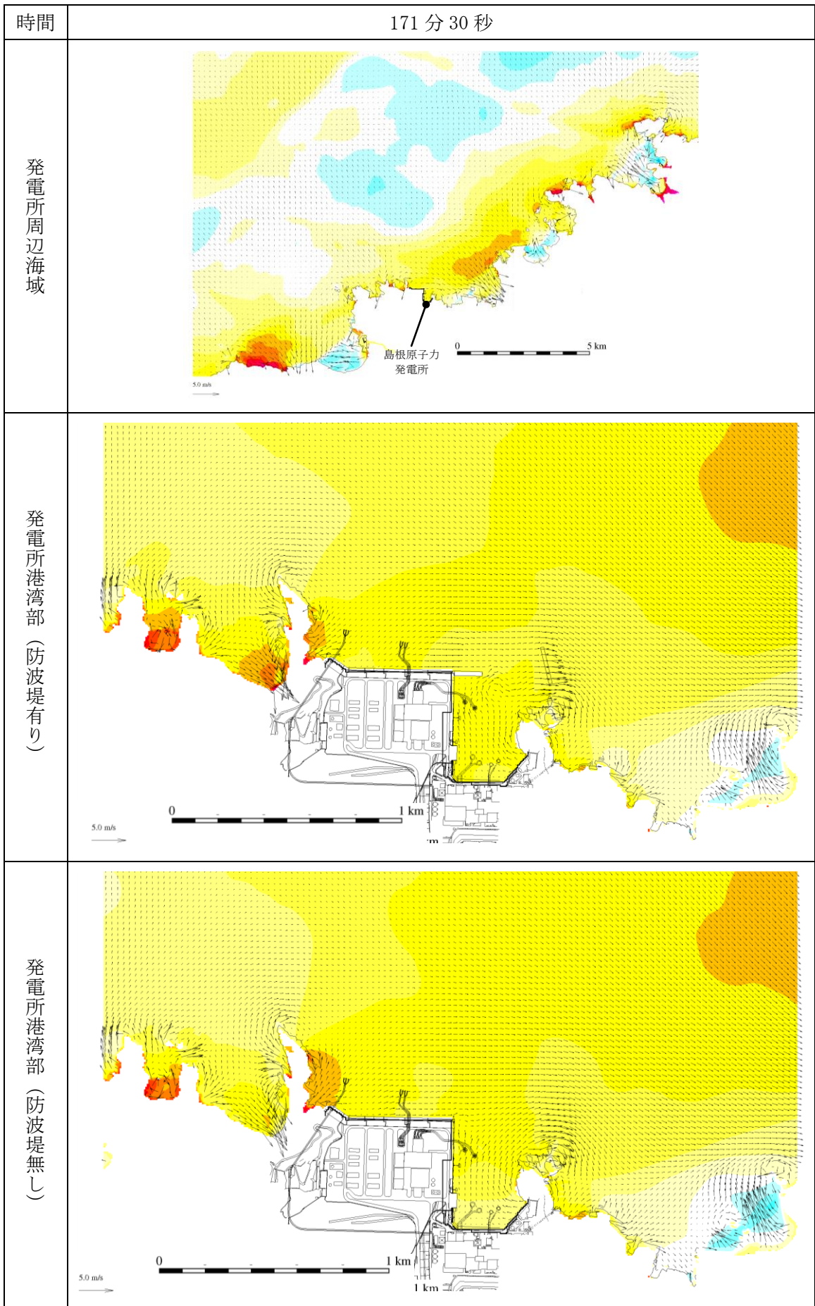
第 1 図(144) 基準津波 1 の水位変動・流向ベクトル
