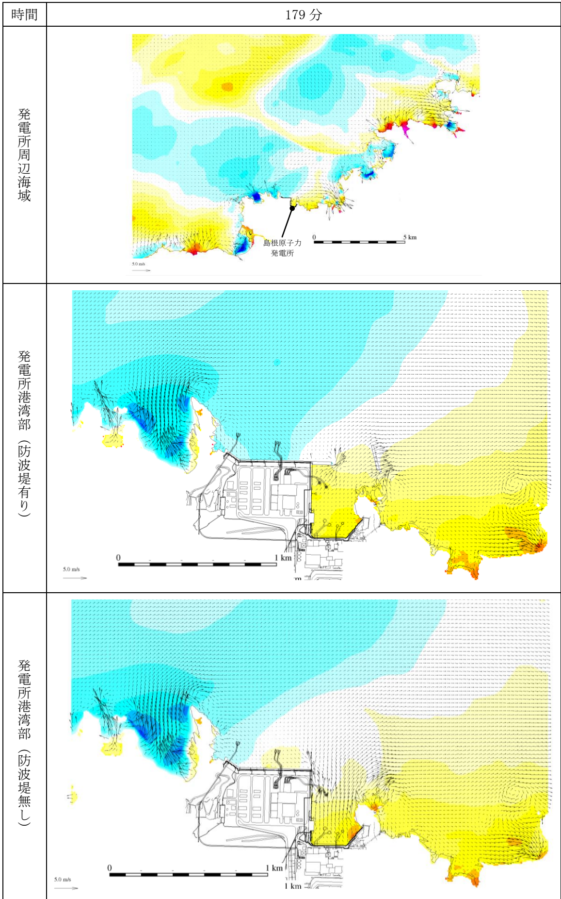
第 1 図 (159) 基準津波 1 の水位変動・流向ベクトル
