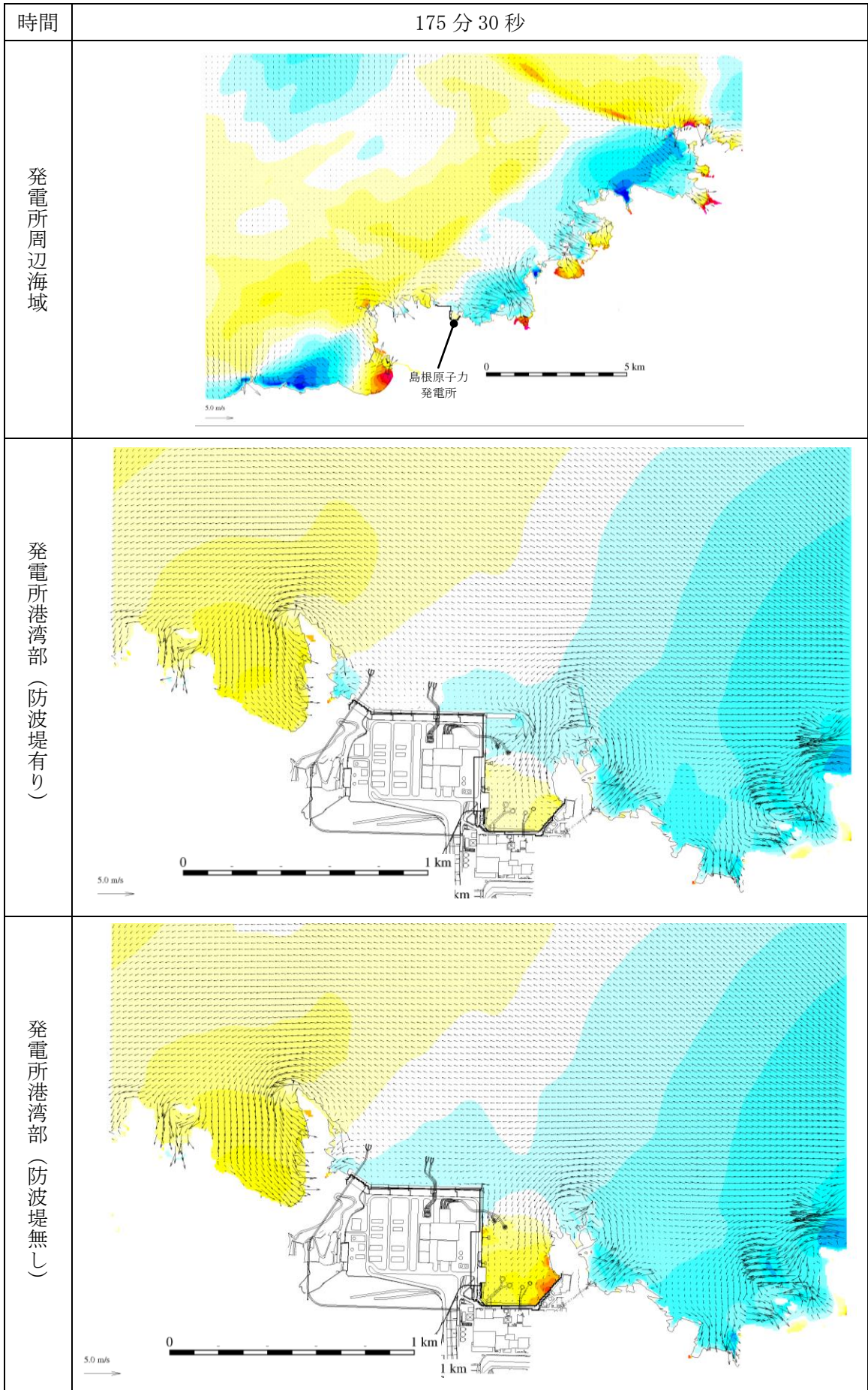
第 1 図(152) 基準津波 1 の水位変動・流向ベクトル
