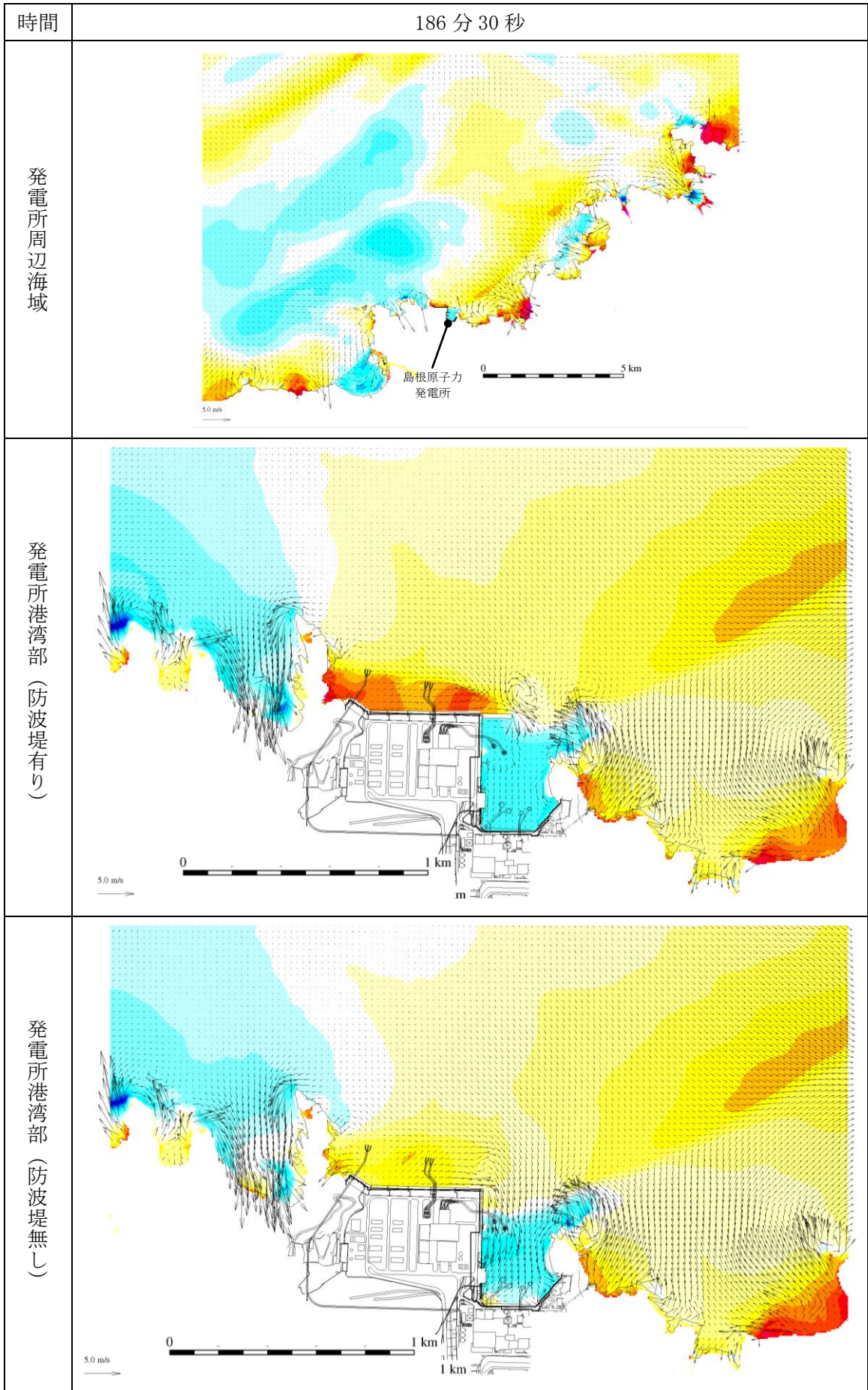
第 1 図(174) 基準津波 1 の水位変動・流向ベクトル
