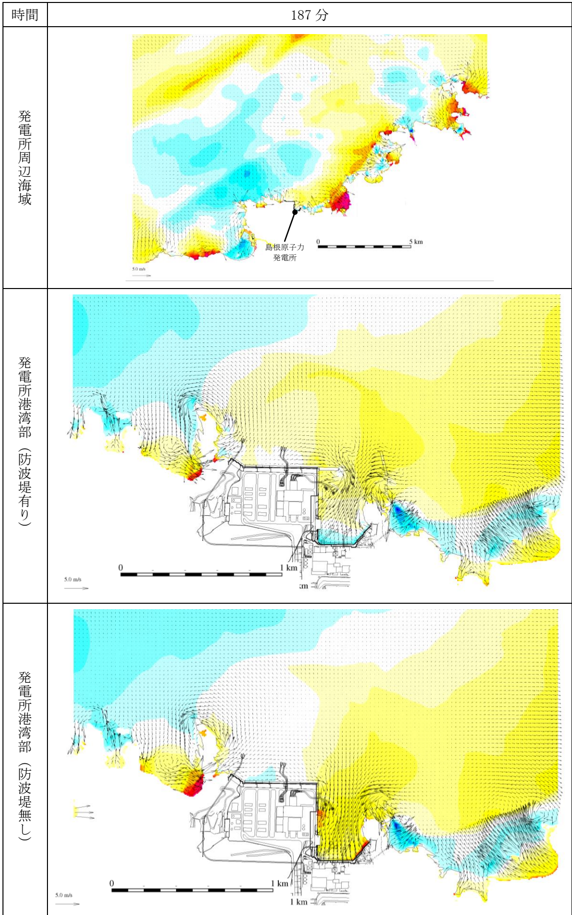
第 1 図 (175) 基準津波 1 の水位変動・流向ベクトル
