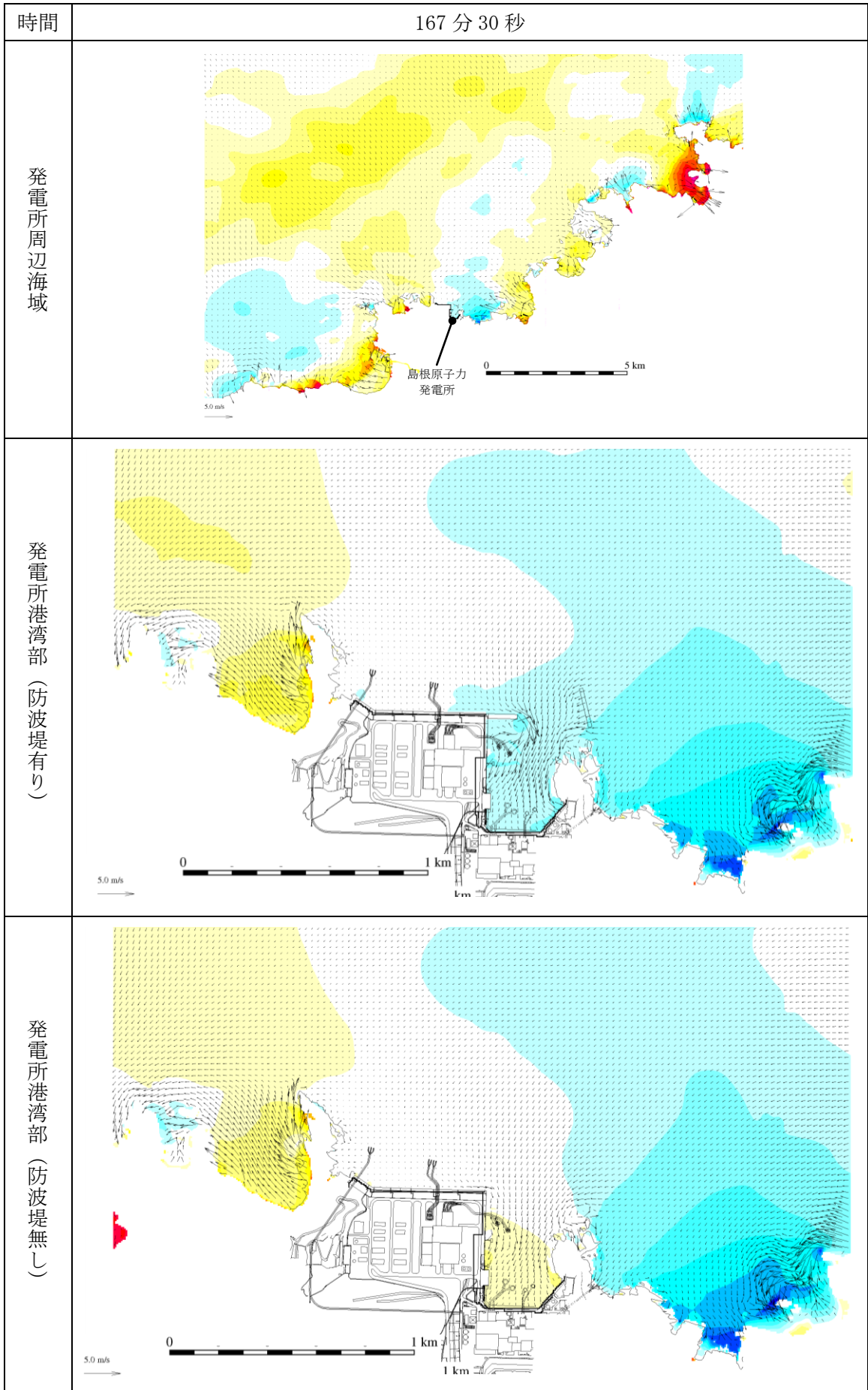
第 1 図(136) 基準津波 1 の水位変動・流向ベクトル
