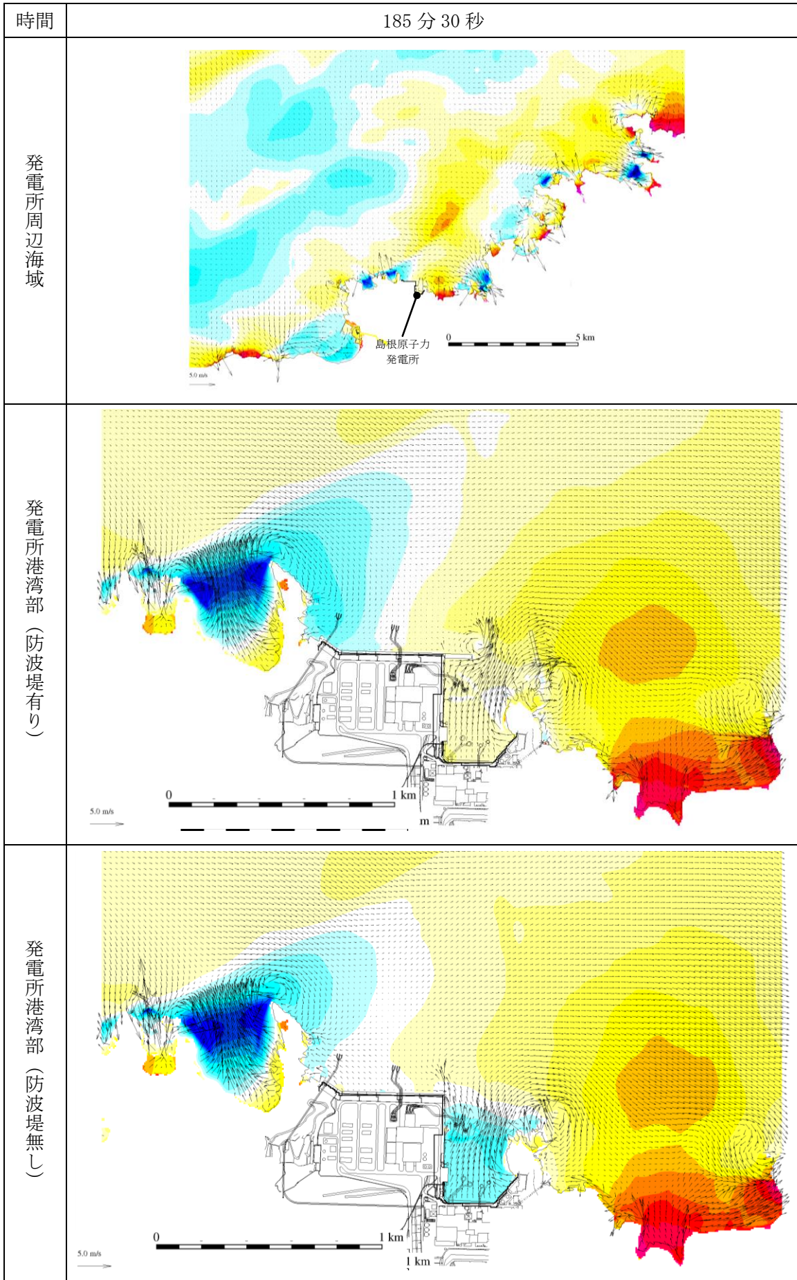
第 1 図 (172) 基準津波 1 の水位変動・流向ベクトル
