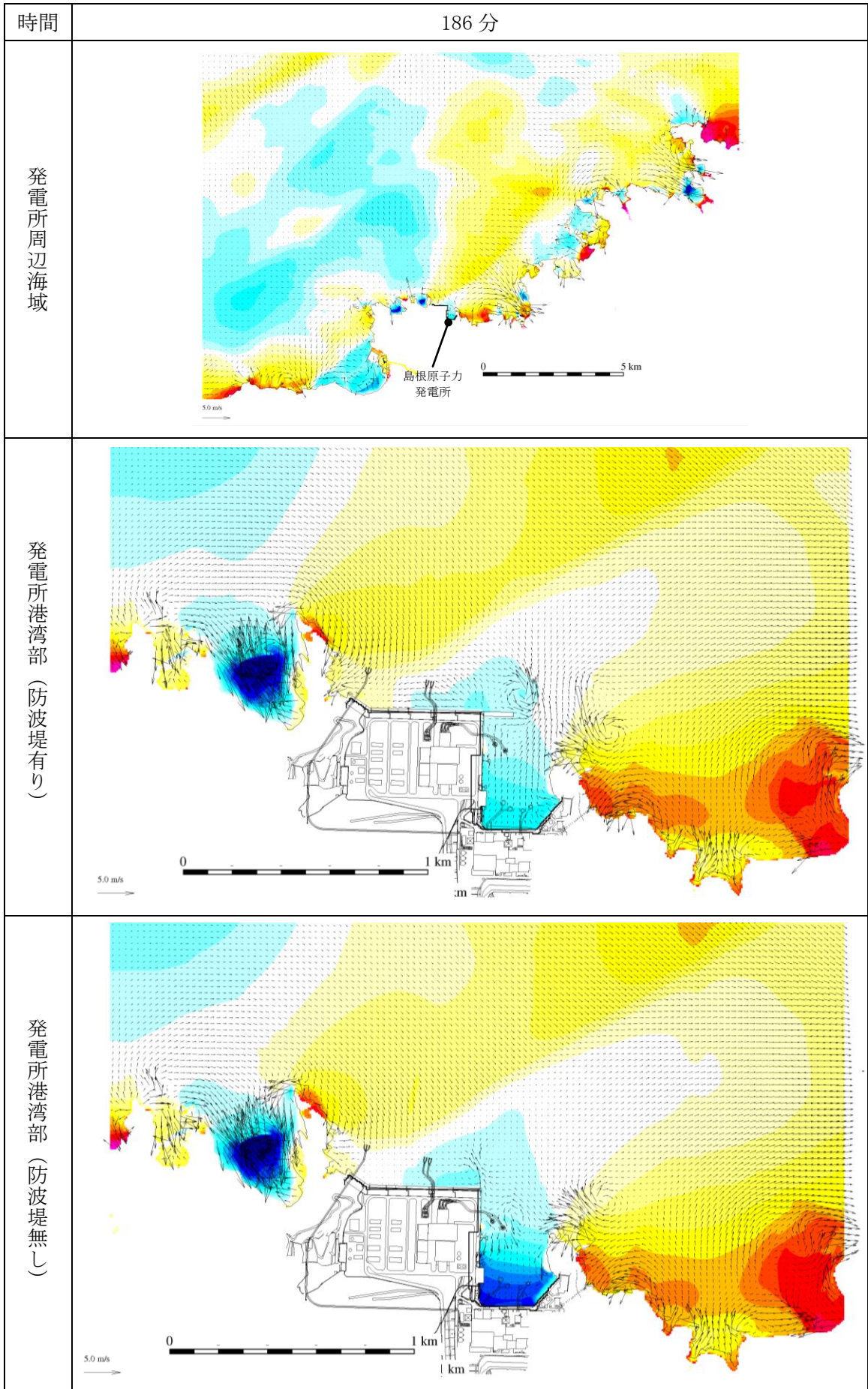
第 1 図 (173) 基準津波 1 の水位変動・流向ベクトル
