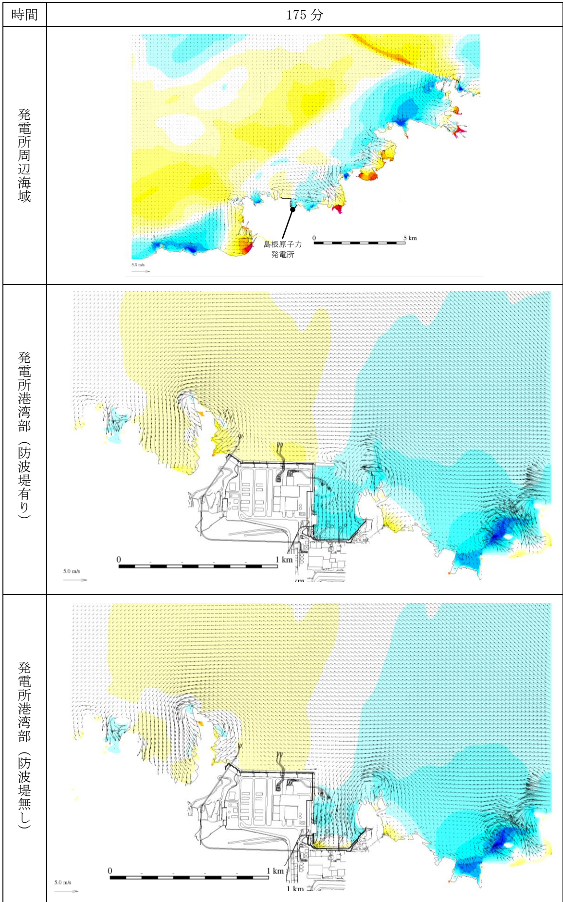
第 1 図 (151) 基準津波 1 の水位変動・流向ベクトル
