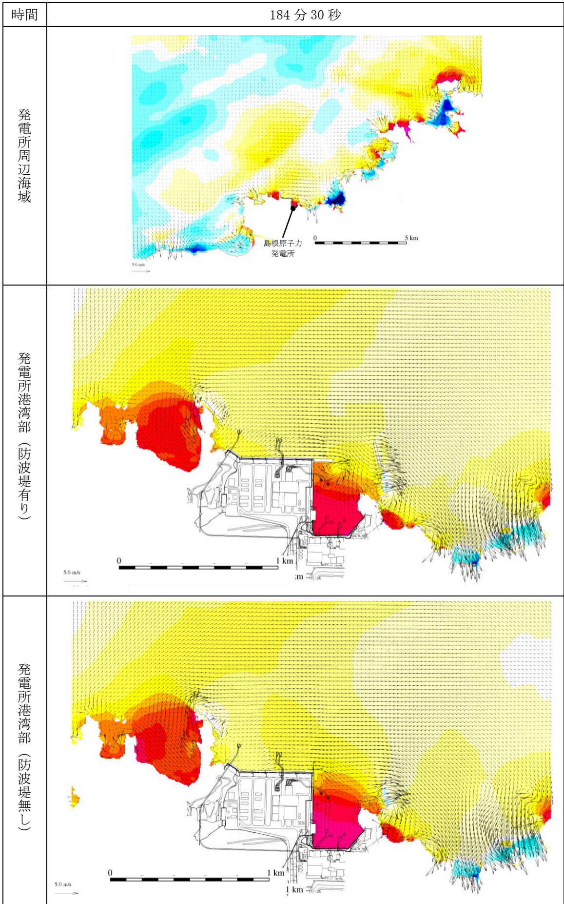
第 1 図 (170) 基準津波 1 の水位変動・流向ベクトル
