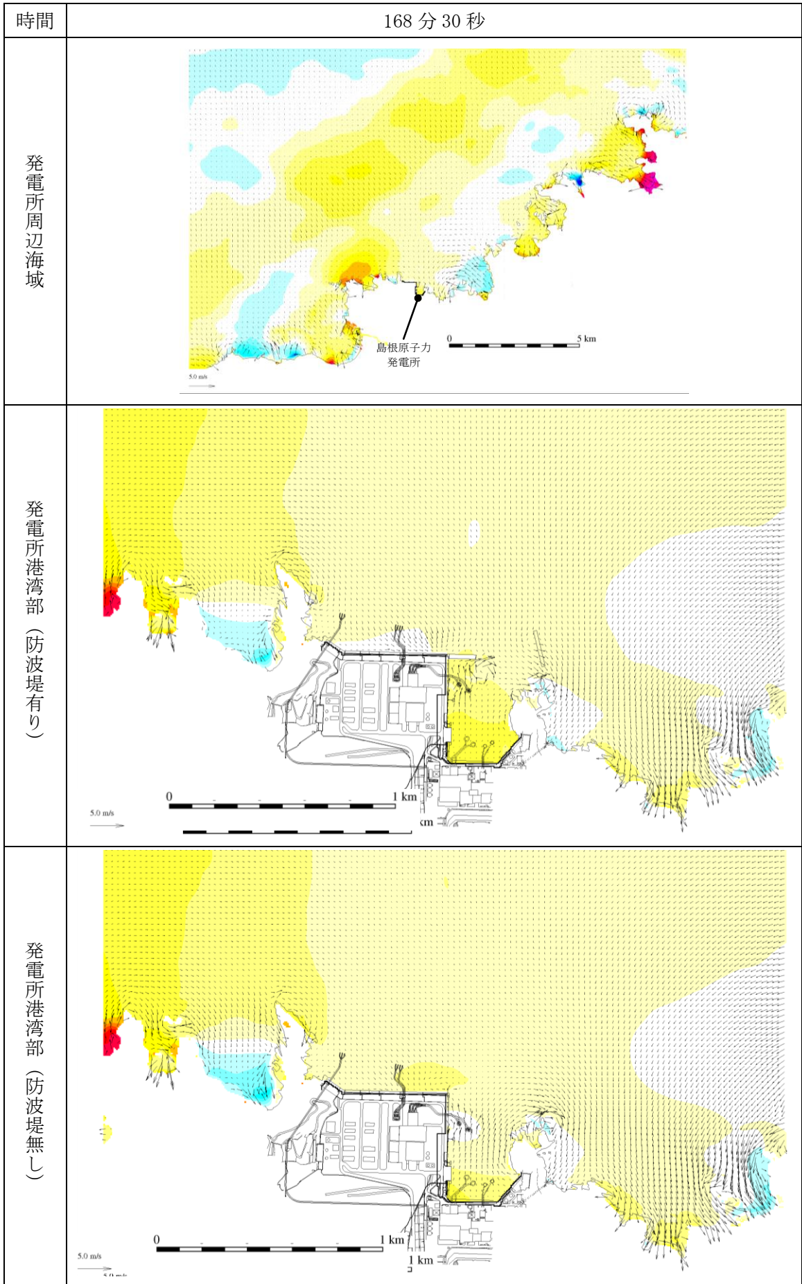
第 1 図 (138) 基準津波 1 の水位変動・流向ベクトル
