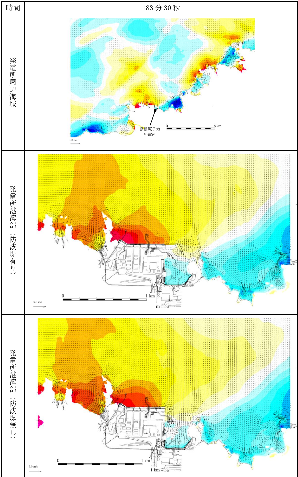
第 1 図(168) 基準津波 1 の水位変動・流向ベクトル
