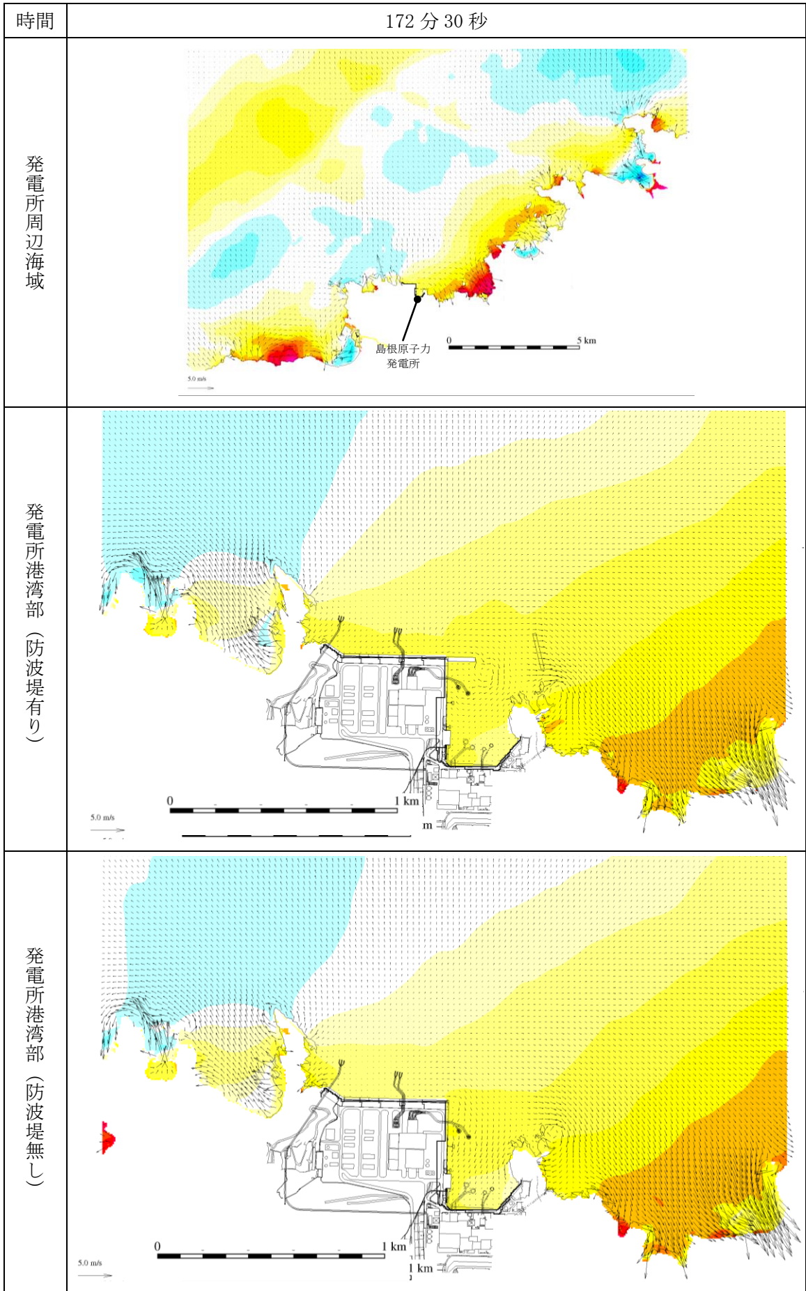
第 1 図(146) 基準津波 1 の水位変動・流向ベクトル
