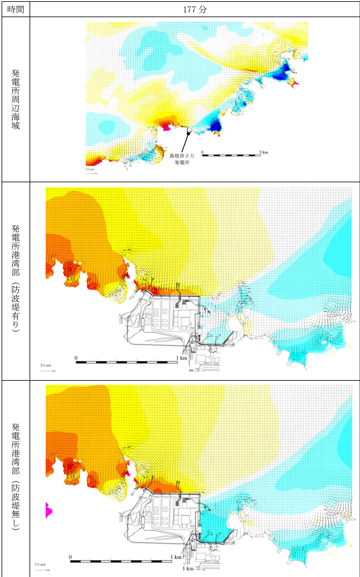
第 1 図(155) 基準津波 1 の水位変動・流向ベクトル
