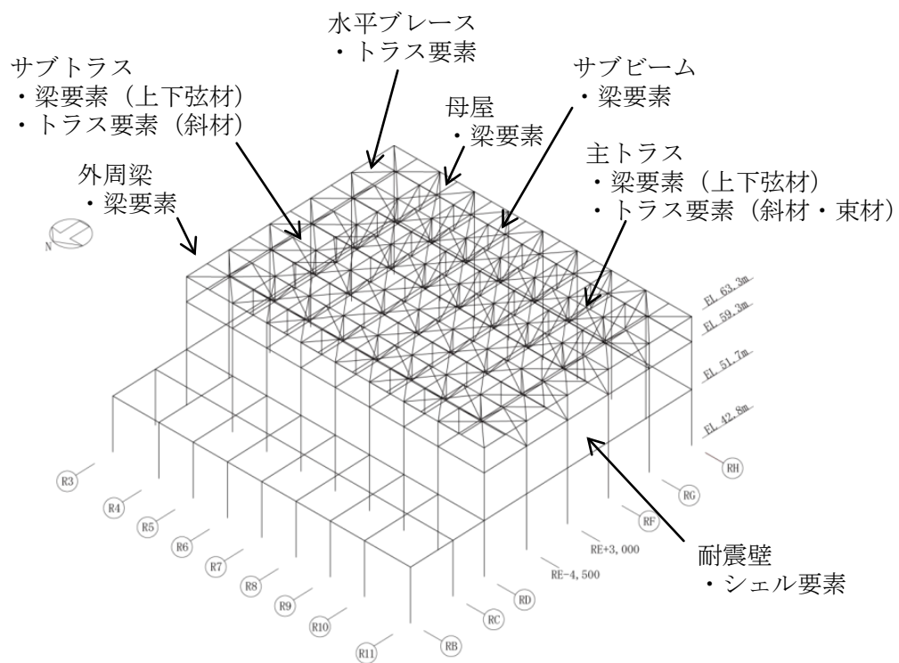
第 1-5 図 原子炉建物主トラスの応力解析に用いる三次元立体モデル (概念図)
