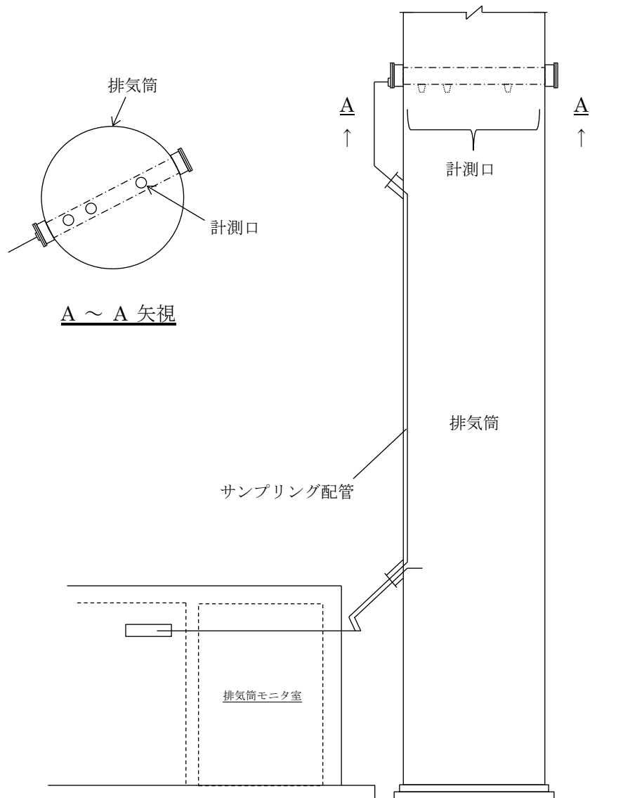
第 10-1 図 排気筒モニタサンプリング配管概要図
