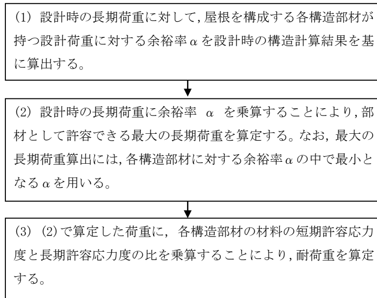
第 1-3 図 耐荷重算定フロー
