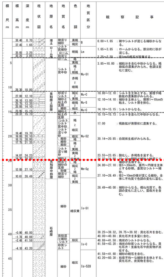
敷地内ボーリング柱状図 (No.114)
