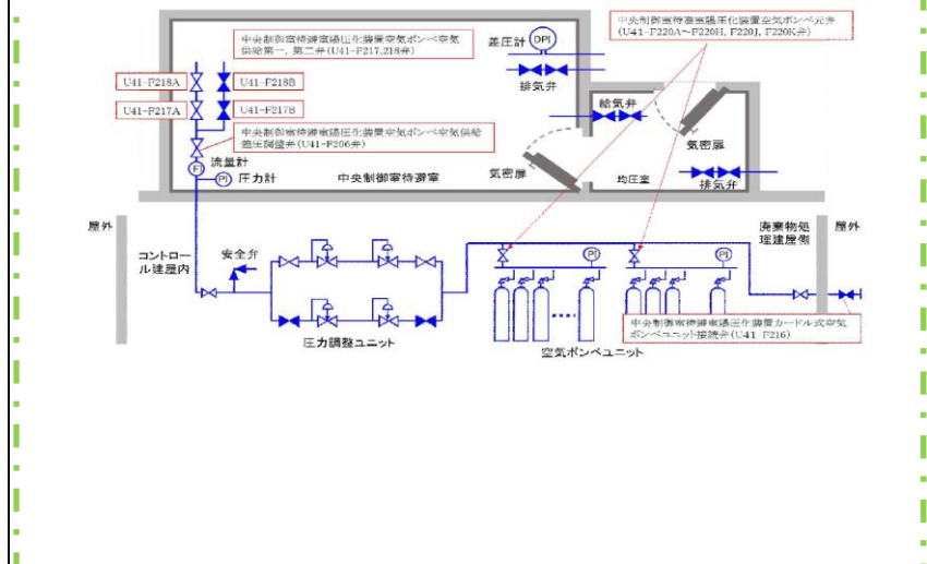
図 2.4-16 陽圧化装置 系統概要図
