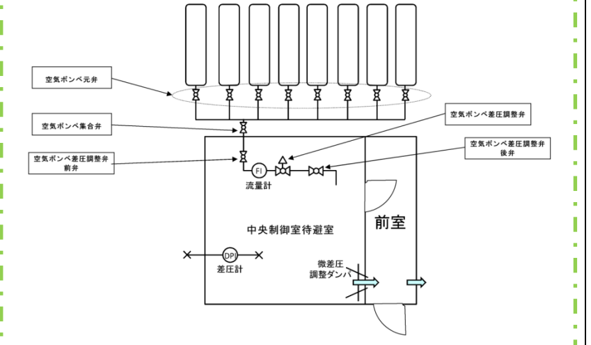
第 2.4-6 図 中央制御室待避室空気ポンベユニット 概要図
