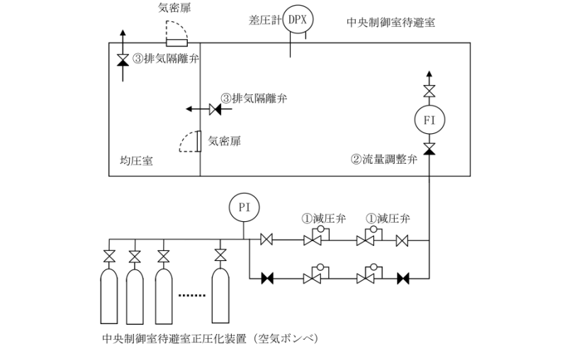
図 2.4-16 中央制御室待避室正圧化装置 系統概要図
