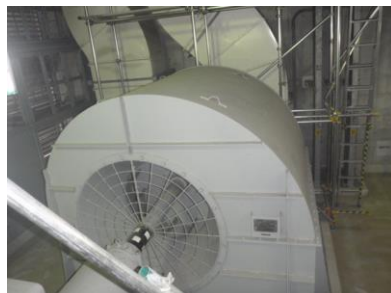
B-ディーゼル室送風機 及びケーブルトレイ
