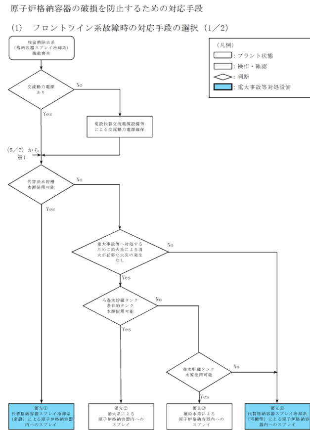
第 1.6-29 図 重大事故等時の対応手段選択フローチャート (3/5)
