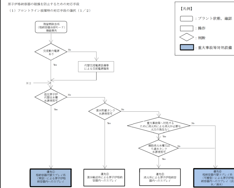
原子炉格納容器の破損を防止するための対応手段 (1) フロントライン故障時の対応手段の選択 (2/2)
