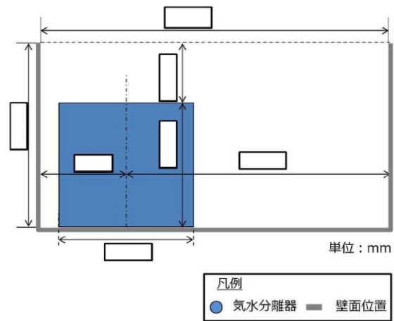
図添 1-12-8 DSP 断面図 (A-A'断面)
