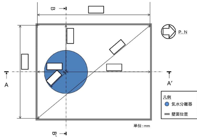
図添 1-12-7 DSP 平面図
