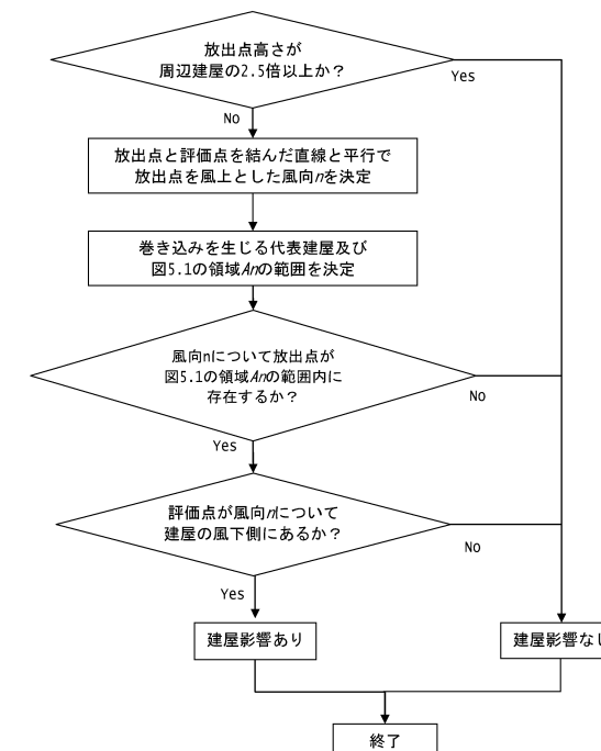
図 5.2 建屋影響の有無の判断手順
