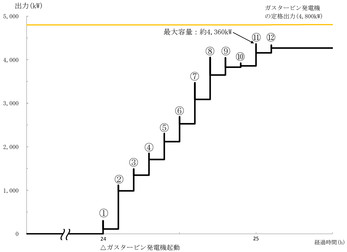
第 57-9-3 図 ガスタービン発電機負荷積上_全交流動力電源喪失 (長期 T B)
