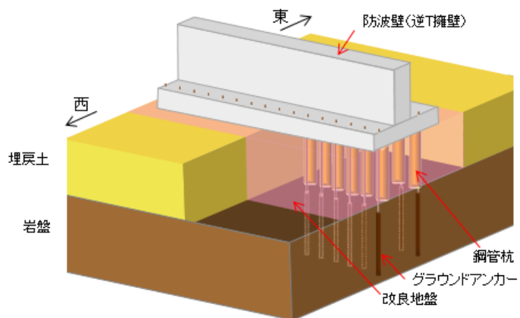
第10.6-4図 防波壁 (逆T擁壁) 概念図
