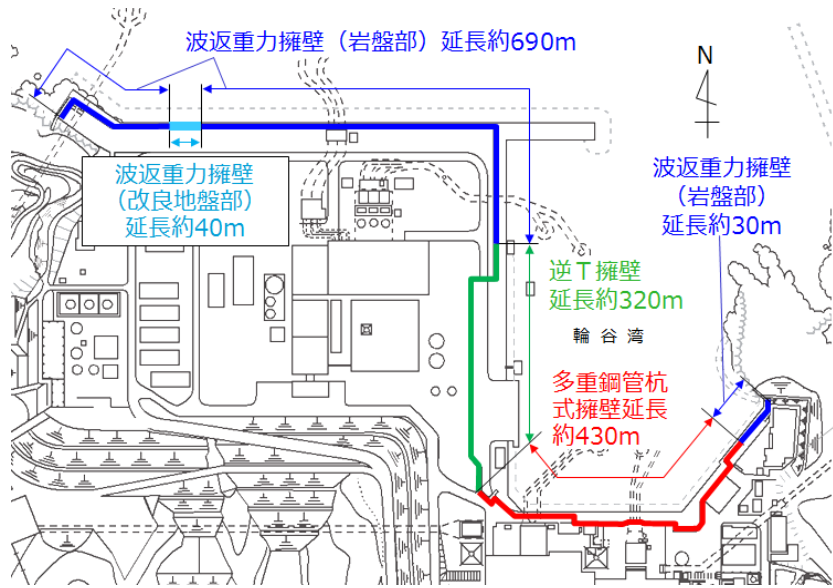
第10.6-2図 防波壁配置図
