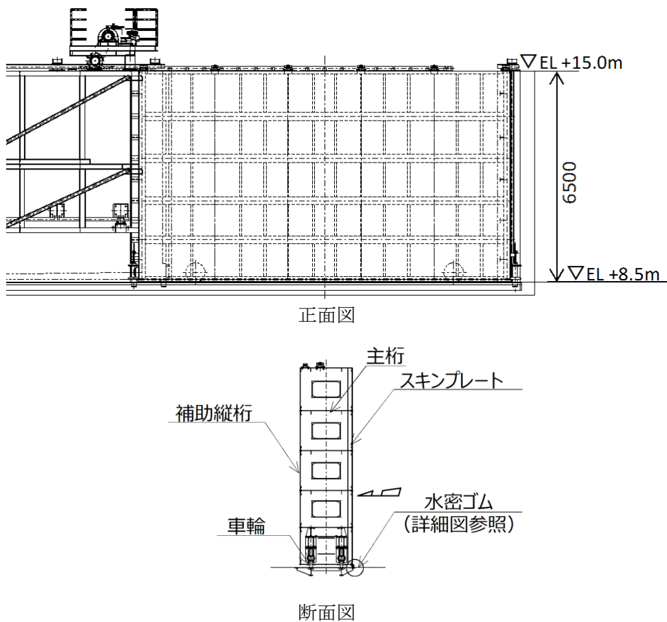
第10.6-6図 防波壁通路防波扉（3号炉東側）概念図
