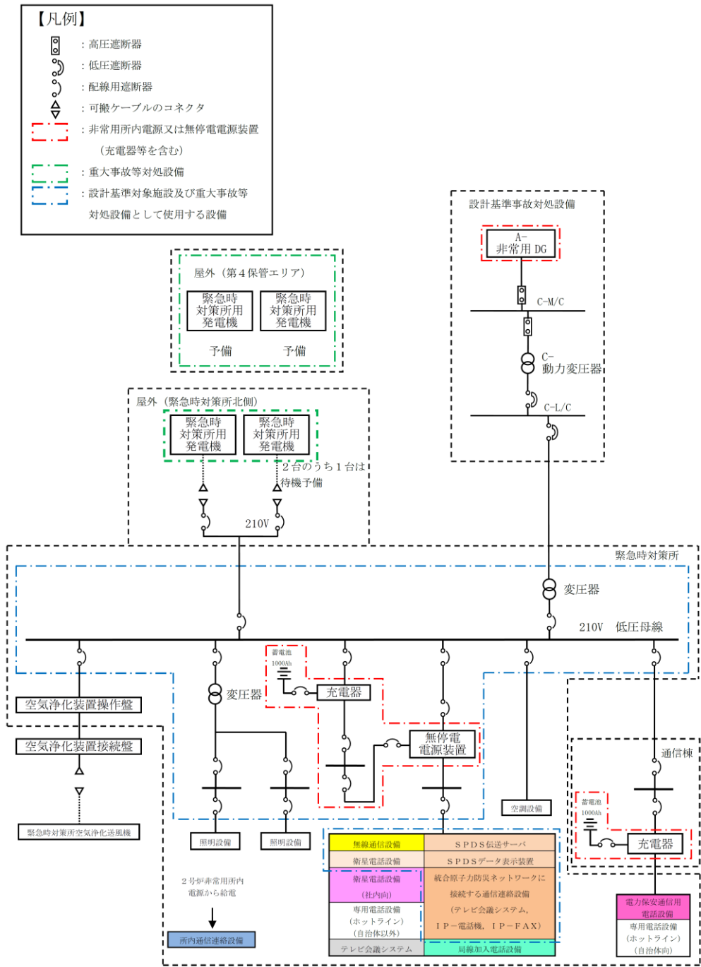
第62-2-2図 緊急時対策所における通信連絡設備の単線結線図
