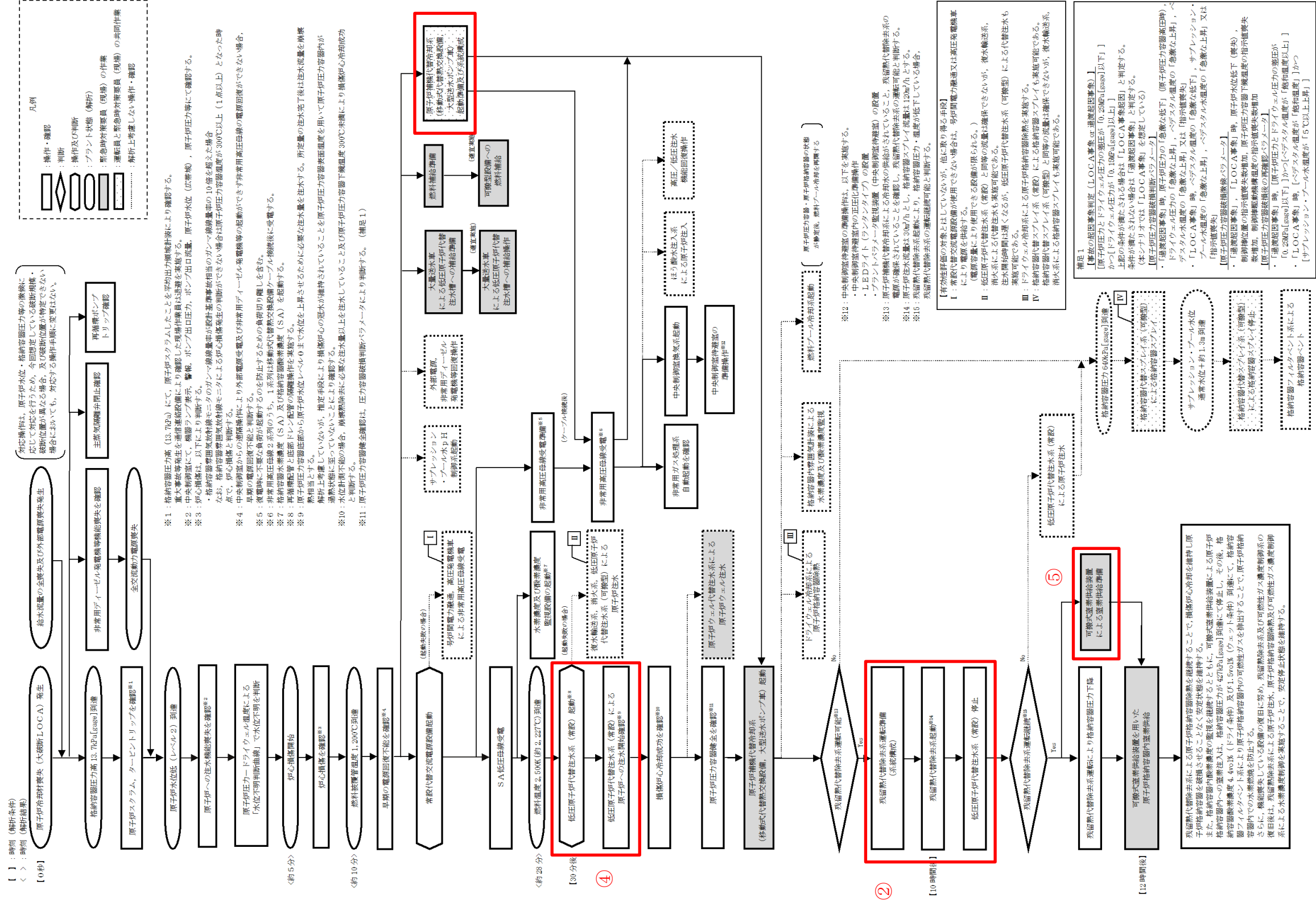
第 3.1.2.1-2 図 「雰囲気圧力・温度による静的負荷（格納容器過圧・過温破損）」の対応手順の概要 (残留熱代替除去系を使用する場合)
