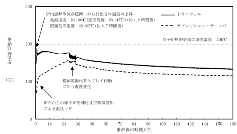
第 3. 1. 3. 3-1(3) 図 操作開始時間 30 分遅れのケースにおける格納容器温度の推移
