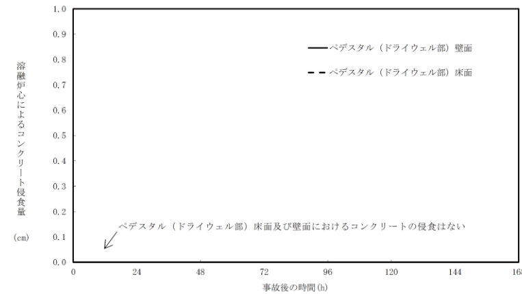
第3図 ペDESTAL (ドライウェル部) 床面及び壁面のコンクリート侵食量の推移
