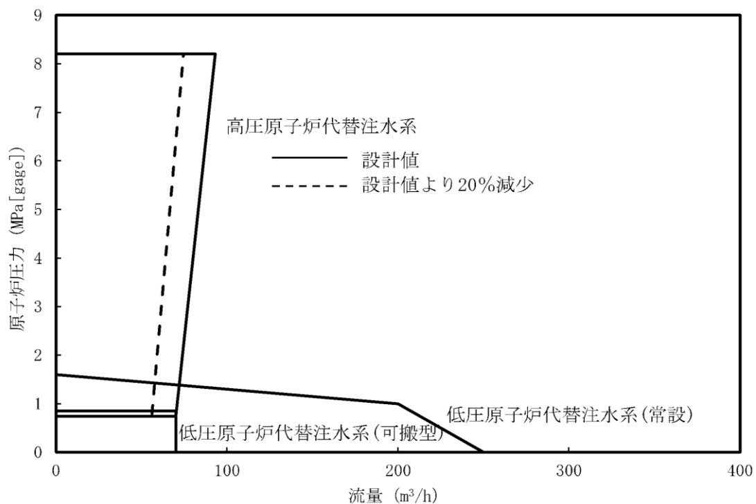
図1 注水特性図
