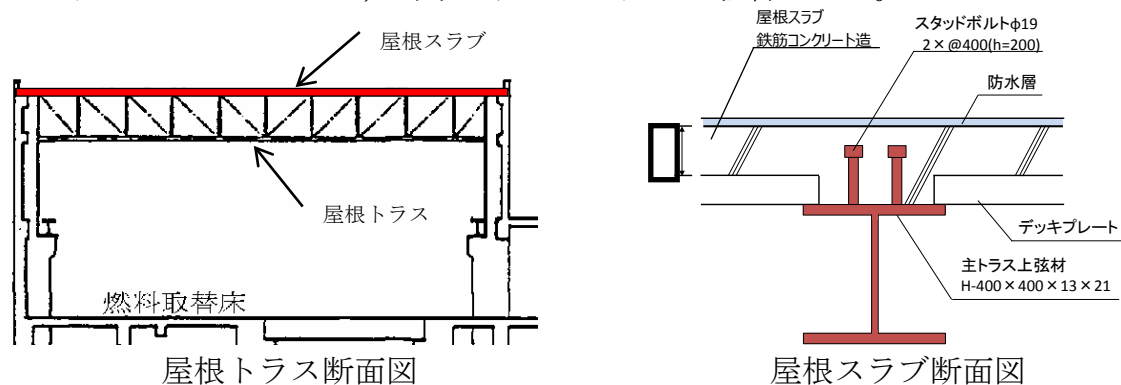
第 1-1 図 原子炉建物屋根スラブの概要
