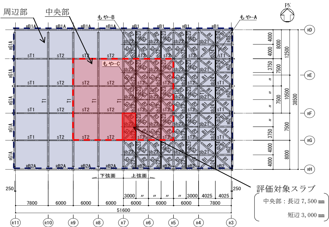
第 1-2 図 原子炉建物屋根スラブ評価位置図
