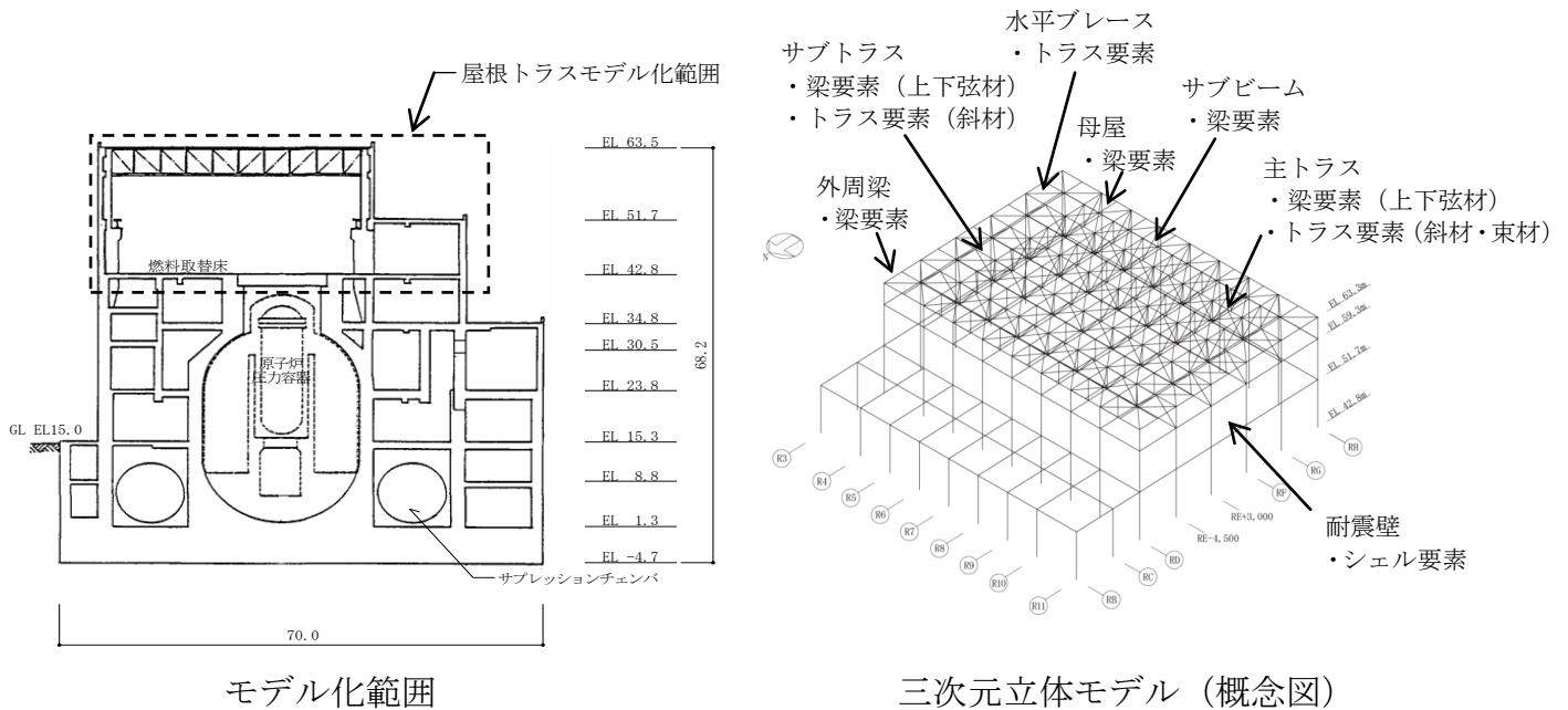
第 1-5 図 原子炉建物主トラスの応力解析に用いる三次元立体モデル (概念図)
