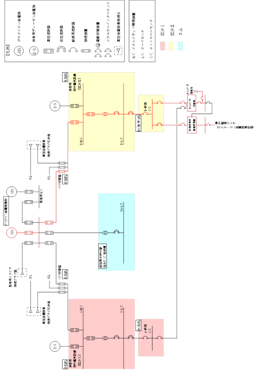
図1 単線結線図
