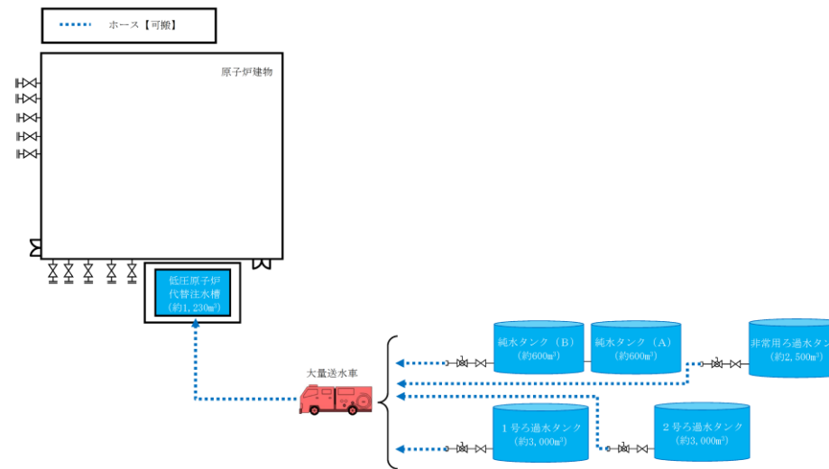
図 1 淡水タンク（ろ過タンク及び純水タンク）から低圧原子炉代替注水槽への供給
