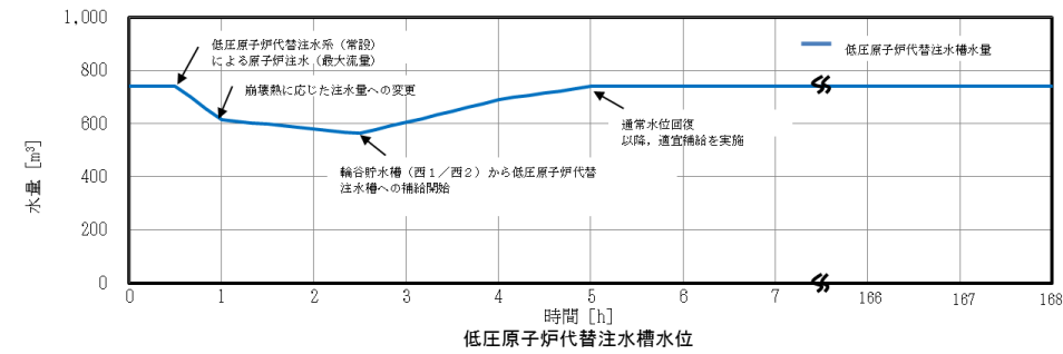
図 1 低圧原子炉代替注水槽の水量変化
