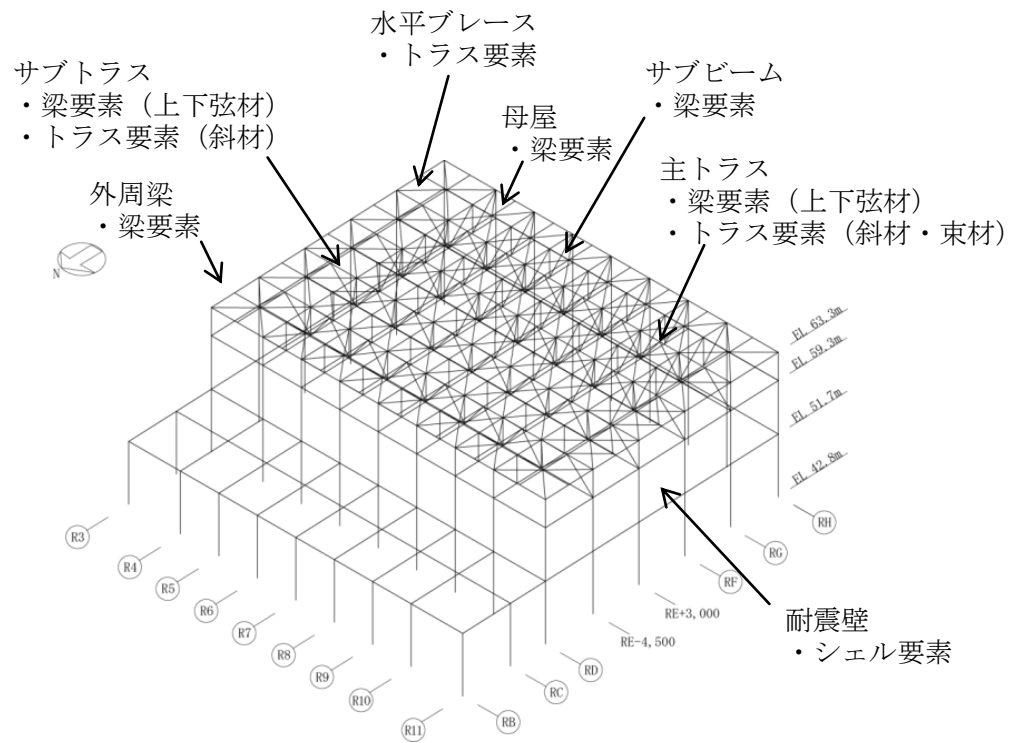
第 1-3 図 原子炉建物主トラスの応力解析に用いる三次元立体モデル（概念図）
