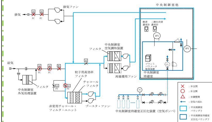
図2.4-5 中央制御室換気系及び中央制御室待避室正圧化装置系統概要図（1/2）（炉心の著しい損傷の発生時、プルーム通過前及びプルーム通過後）
