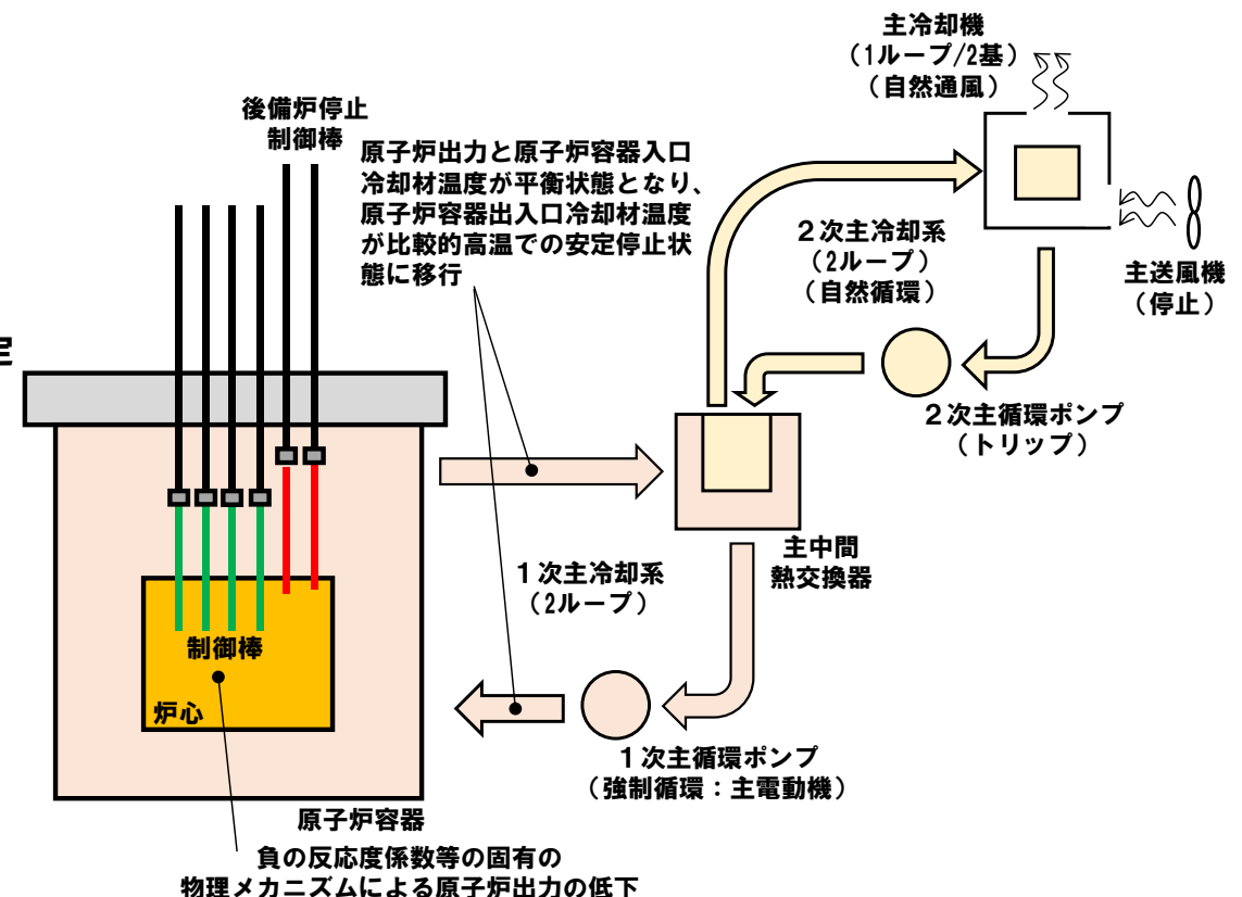
事象進展 (i) (ii) 及び格納容器破損防止措置の概念図
