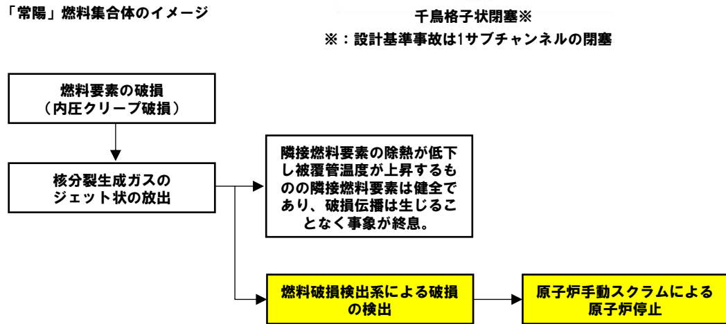
事象進展及び炉心損傷防止措置の概念図
